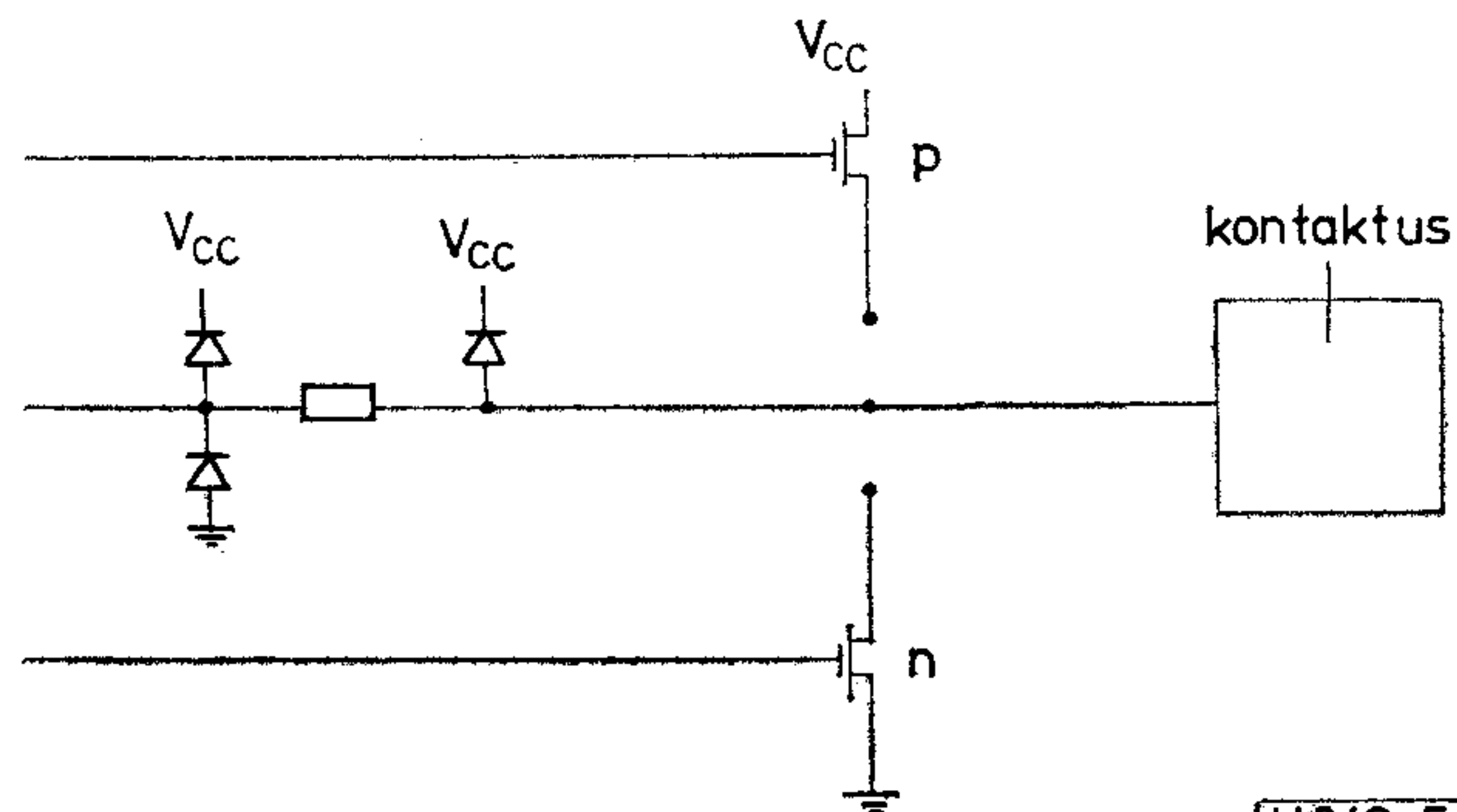
5. ábra. CMOS ULA I/O cellája
