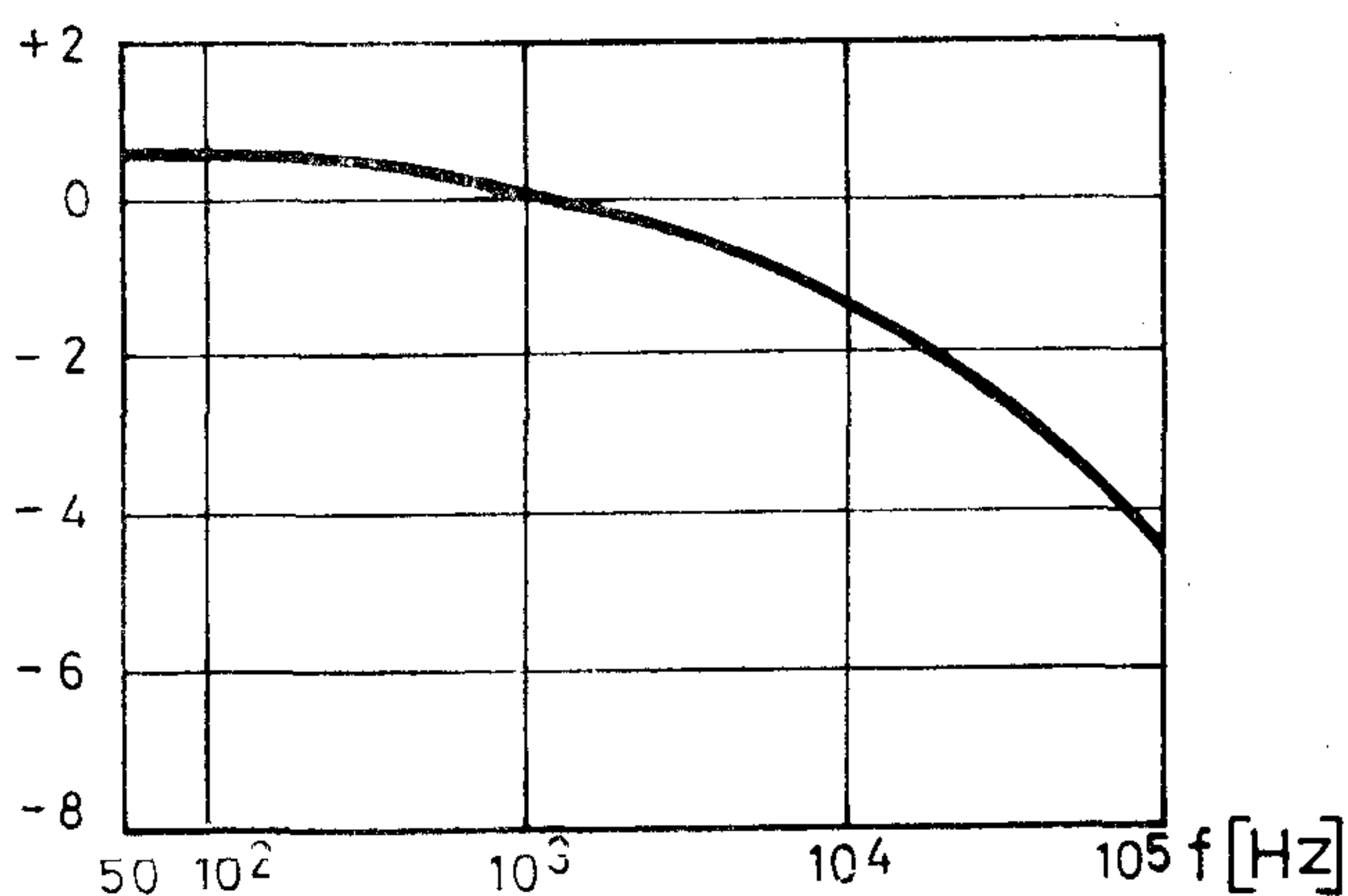
Kapacitás változás a frekvencia függvényében
