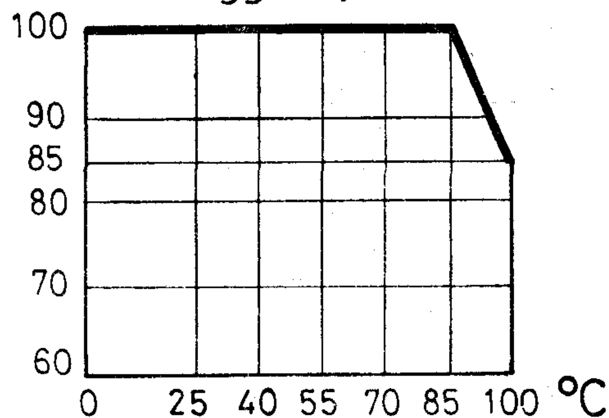
Üzemi feszültség a hőmérséklet függvényében
