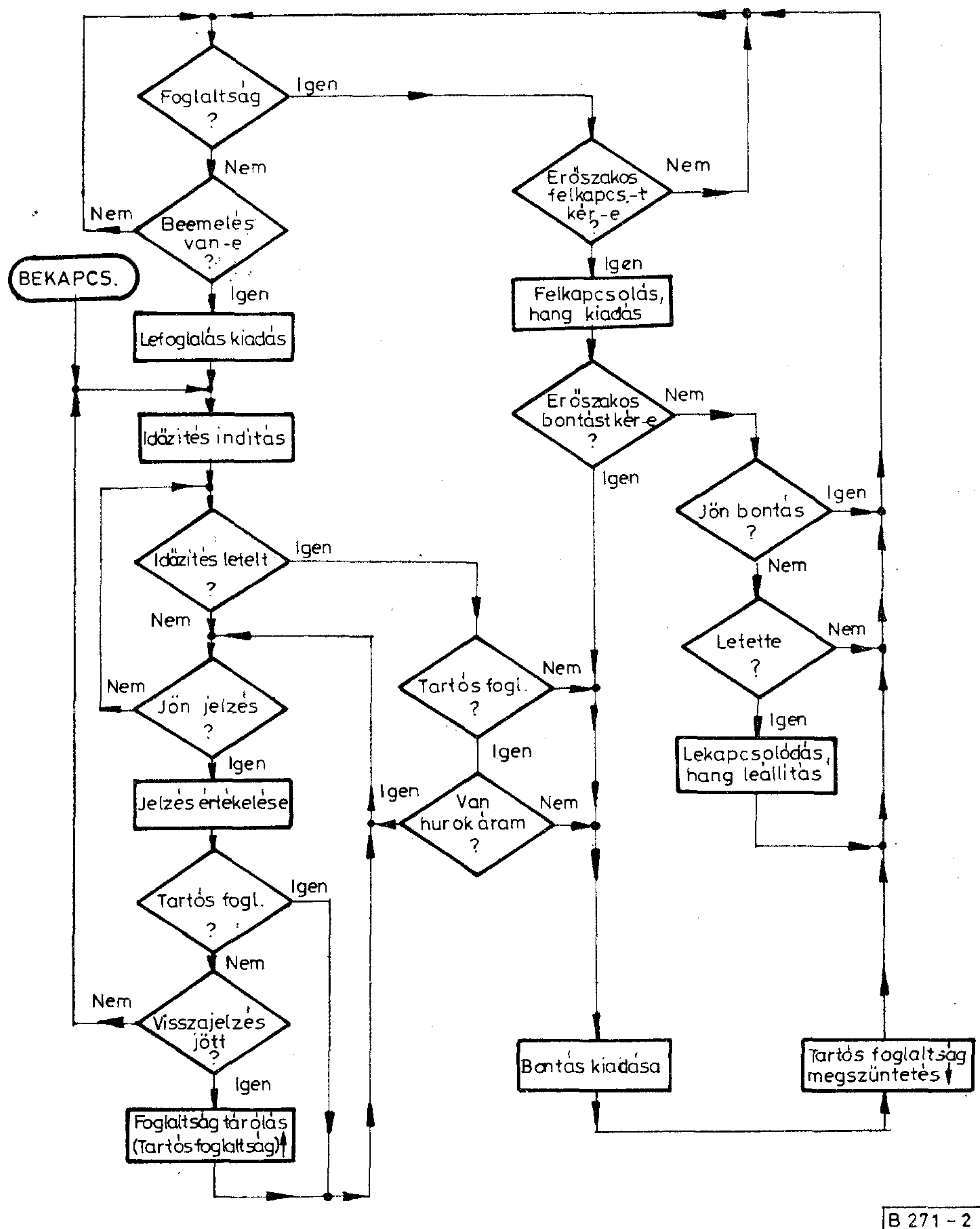
2. ábra. Decentralizált társasvonali távbeszélő rendszer mellékállomási berendezés egyszerűsített folyamatábrája
