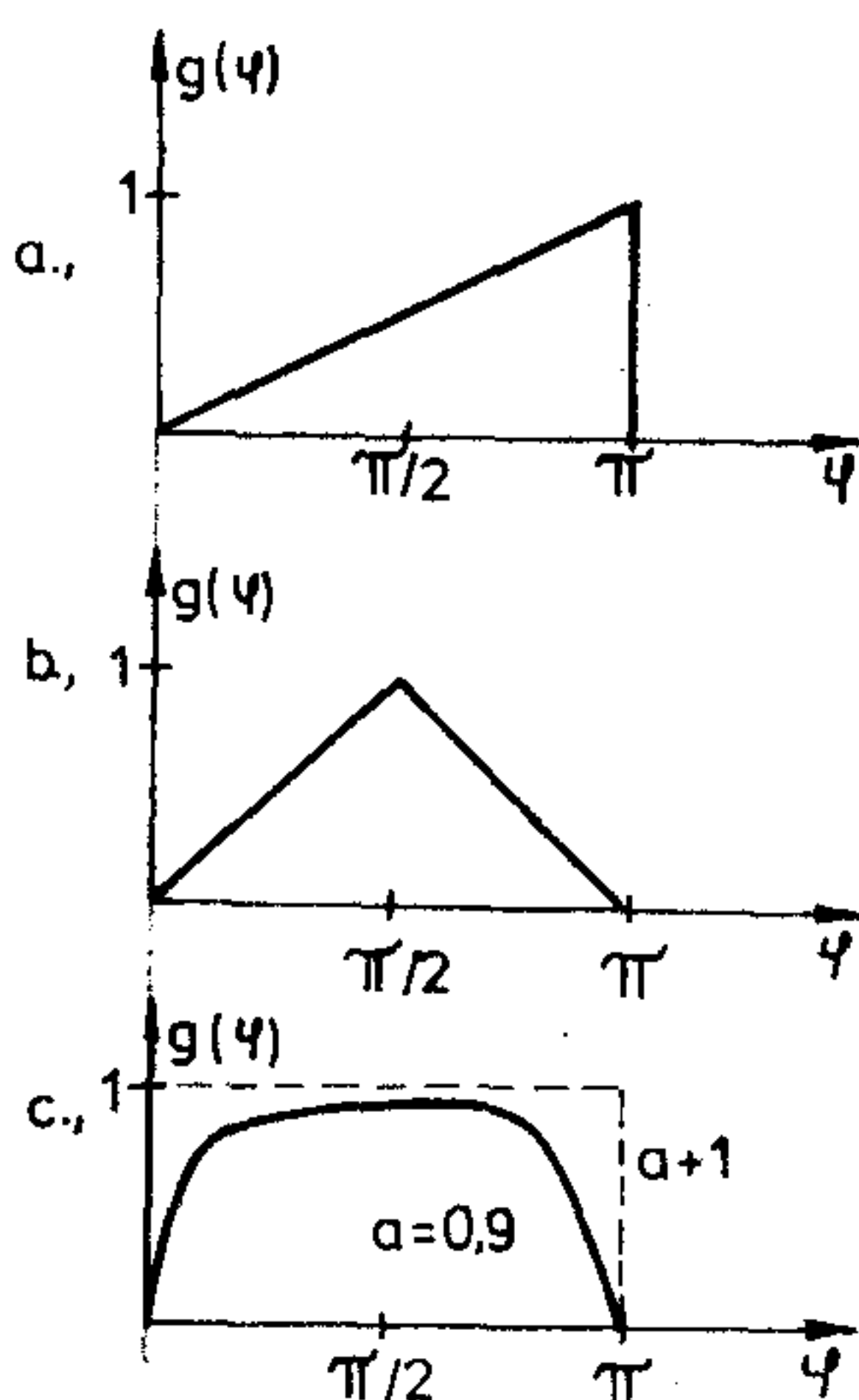
3. ábra. Néhány fontosabb Serra-függvény
