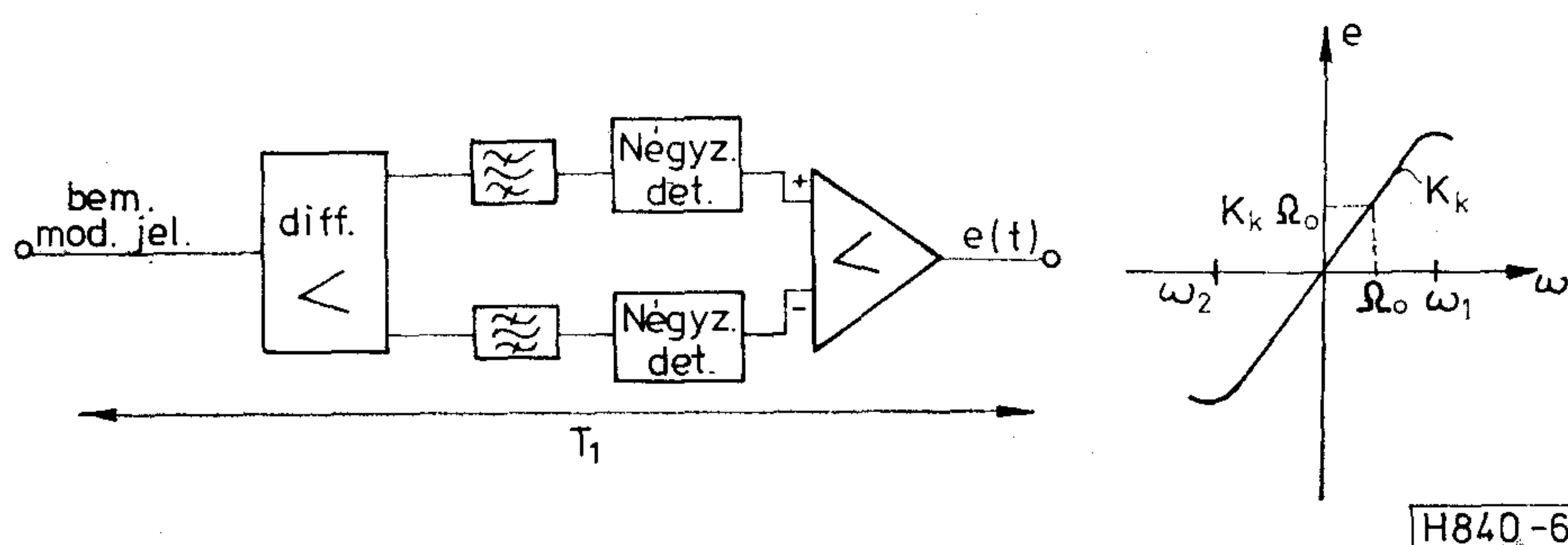
6. ábra. A spektrum-diszkriminátor blokkvázlata és jellemző karakterisztikája
