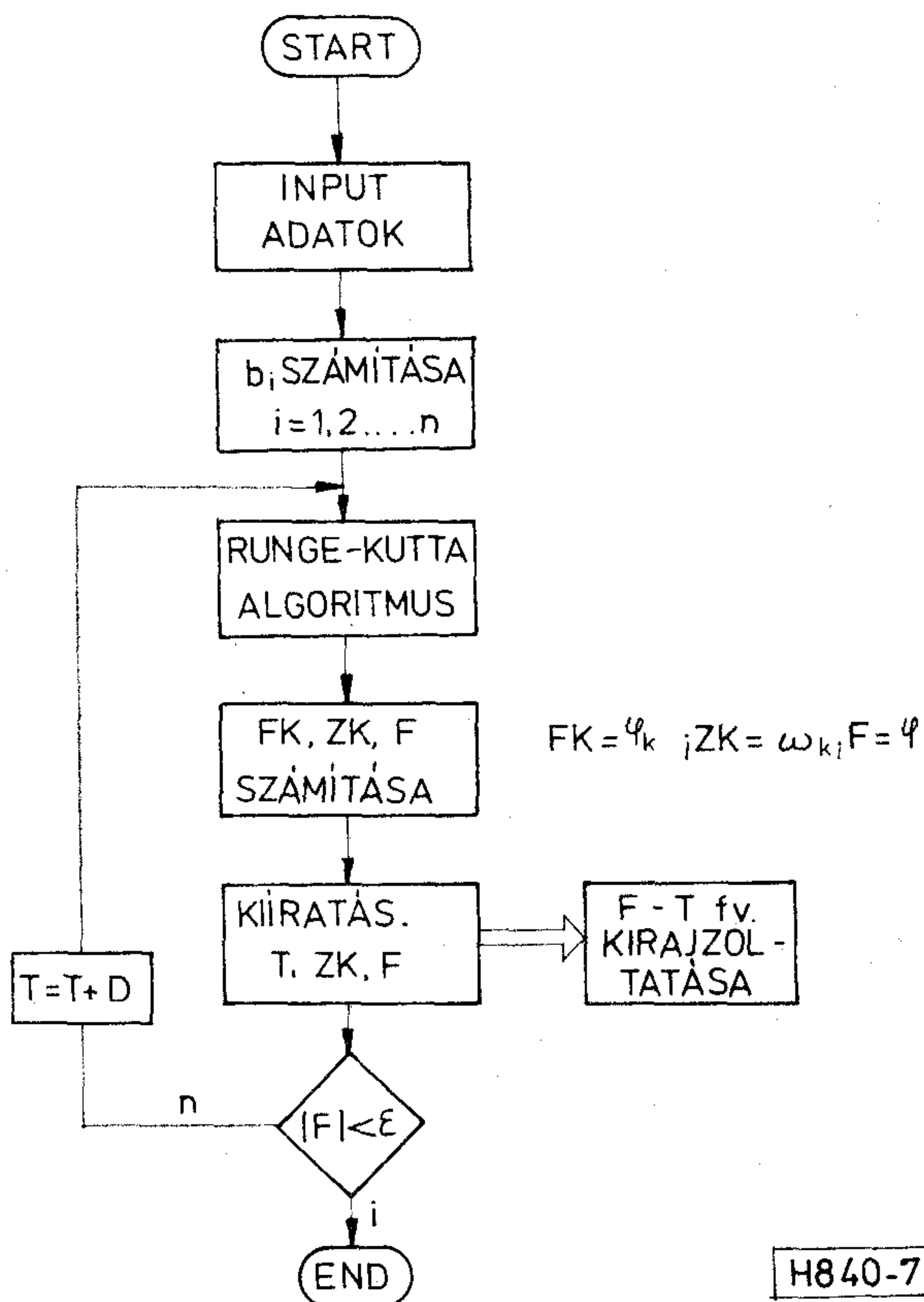
7. ábra. A tranziens-analízis program blokkdiagramja
