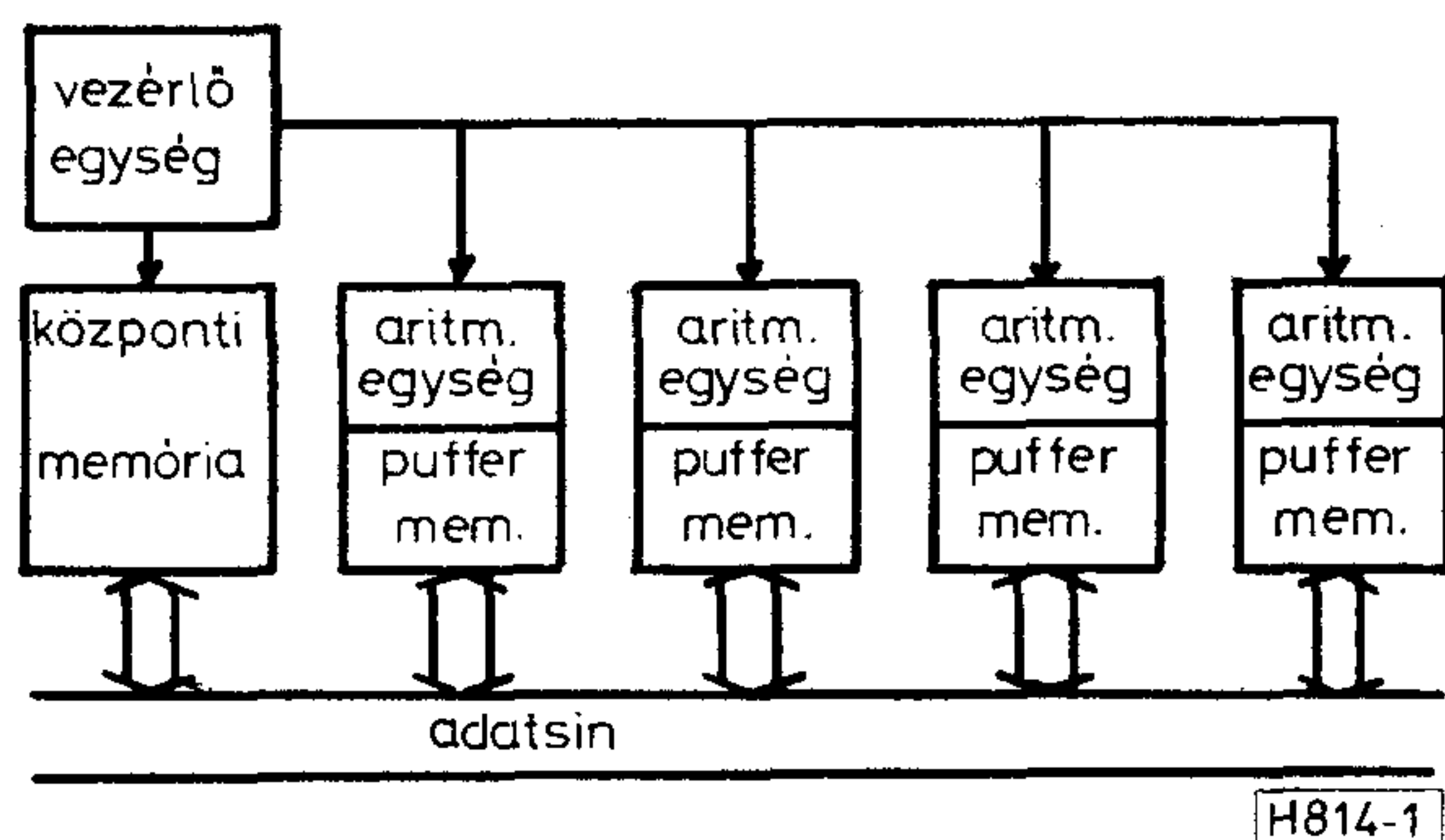
1. ábra. Tömbprocesszor-architektúra
