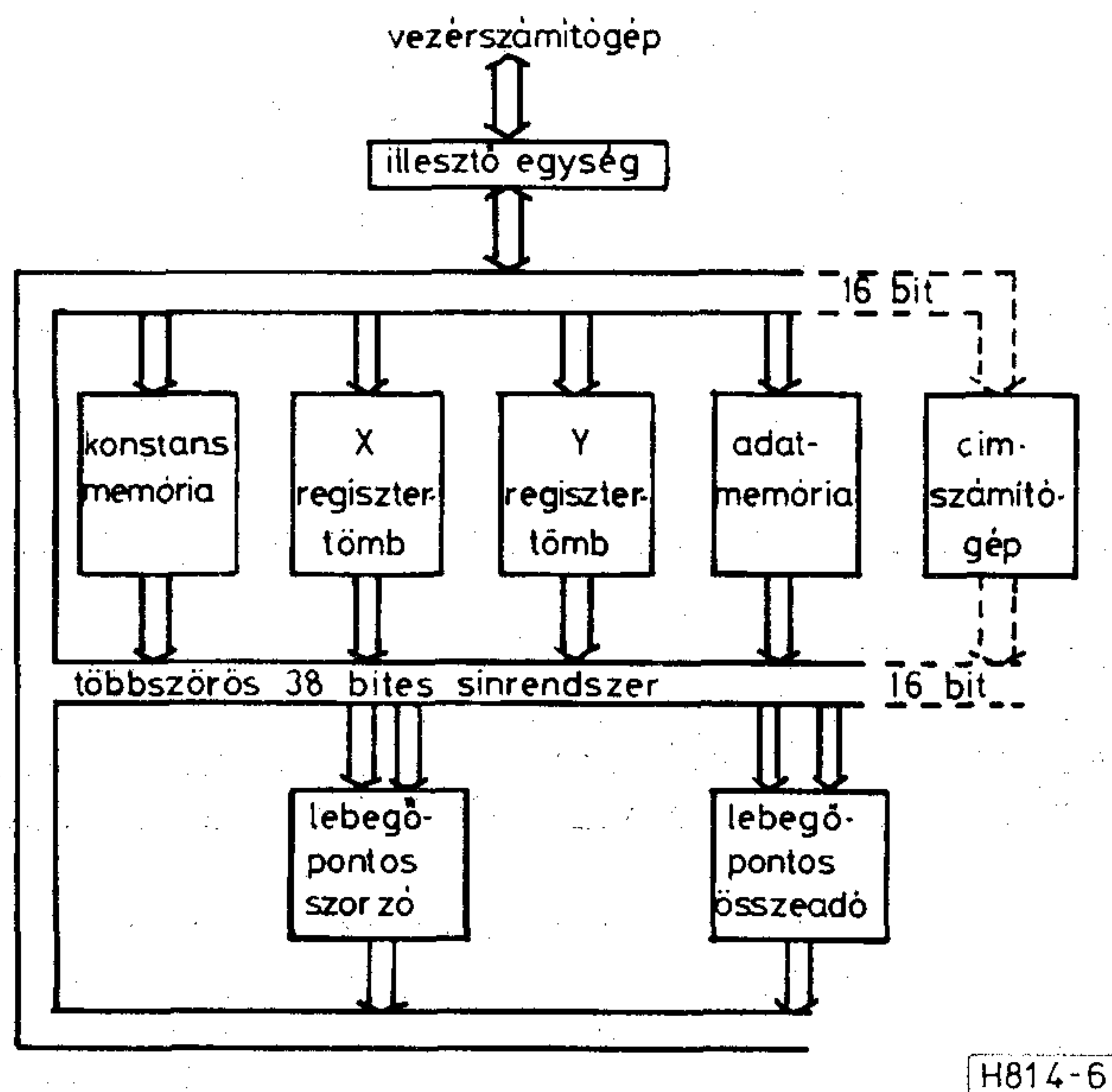
6. ábra. Az AP 120 B vektorprocesszor felépítése [3]
