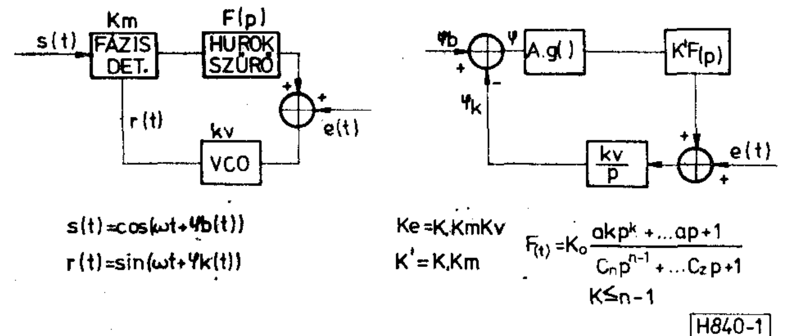
1. ábra. A PLL általános és alapsávi helyettesítőképe
