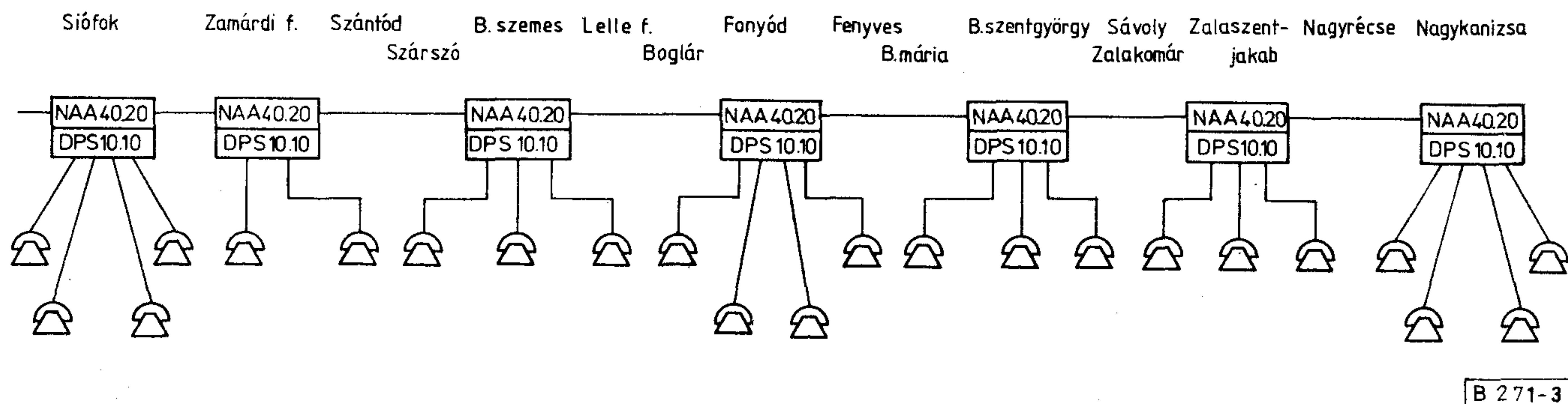
3. ábra. Siófok—Nagykanizsa vonalszakasz rendszervázlat
