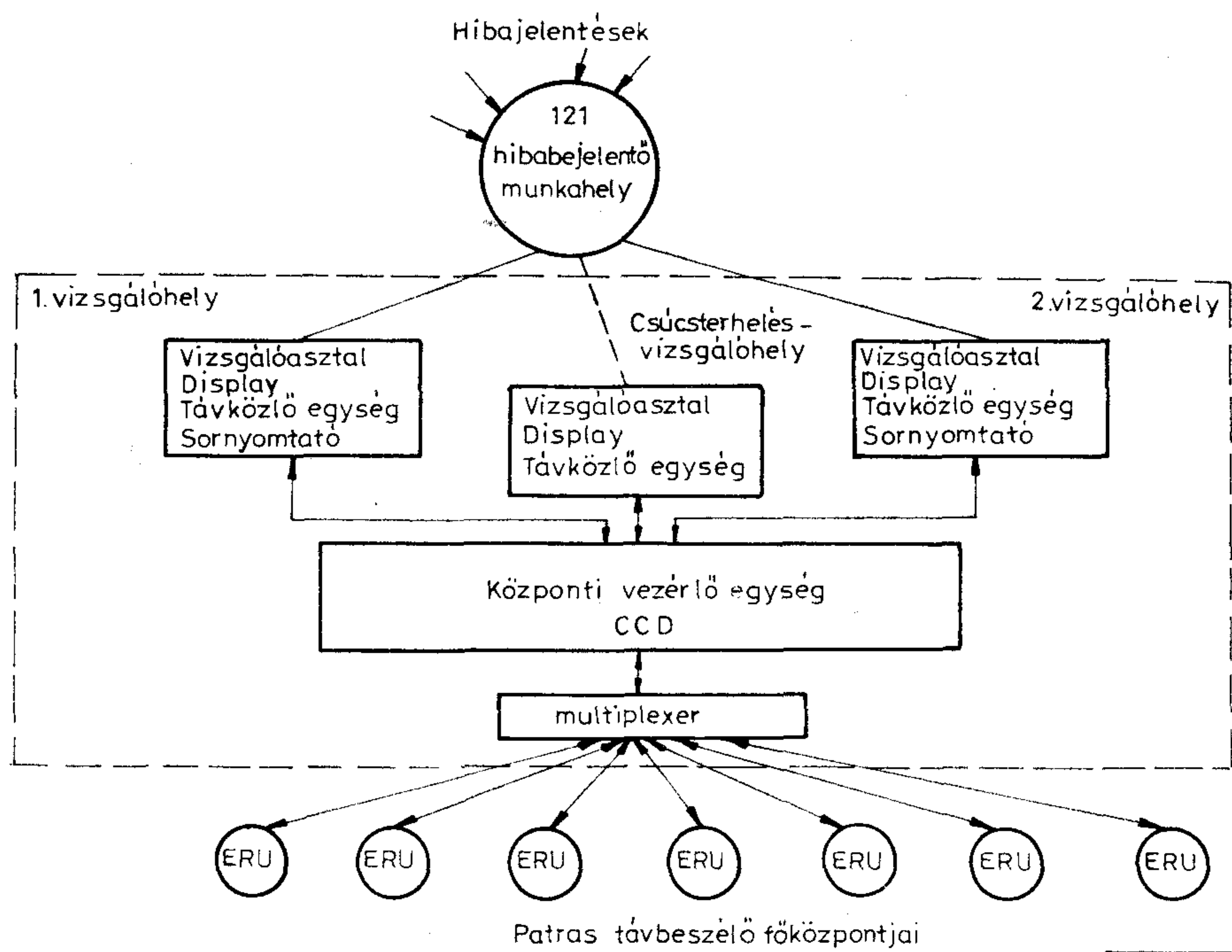
3. ábra. Az LNMCC előfizetői vonalvizsgáló (SLT) alrendszere
