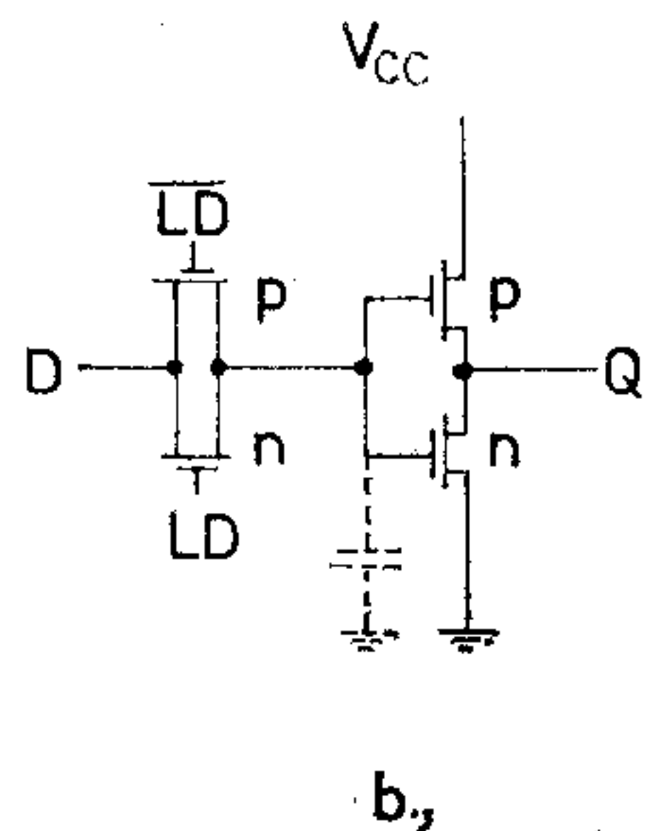
4. ábra. Példák CMOS logikai elemekre. a) komplex ÉS-VAGY-NEM kapu. b) dinamikus tároló egy bitje
