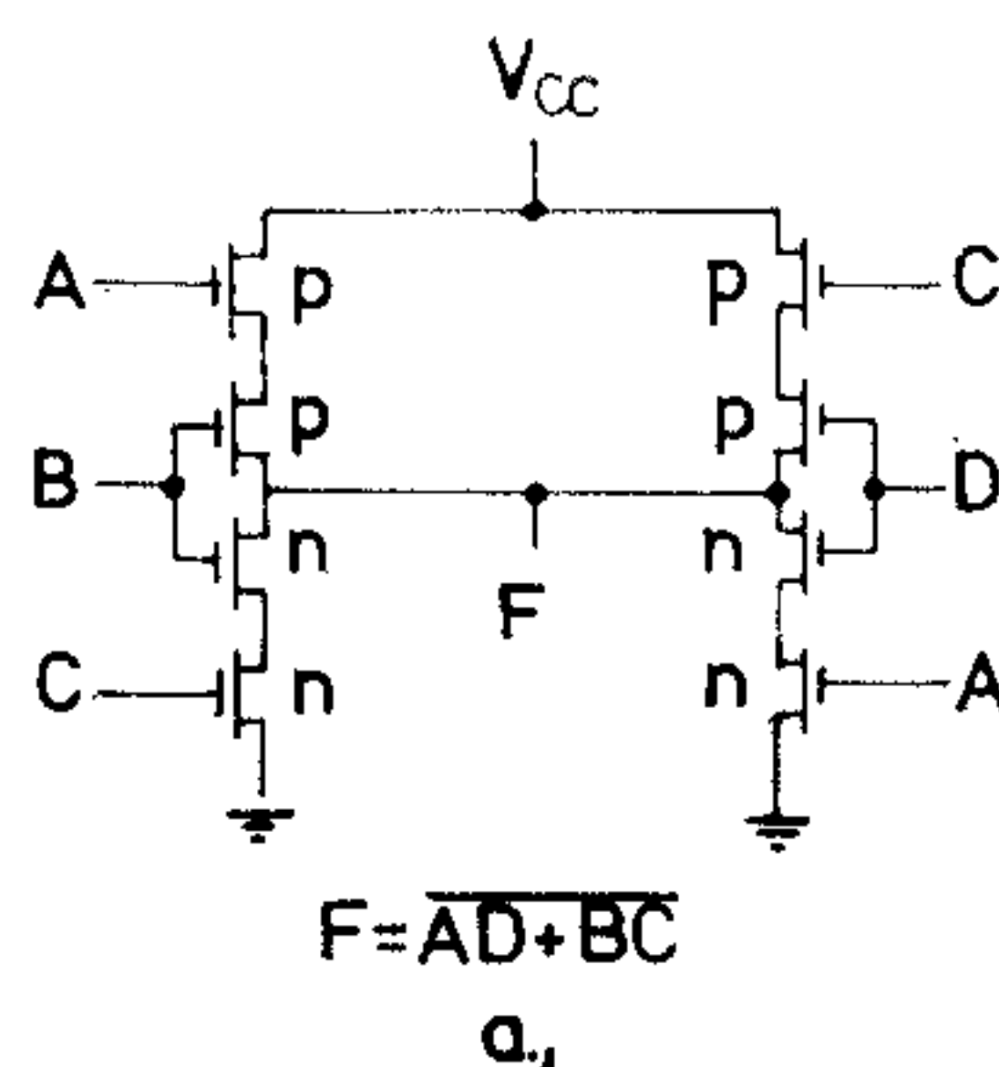
4. ábra. Példák CMOS logikai elemekre. a) komplex ÉS-VAGY-NEM kapu. b) dinamikus tároló egy bitje
