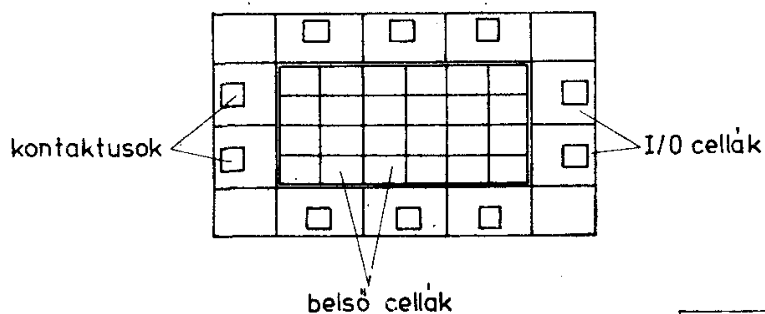
3. ábra. Gate array áramkör belső felépítése
