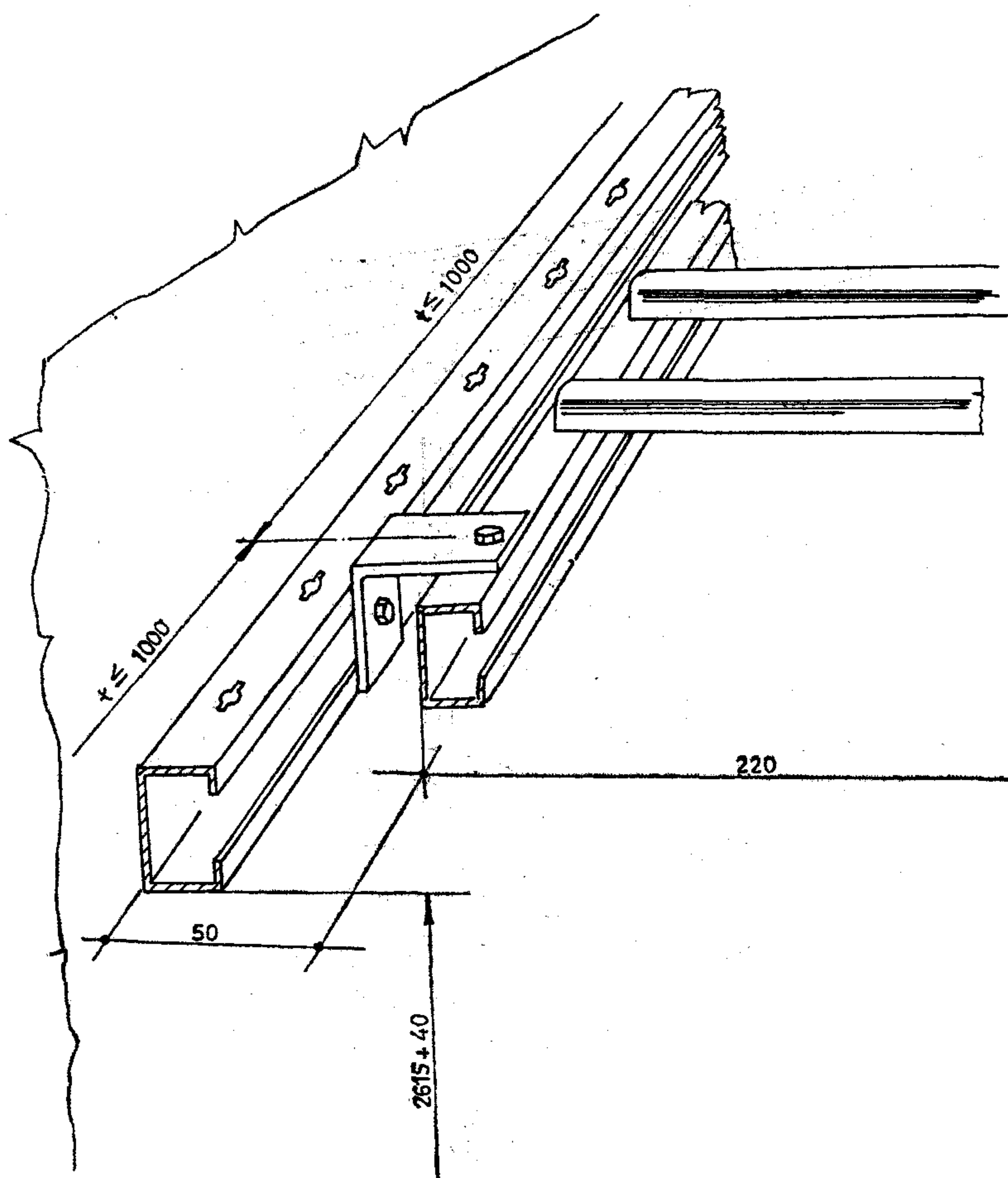
3. ábra. A fal melletti kábelletrásor részlete
