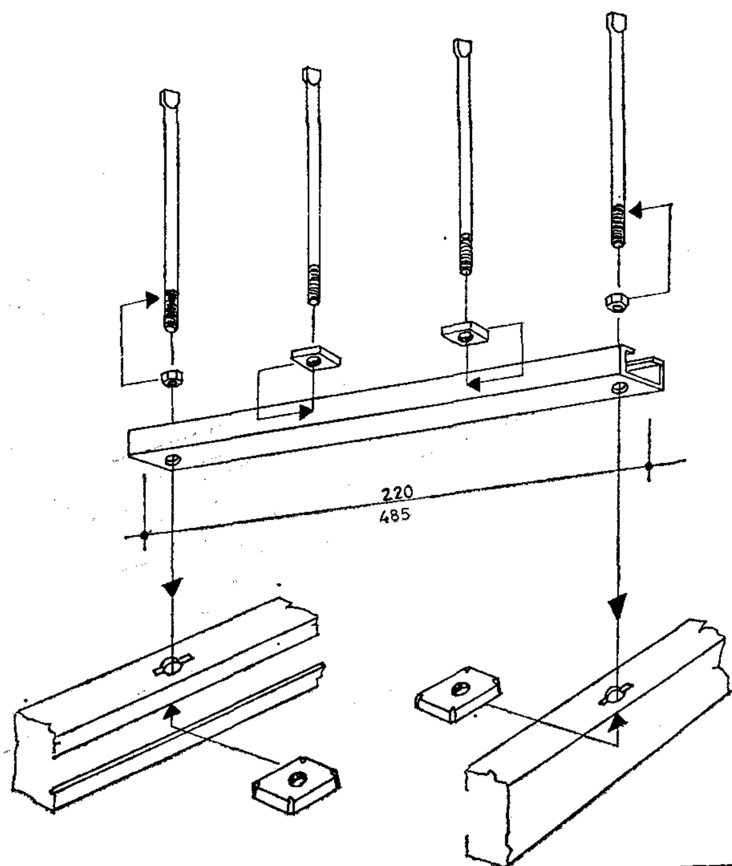
11. ábra. Az „osztott” kivitelű létrafok kialakítása
