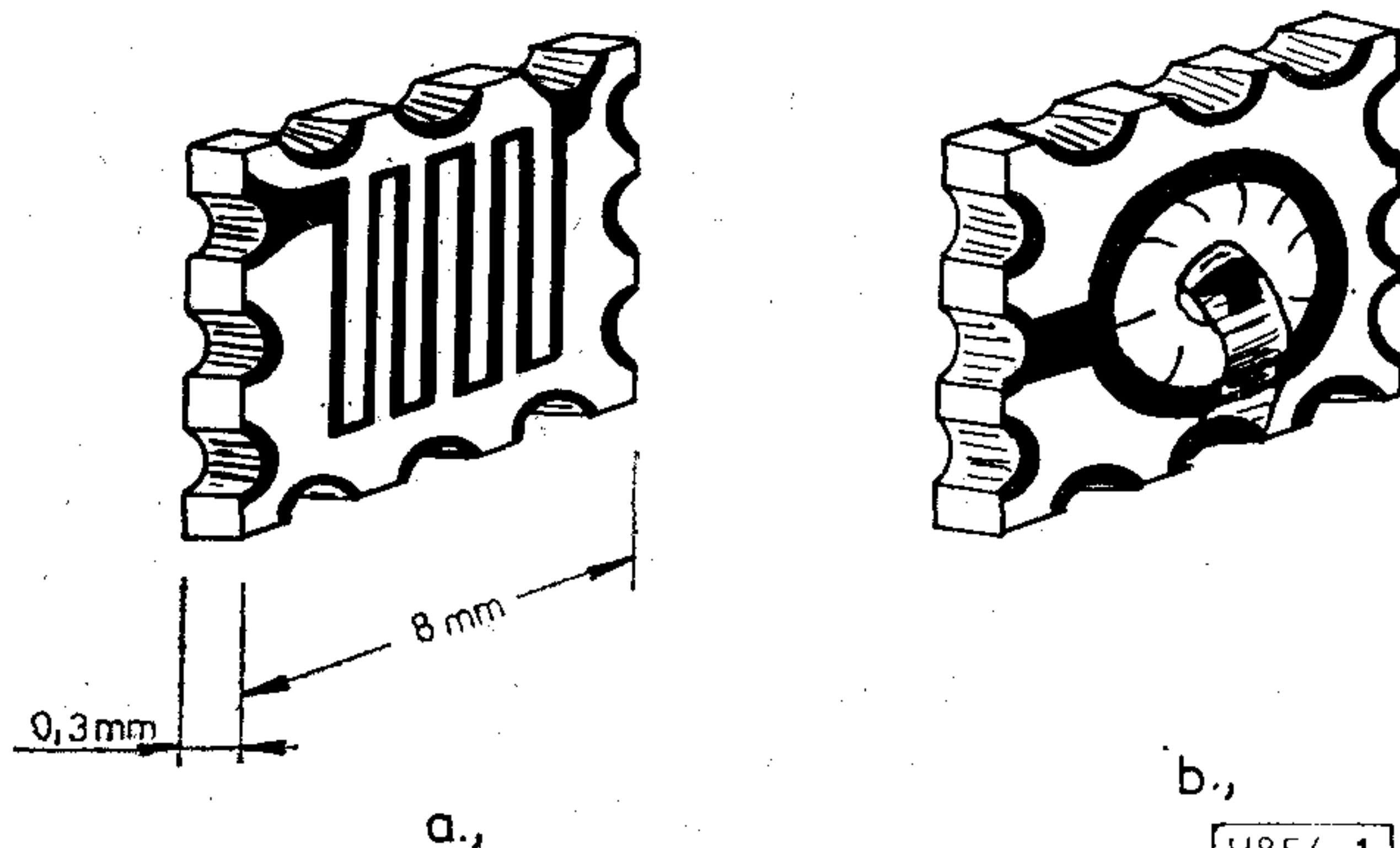
1. ábra. Mikromodul-lapok (1959)
