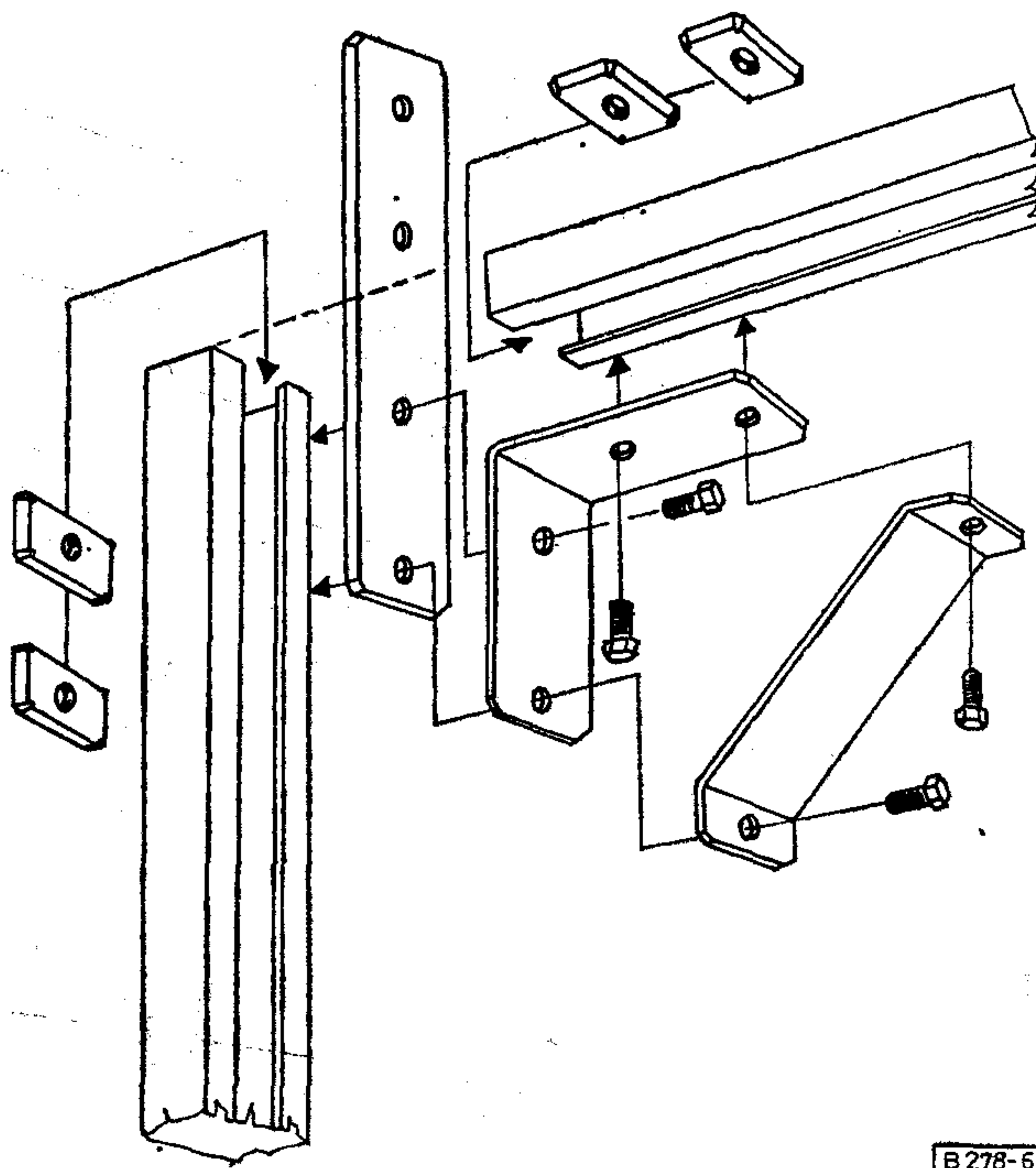
6/b ábra. A tartóoszlop felső sarokpontjának kialakítása
