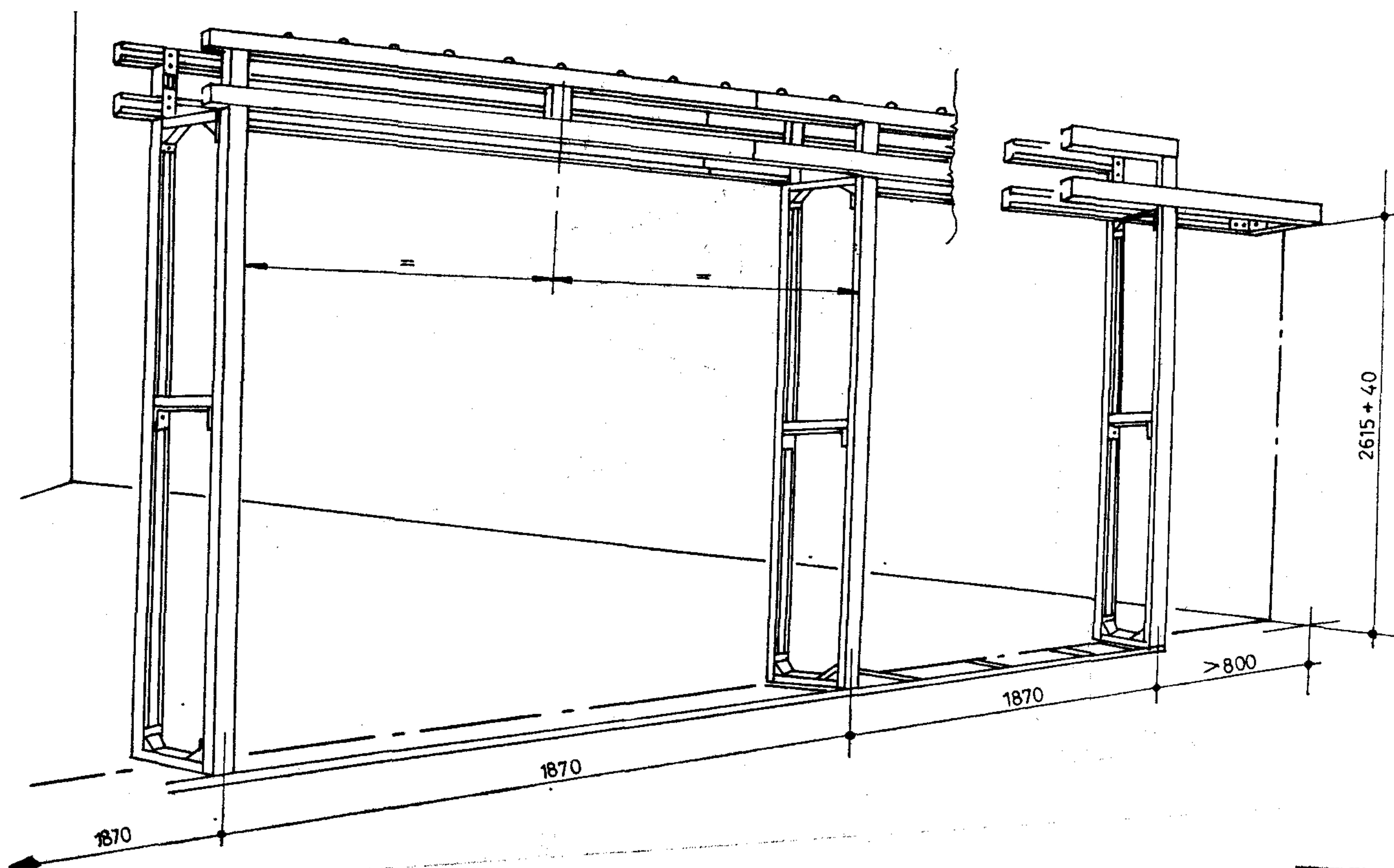
2. ábra. A szabadon álló kábelletrásor
