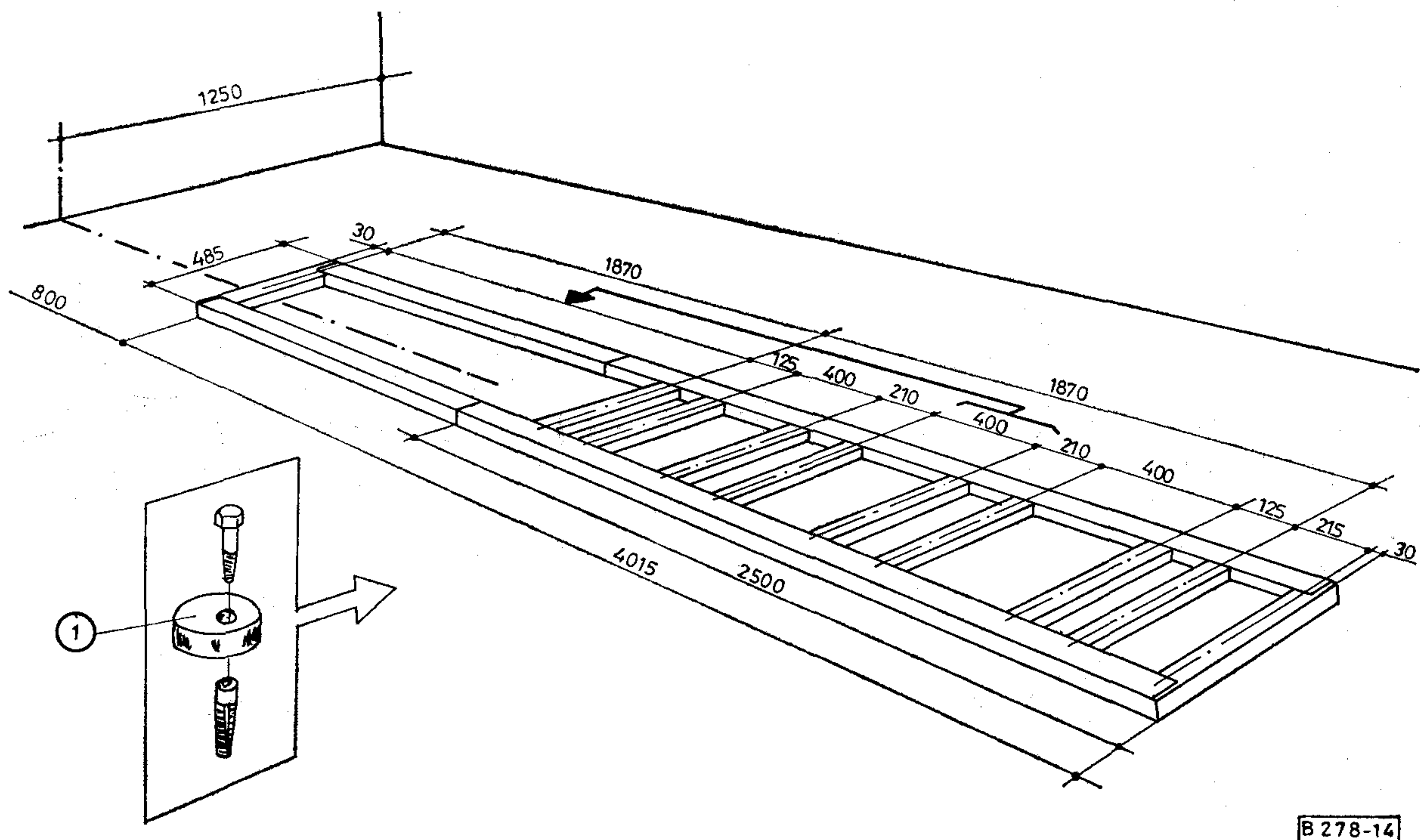
14. ábra. Az alapzatszerelvény részlete
