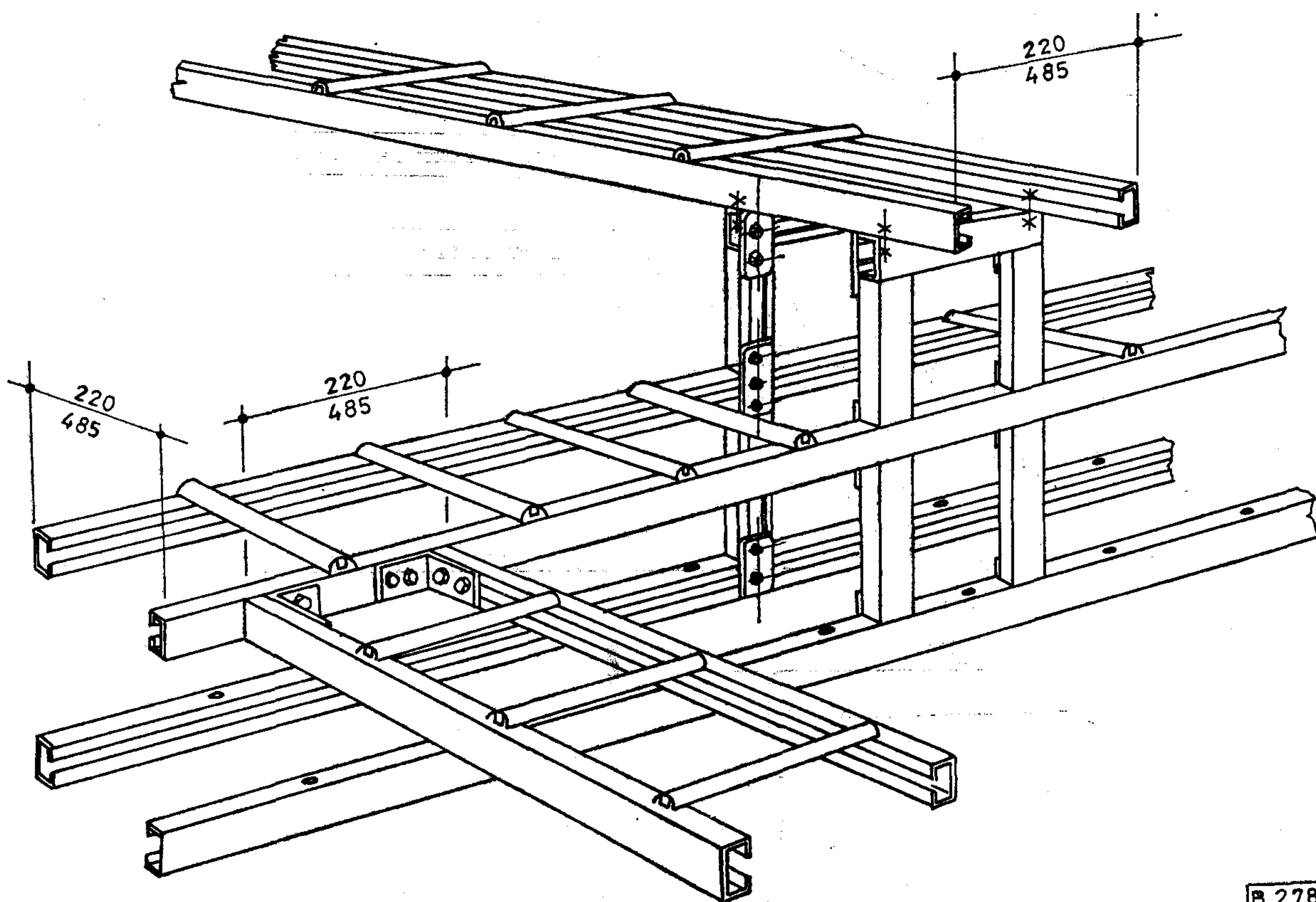
5. ábra. A kábeltrahíd részlete
