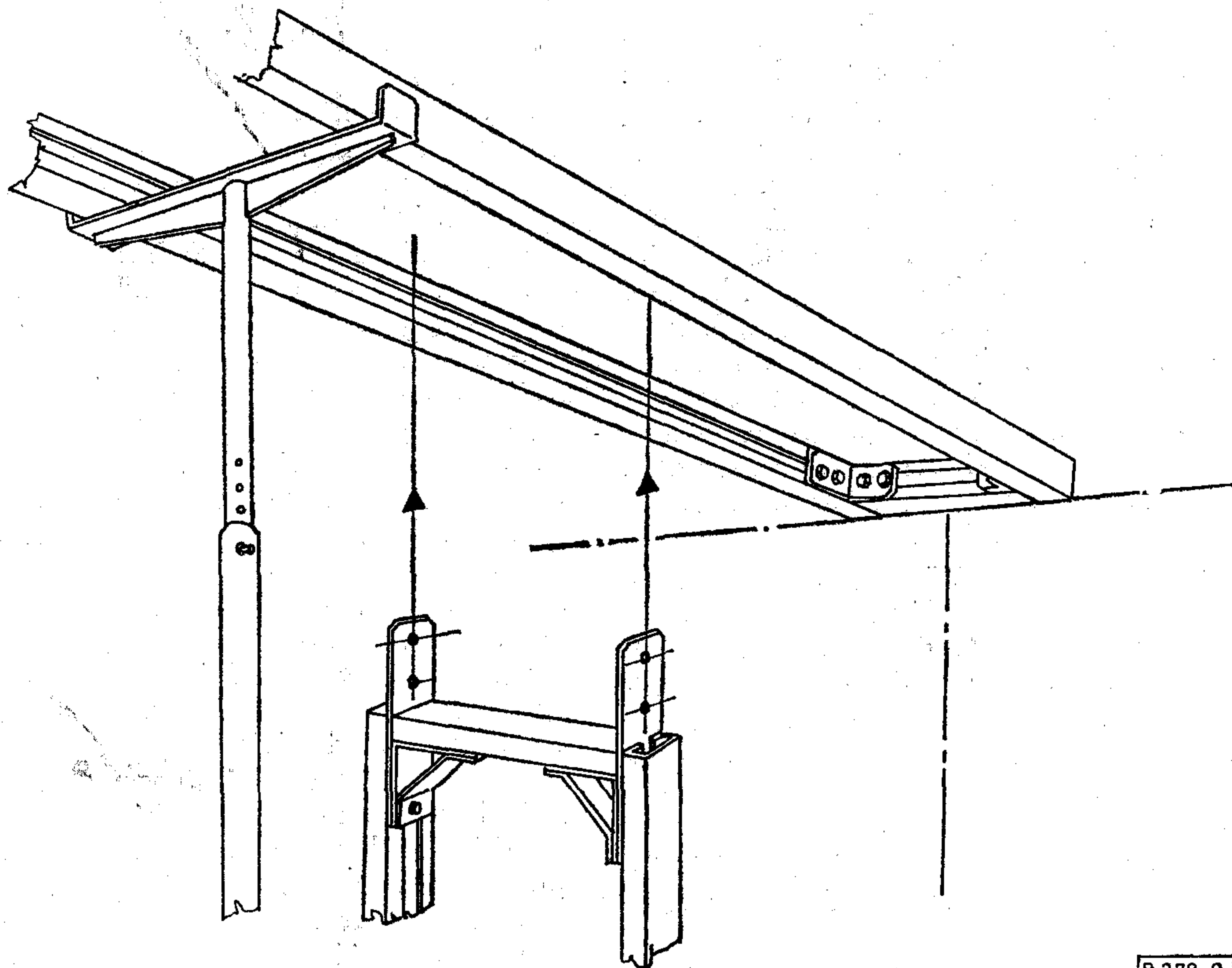
9. ábra. A kábellétra-kitámasztó segédeszköz
