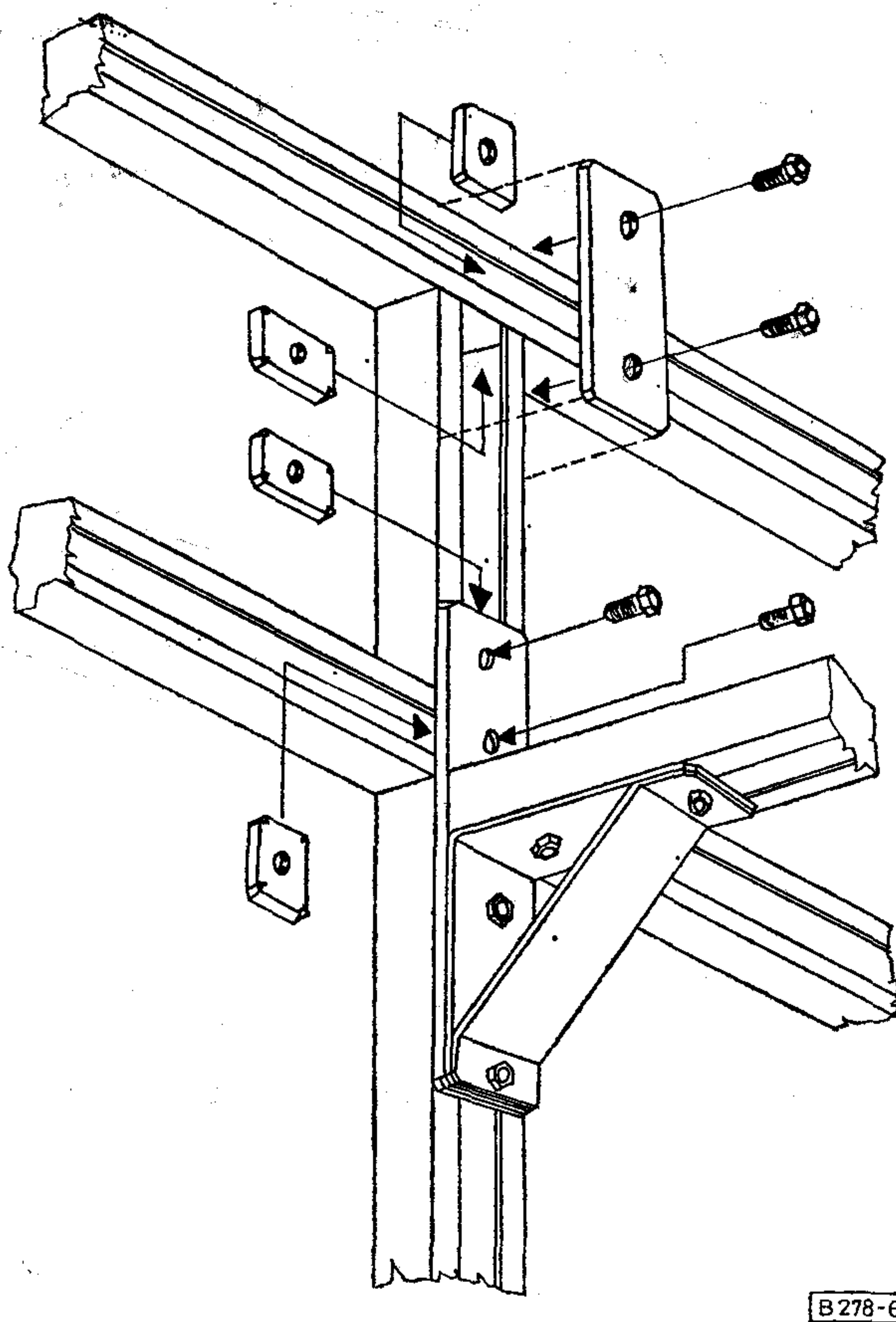
6/a ábra. A tartóoszlop és a sorlétra csatlakoztatása
