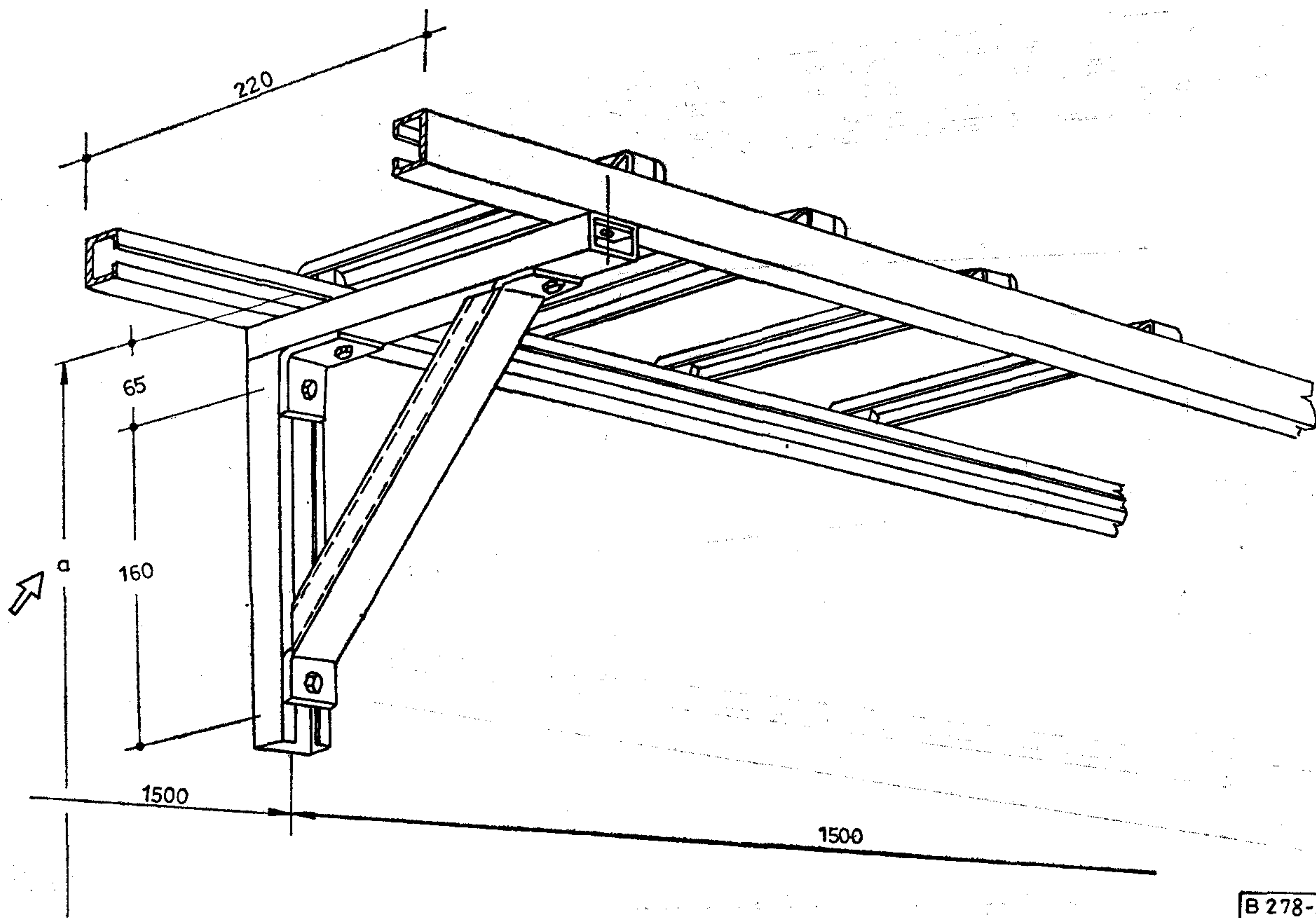
4. ábra. A falra szerelt kábeltráyor részlete
