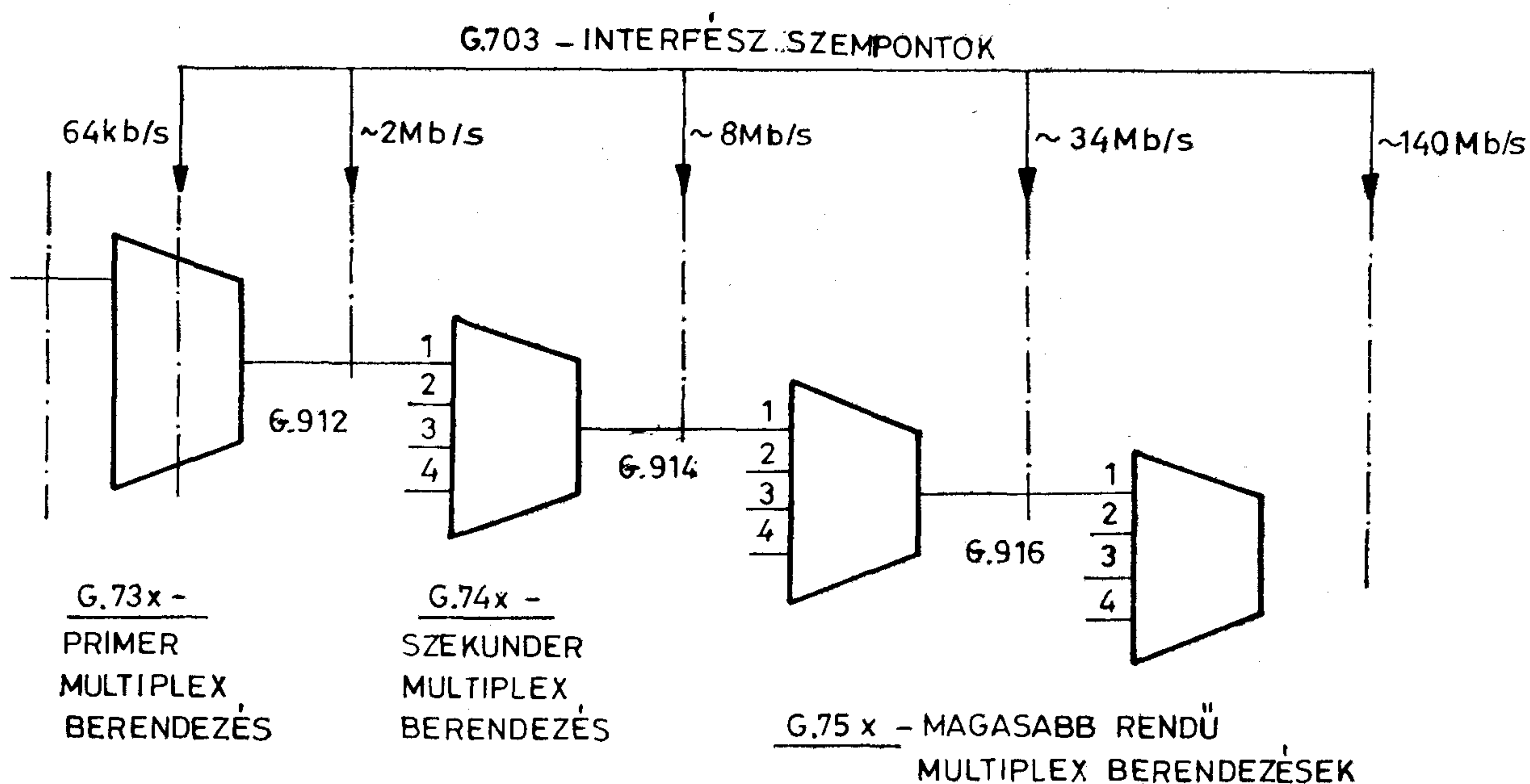
1. ábra. A CCITT európai digitális átviteli hierarchiája
