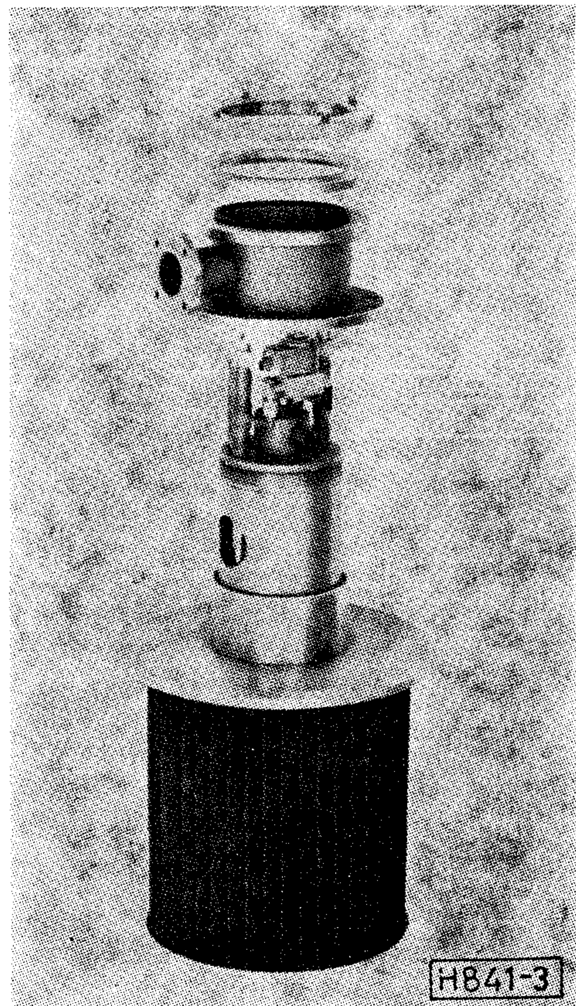
3. ábra. Merülő, vagy fürdő ultravákuum kryosztát
