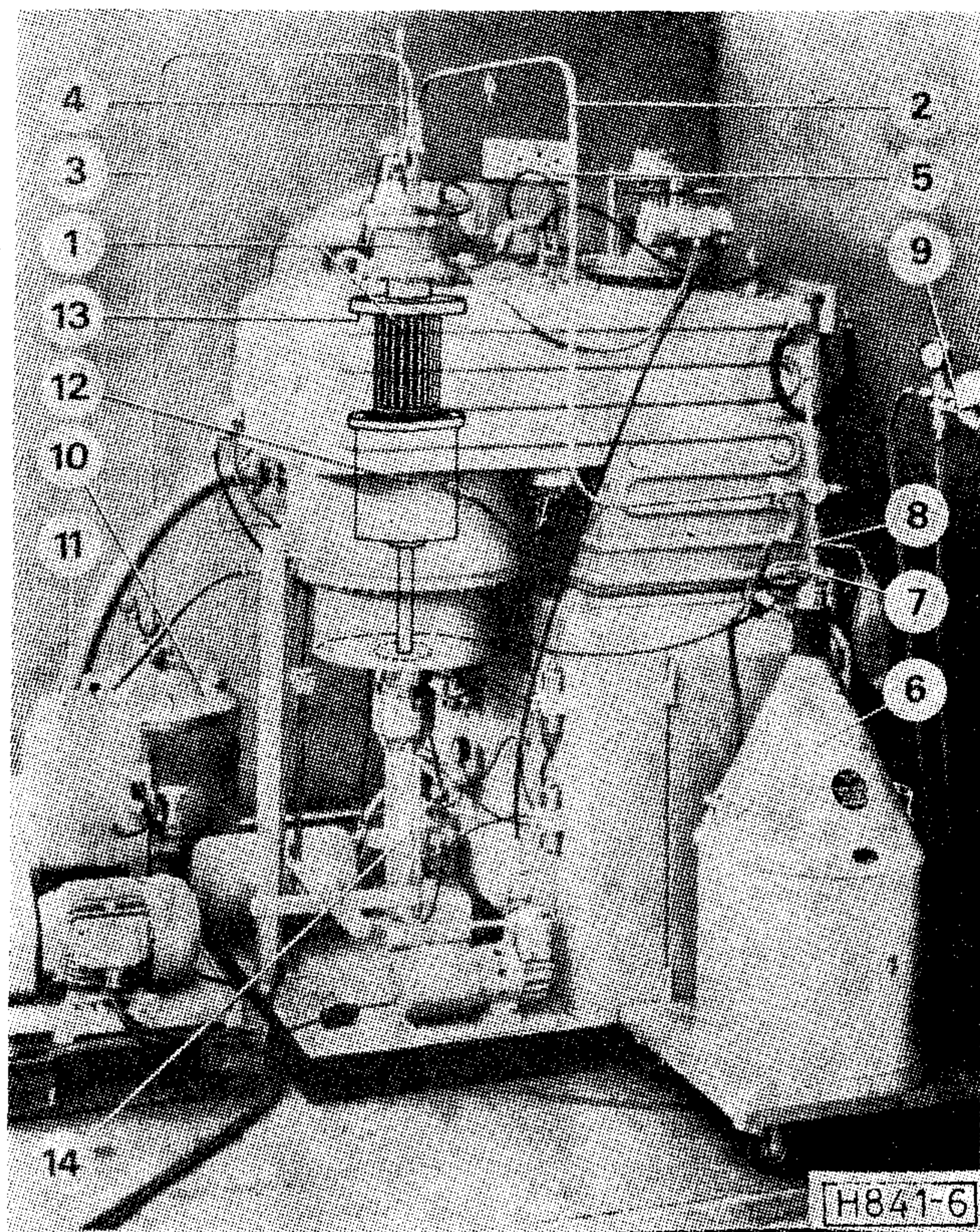
6. ábra. Komplet szuper-ultravákuum gőzölő berendezés Kry. 5000 l/sec kryosztáttal. 1 kryoszivattyú, 2 cseppfolyós héliumot szállító vákuum szigetelt vezeték, 5 hélium vivő szabályzó, 6 héliumtároló, 10 nitrogént tároló edény, 11 elővákuum szivattyú
