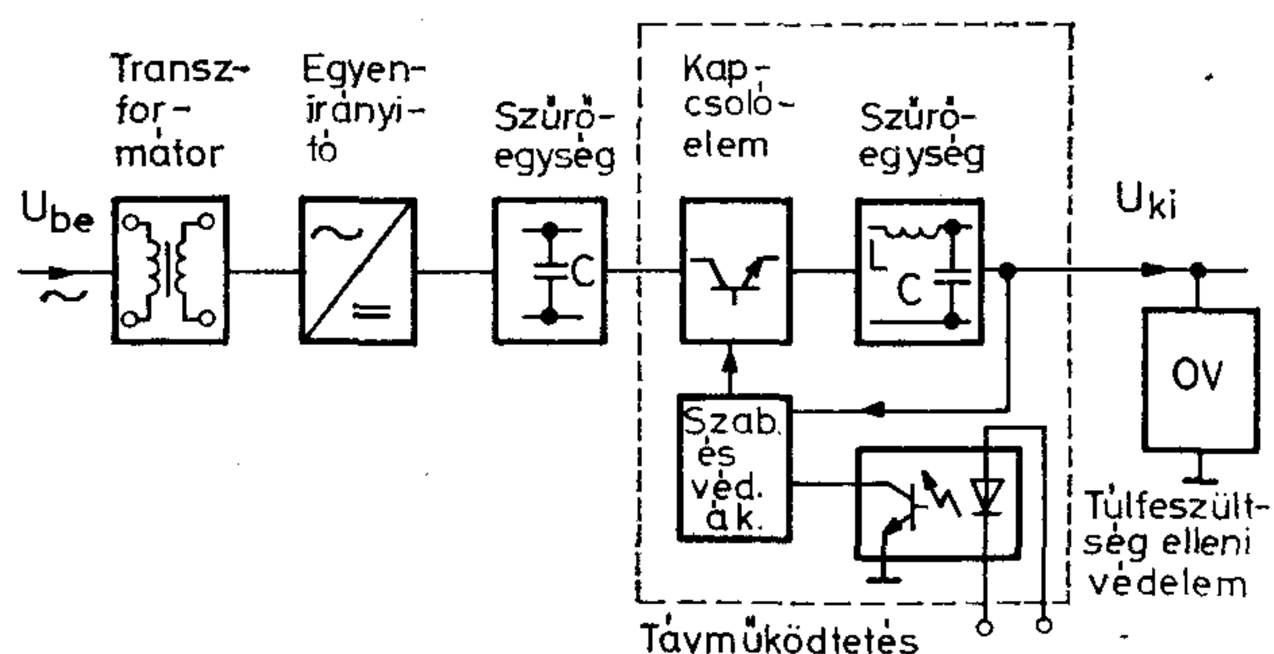
7. ábra. Soros kapcsolóüzemű stabilizátorral felépített tápegység blokk-sémája
