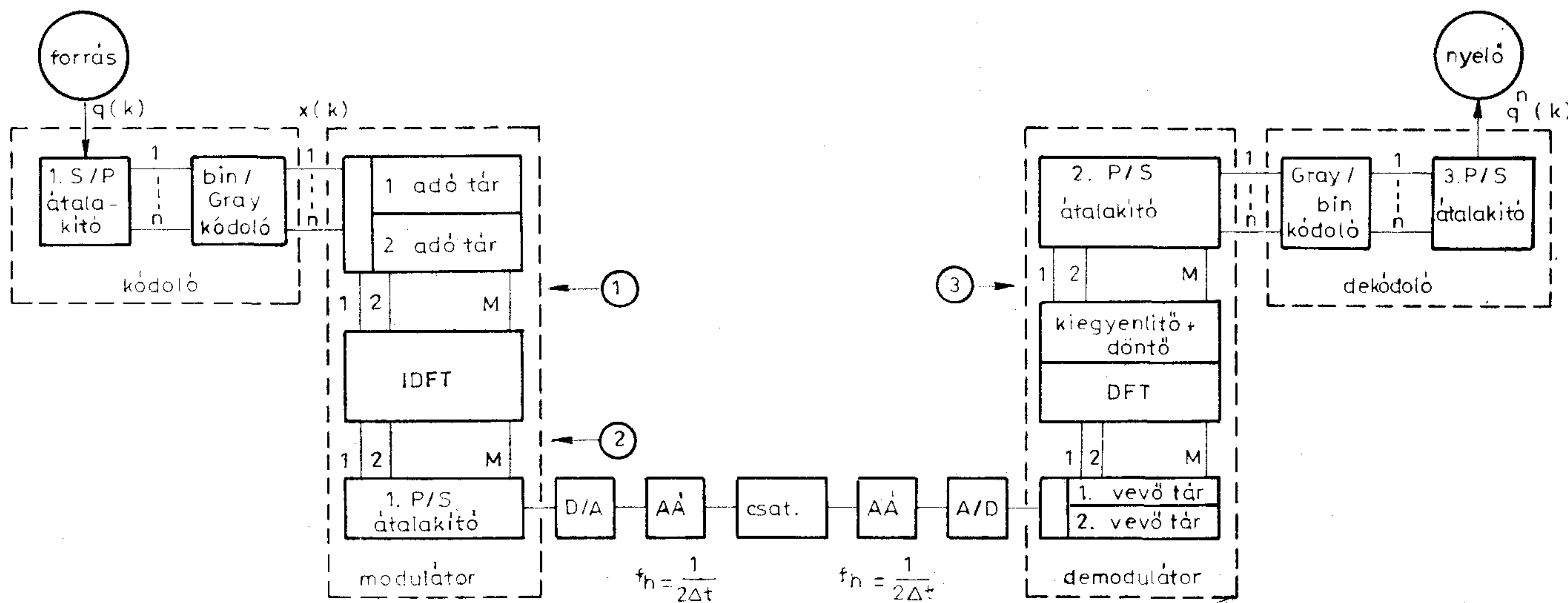
2. ábra. Az eljárásra épülő modem rendszerteknikája
