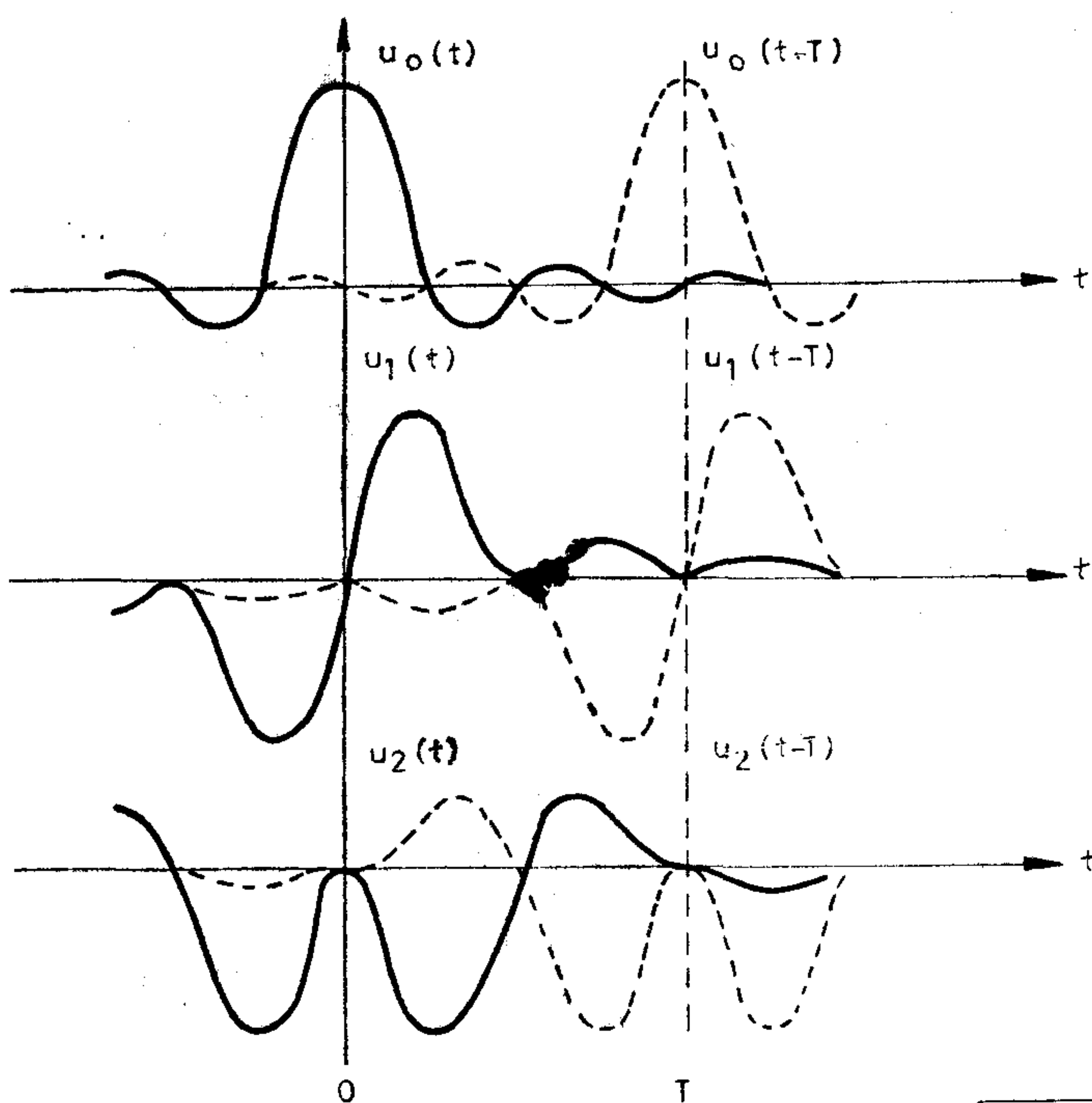
8. ábra. Tágabb értelemben orthogonális időfüggvények
