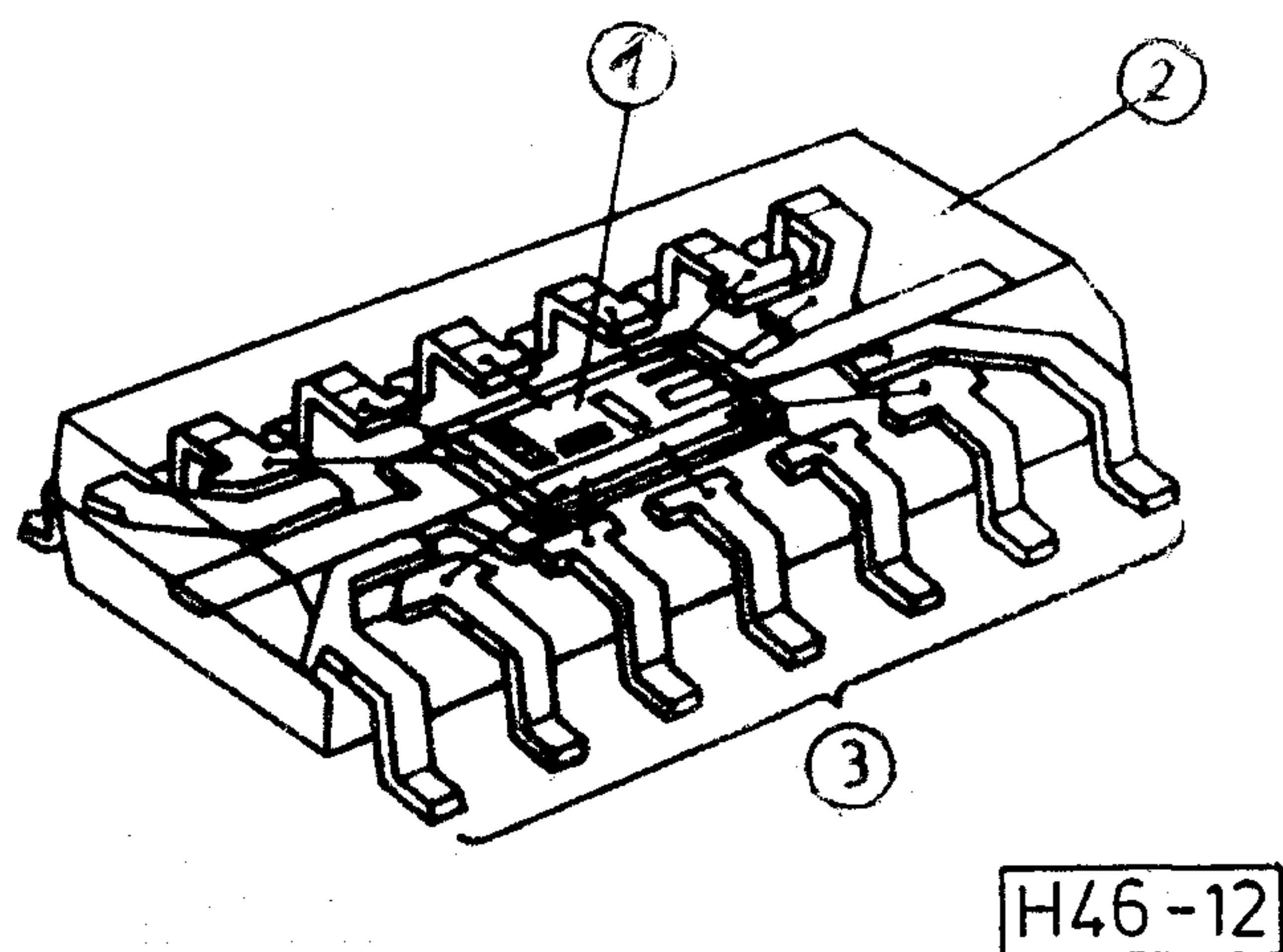
12. ábra. Mikrotokozott félvezetők 1 — a félvezető morzsa (chip); 2 — hőálló műanyag tok; 3 — kivezetők
