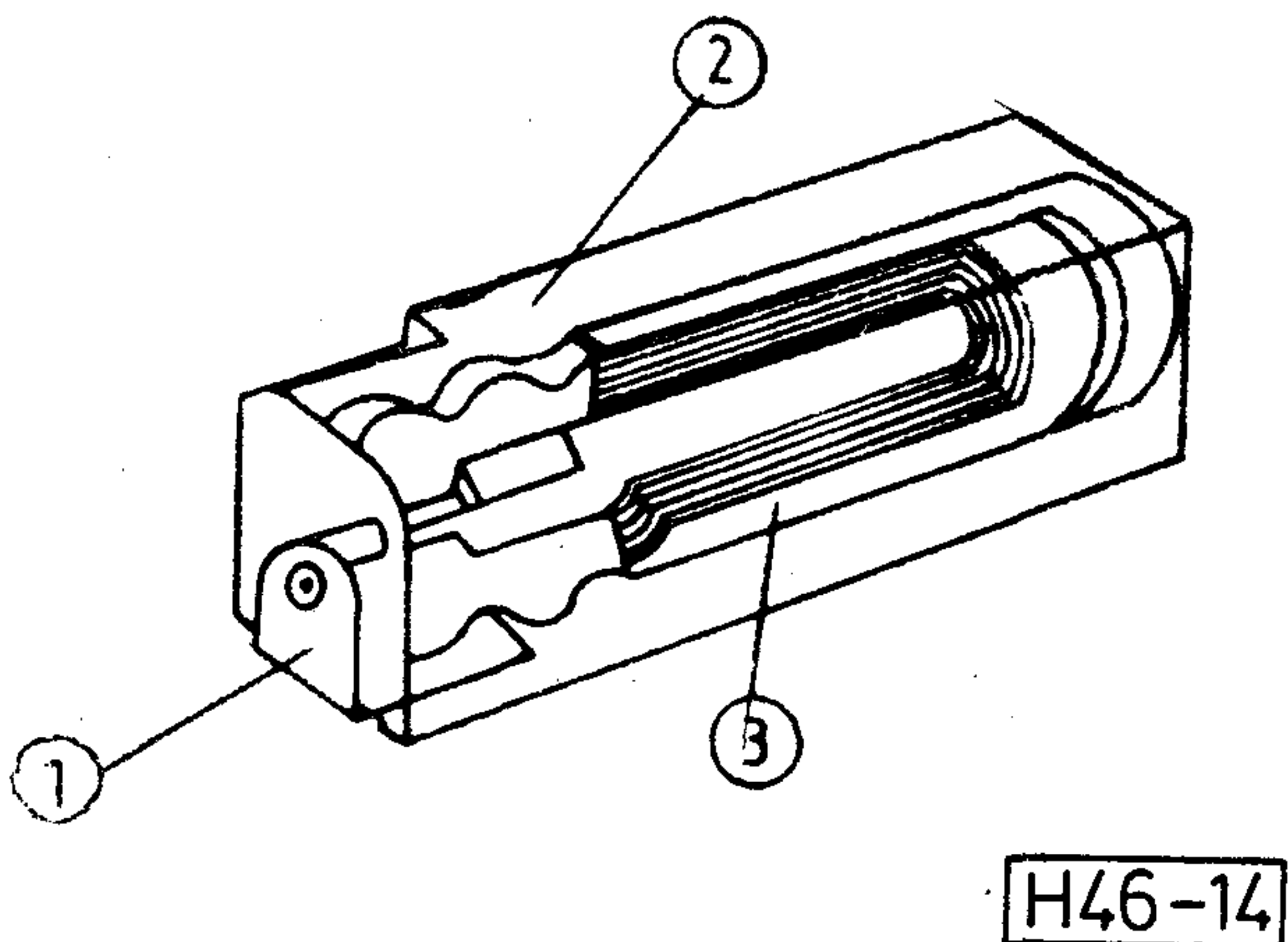
14. ábra. Elektrolit-kondenzátor 1 — anódkivezető és forraszfelület; 2 — hőálló szigetelő tok; 3 — kondenzátor tekercs (Philips)
