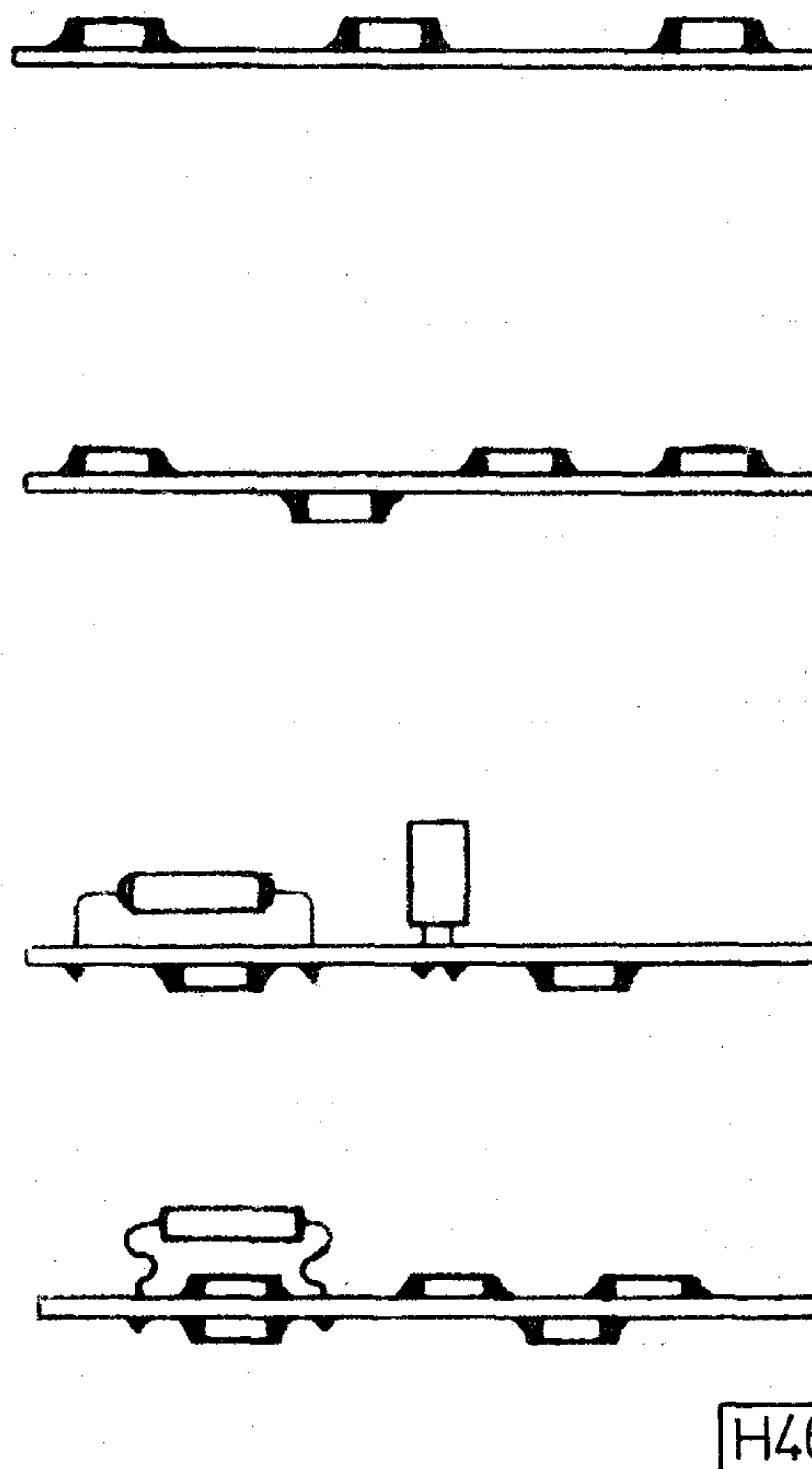
8. ábra. A felületszerelt alkatrészek elhelyezési lehetőségei a nyomtatott áramköri lemezen. A hagyományos és az új szerelés kombinációja is megfér a gyakorlatban
