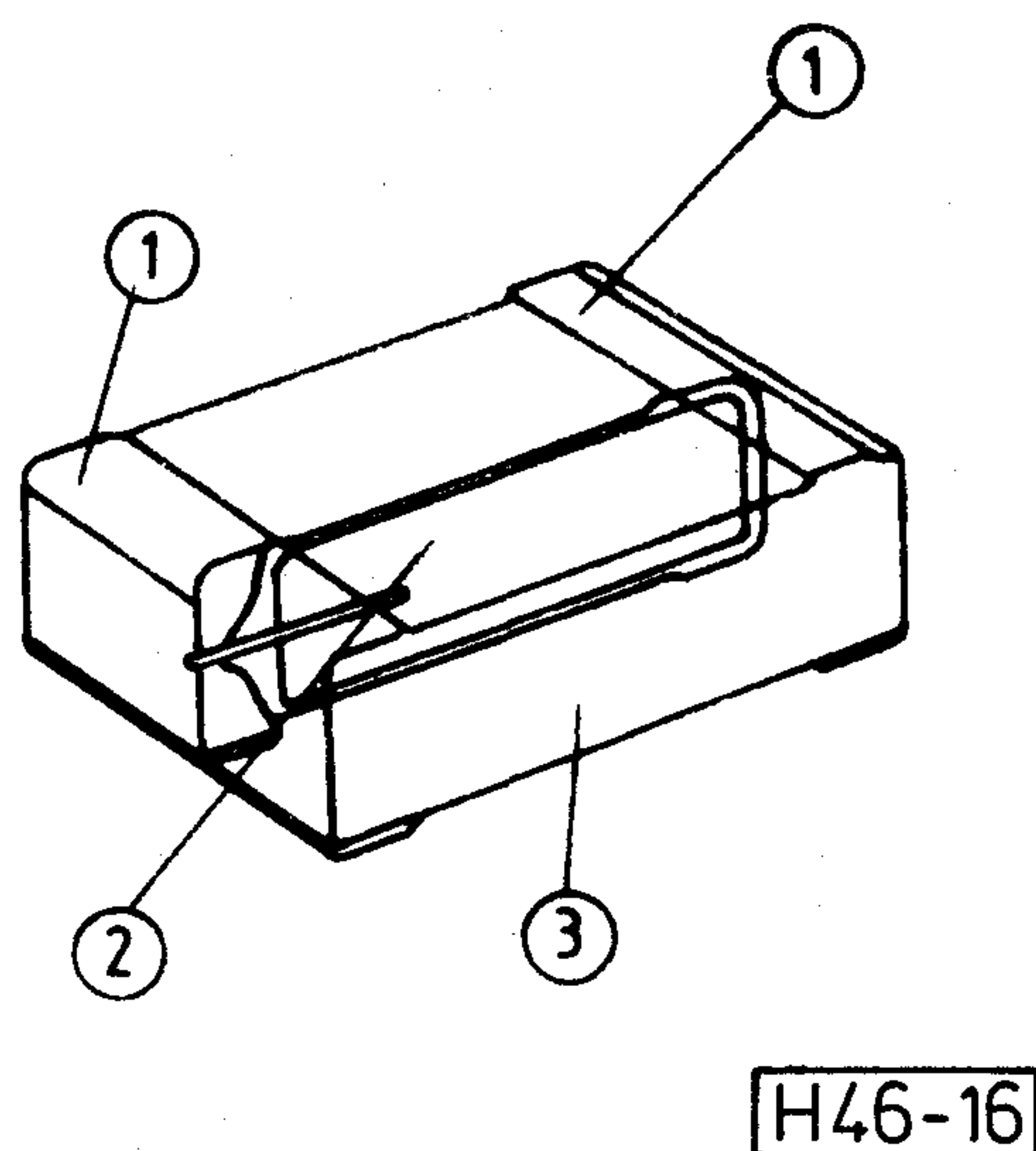
16. ábra. Tantál chipkondenzátor 1 — forraszható anód-, ill. katód-kivezetés; 2 — \text{Ta}_2\text{O}_5 — \text{MnO}_2 szinterfest; 3 — burkolat
