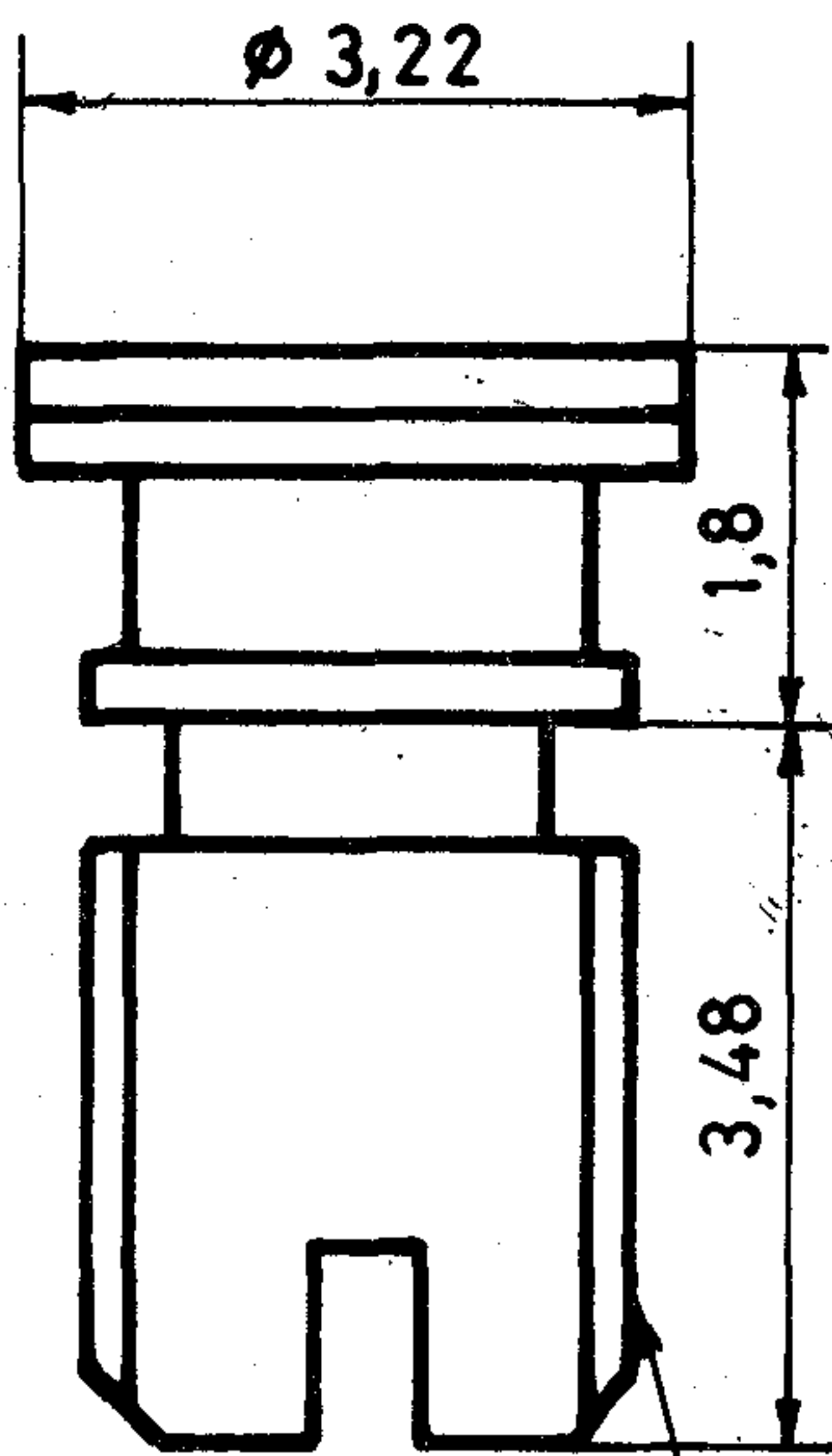
3-48 UNC 2A
