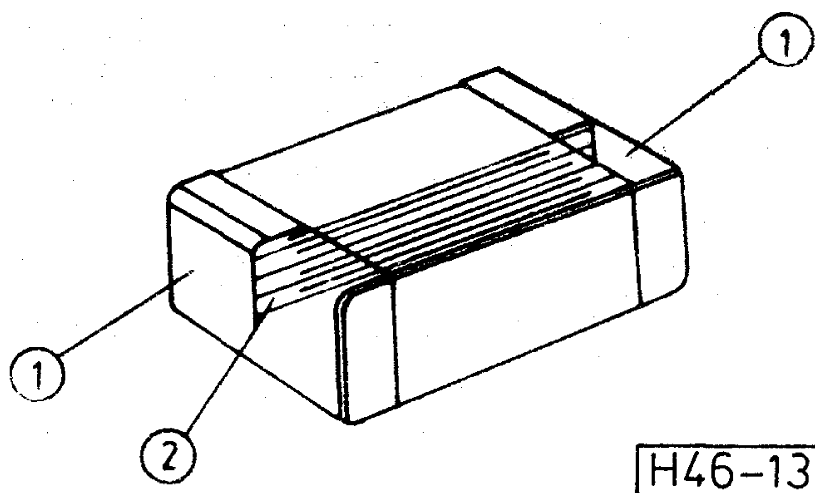
13. ábra. Kerámia monolit (chip) kondenzátor 1 — forraszfelület; 2 — kerámia-fólia dielektrikum és Pd-Ag fegyverzetek
