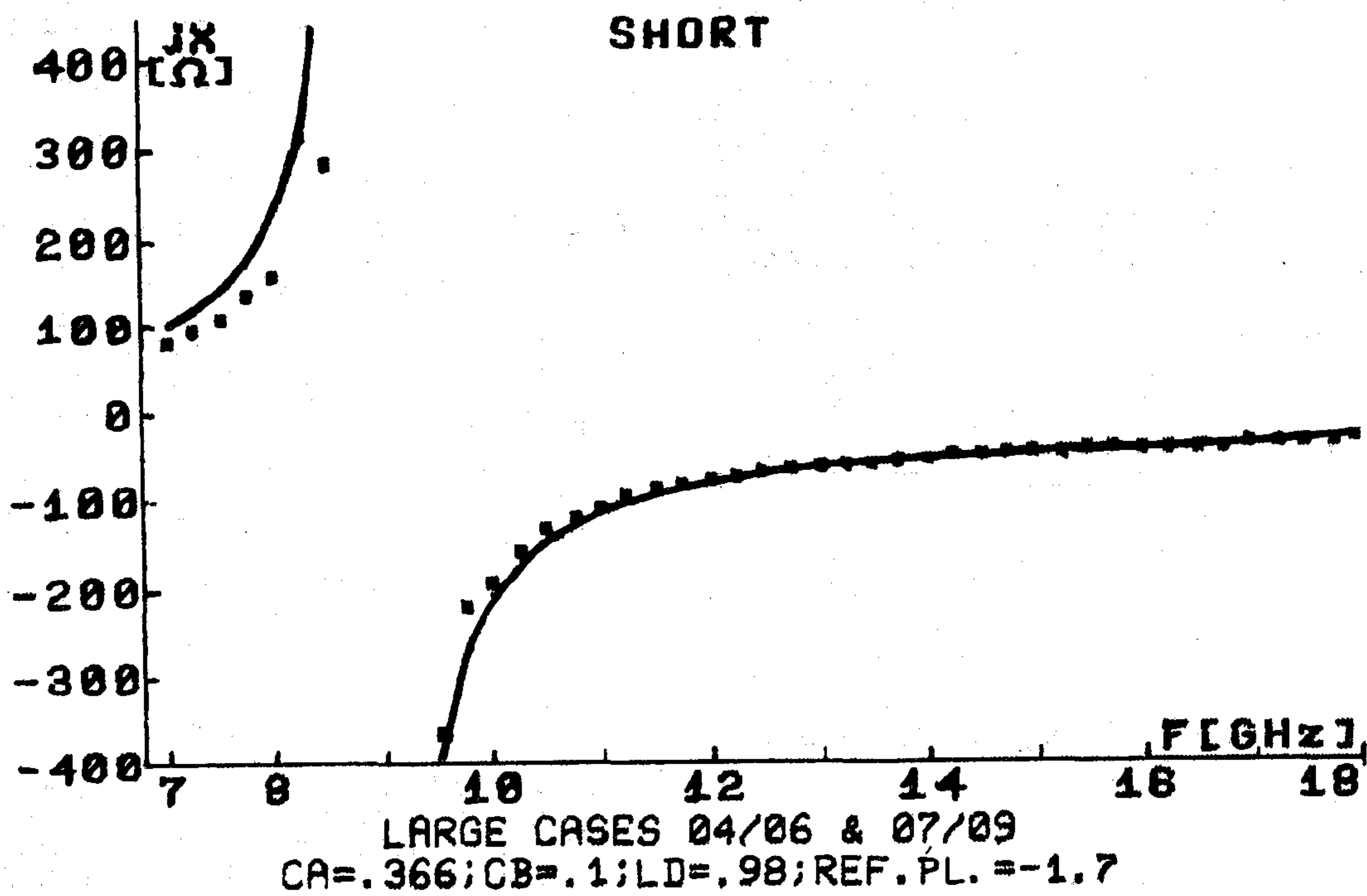
9. ábra. Menetes Gunn-tok impedanciájának frekvenciafüggése a chip helyén szakadósos (open) és rövidzáras (short) esetben. (Vonal: számított érték, csillag: mért érték)
