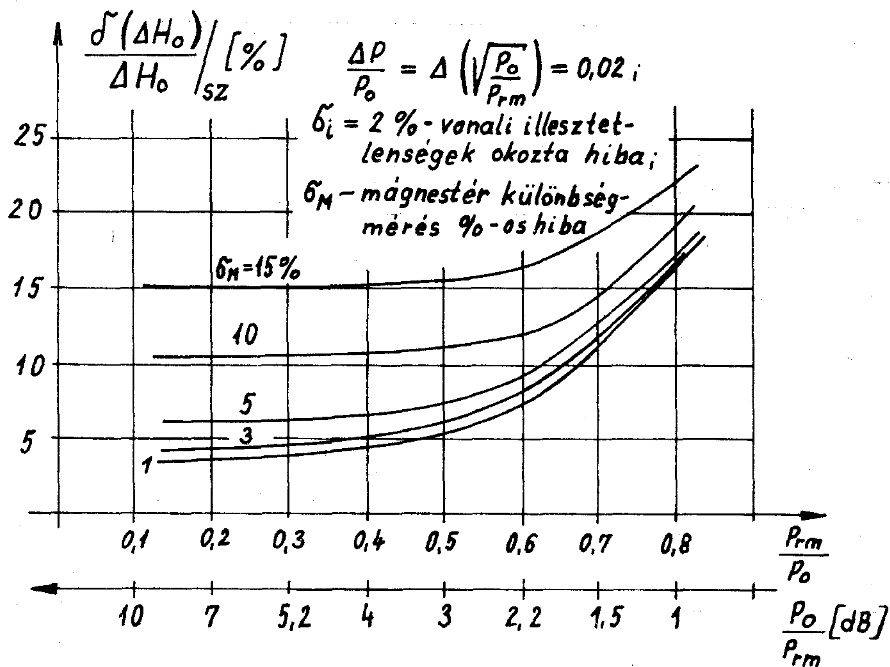
8. ábra. \Delta H_0 mérési pontosságának változása a P_{rm}/P_0 fv.-ében különböző relatív hibák esetén (illesztetlenségi hiba \sigma_i = 2\% , rel. teljesítmény ingadozás \Delta P/P_0 = 0,02 , mágnes tér-különbség mérési hiba \sigma_M, \% )
