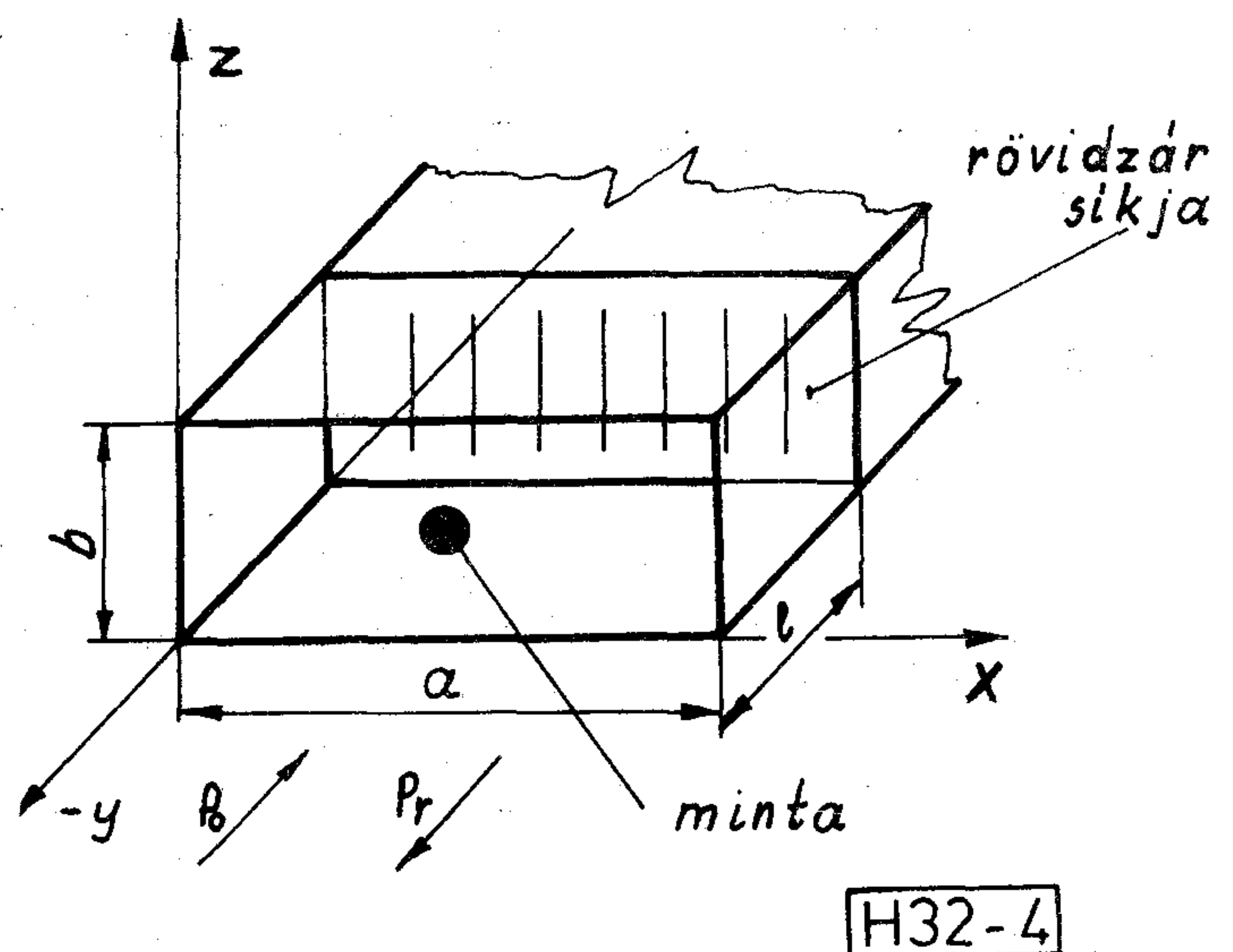
4. ábra. Rövidre zárt mérővonalba a behelyezett mintával
