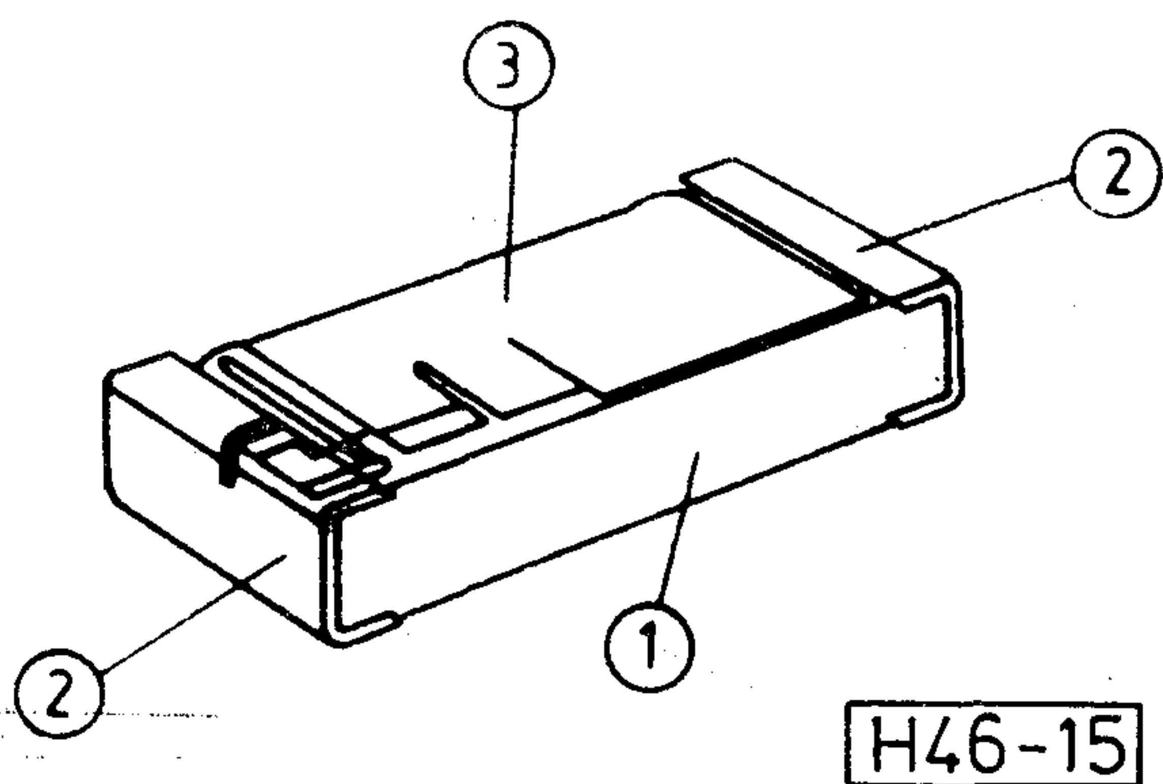
15. ábra. Sík (chip, vastagréteg) ellenállás 1 — \text{Al}_2\text{O}_3 hordozó; 2 — forraszfelületek; 3 — ellenállás réteg
