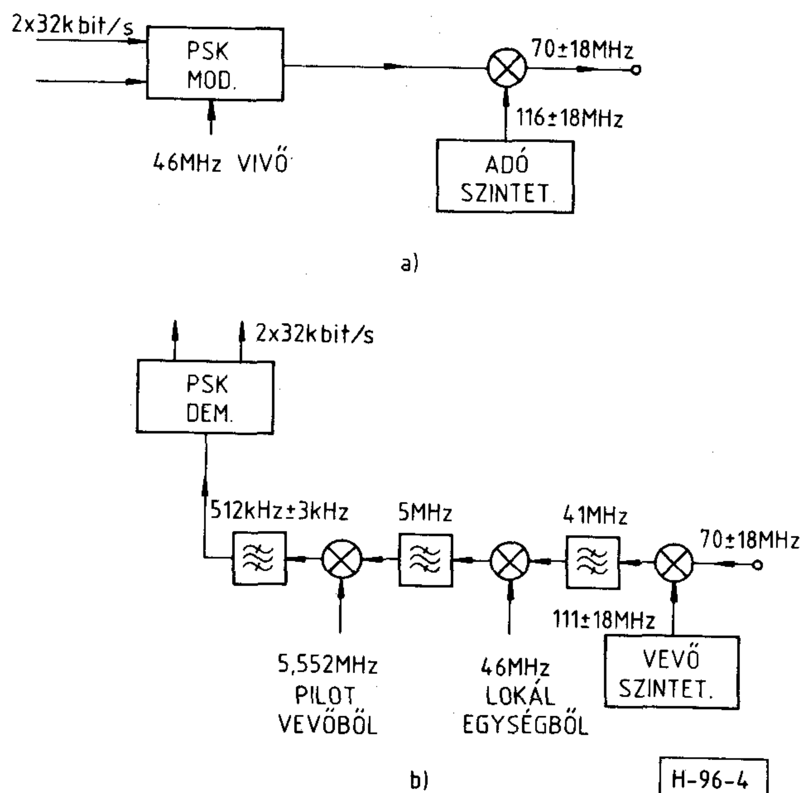
4. ábra. A PSK egység felépítése. a) PSK adó, b) PSK vevő
