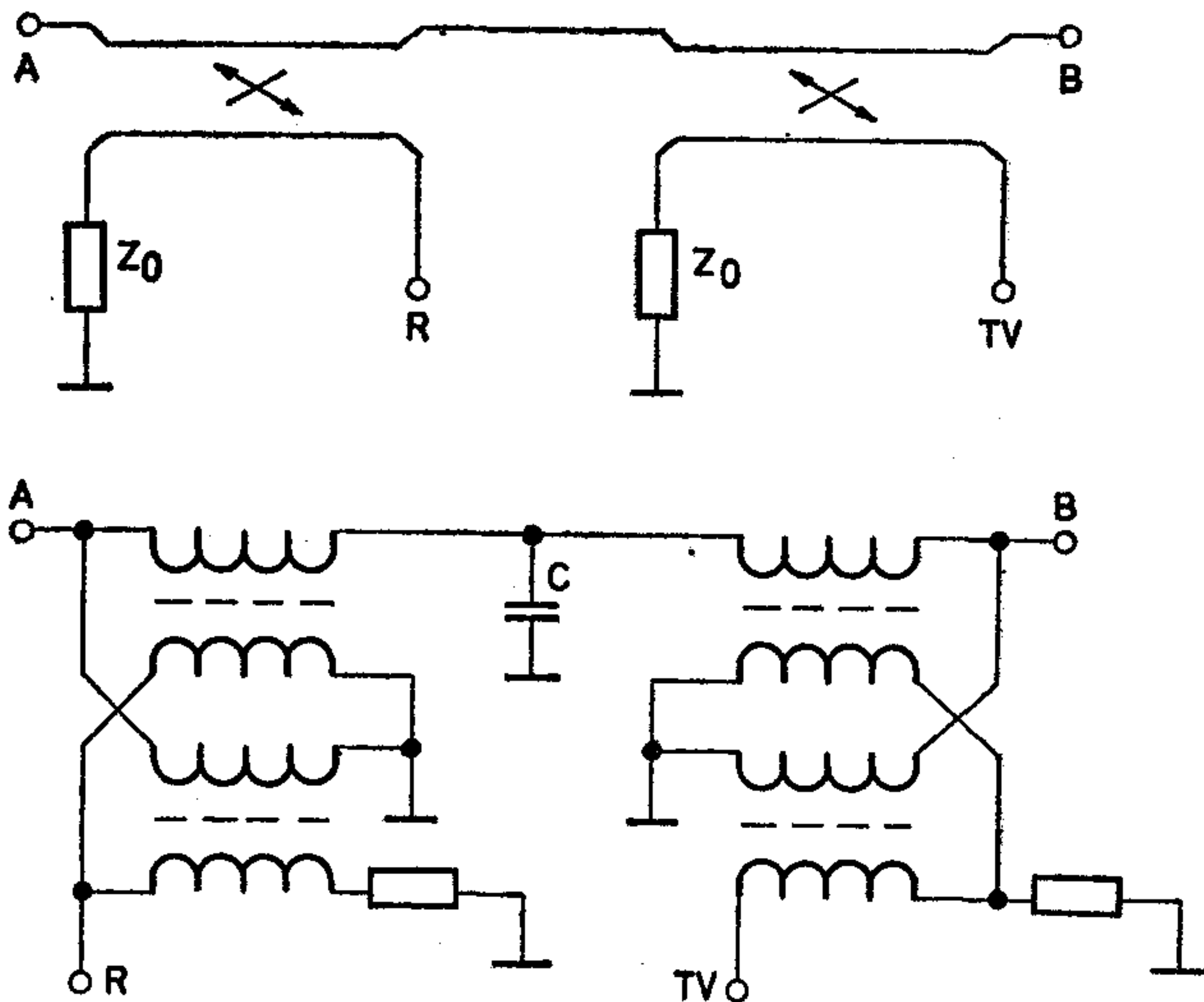
5. ábra Kettős iránycsatoló és megvalósítása
