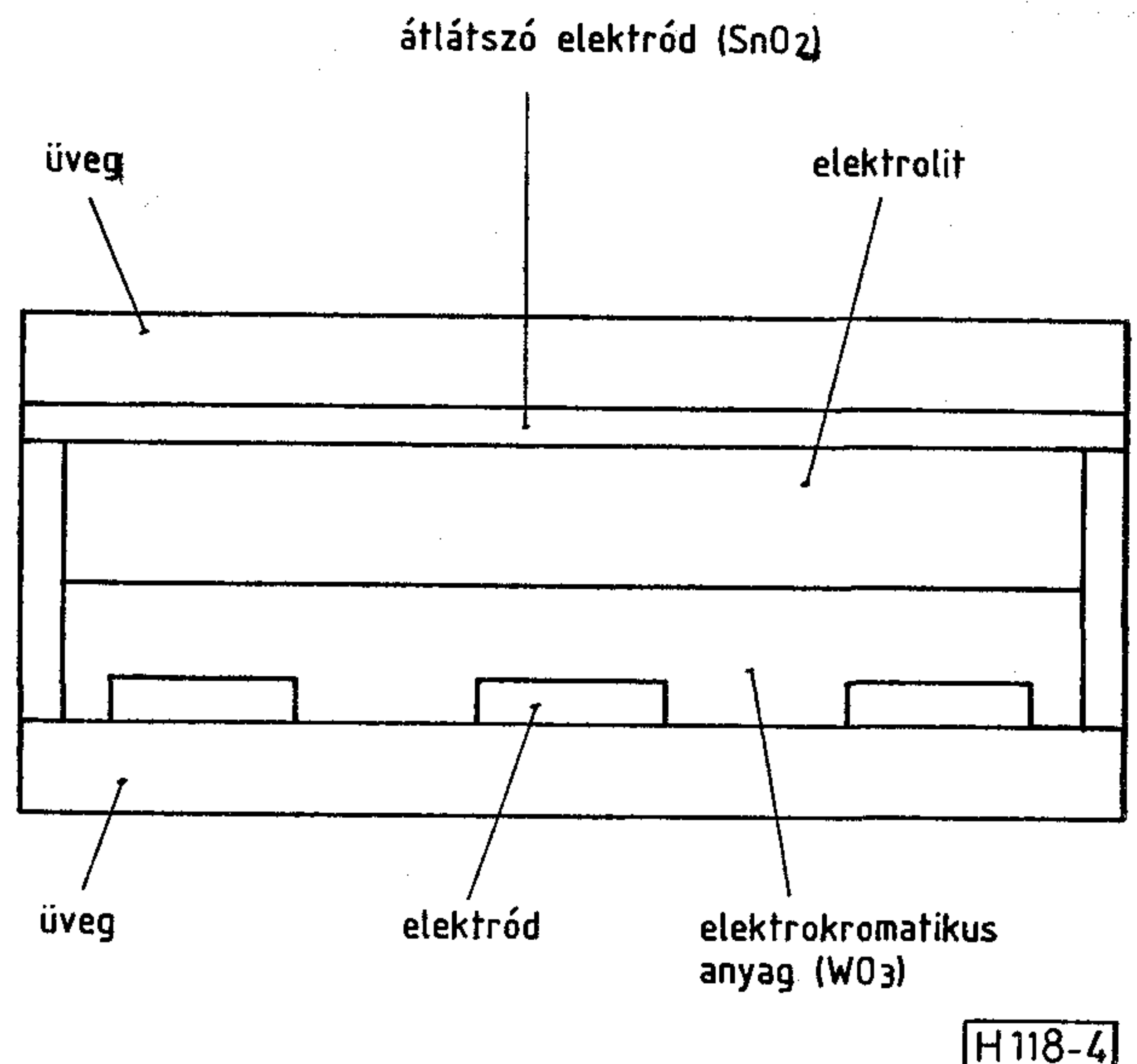
4. ábra. Az elektrokromatikus kijelző felépítése
