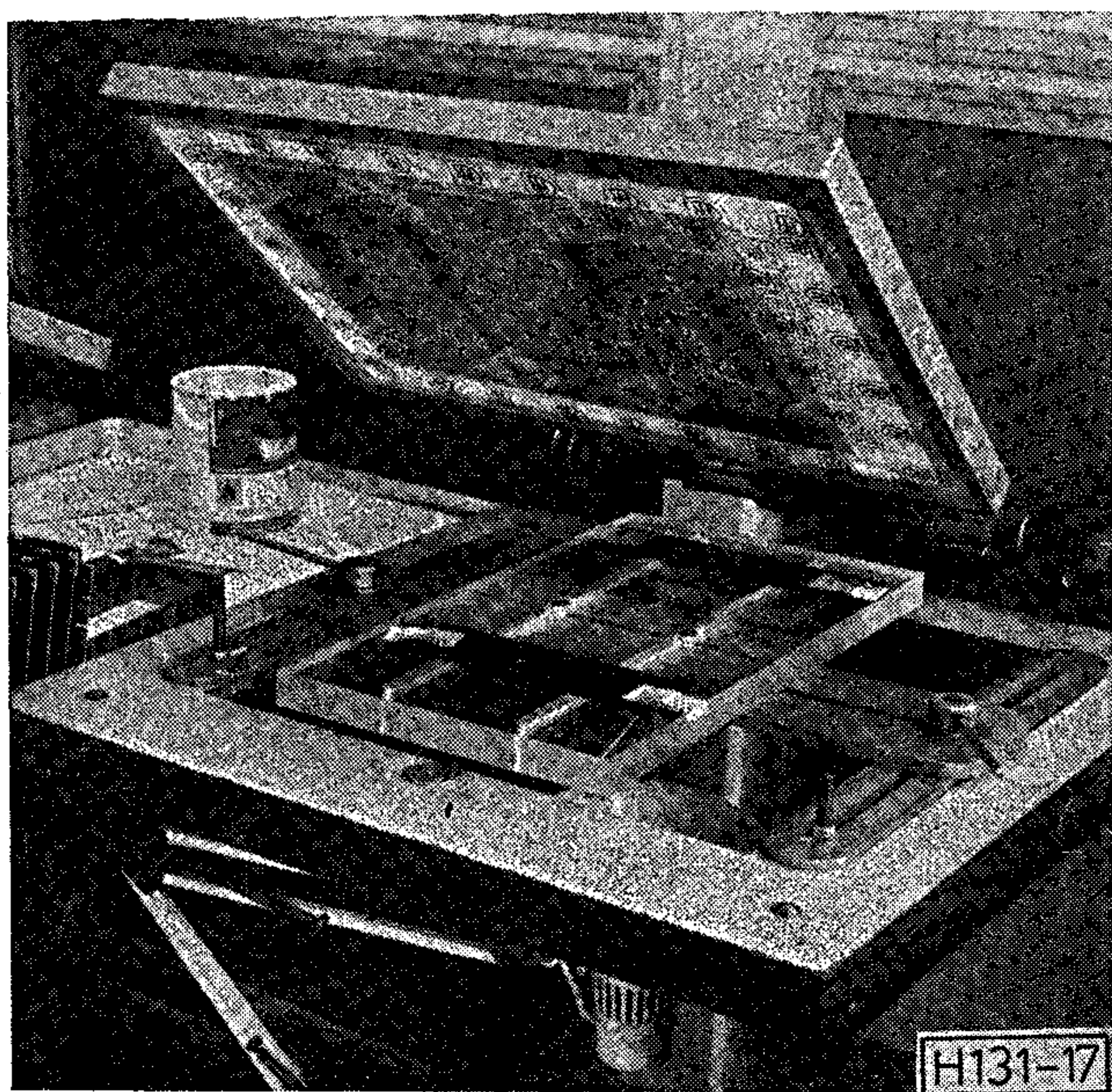
17. ábra. Kézi szitanyomó munkahely durva beállításának elemei
