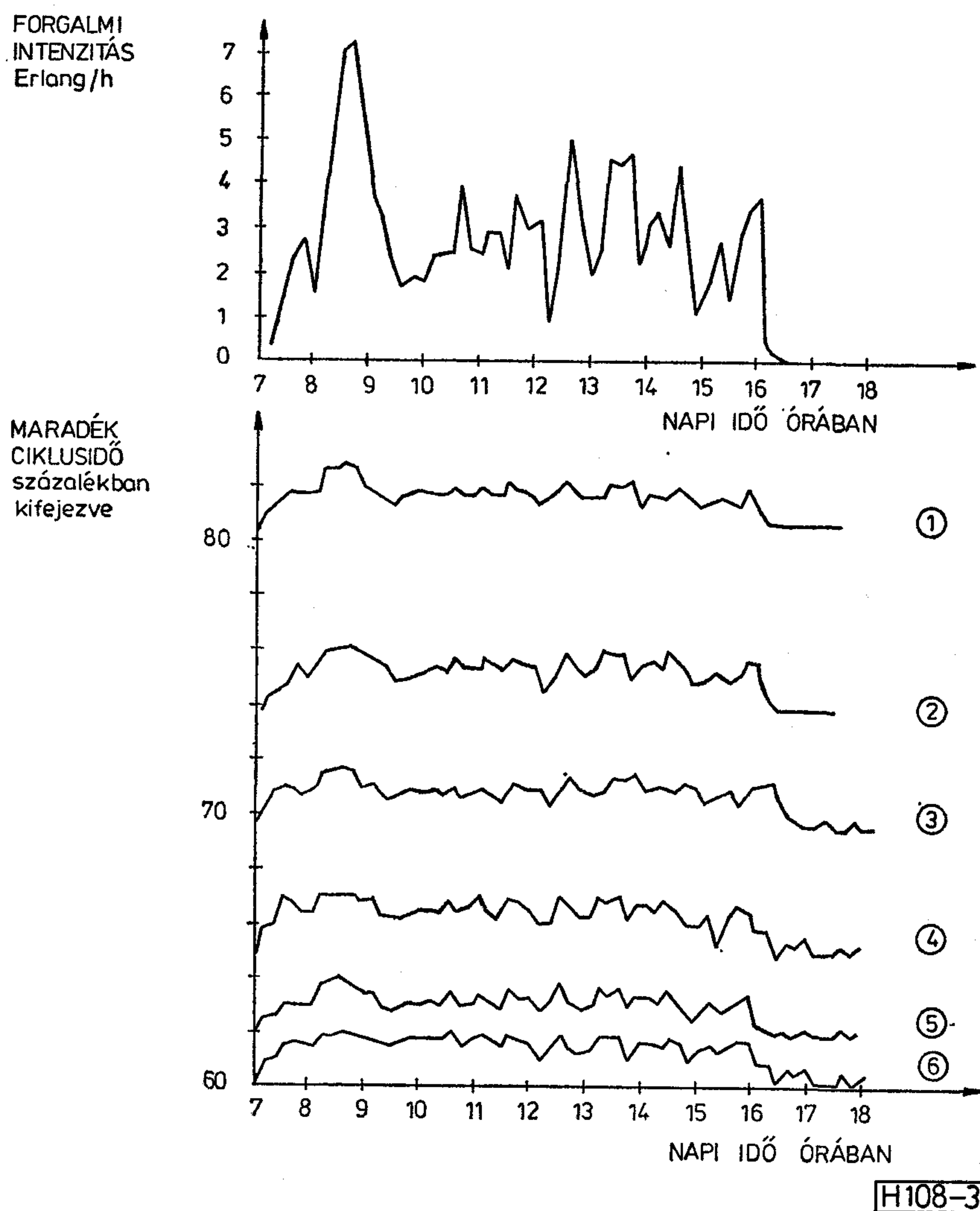
3. ábra. A processzor maradék idejének alakulása a forgalmi intenzitással összevetve. Az ábra számjelzései magyarázata:
