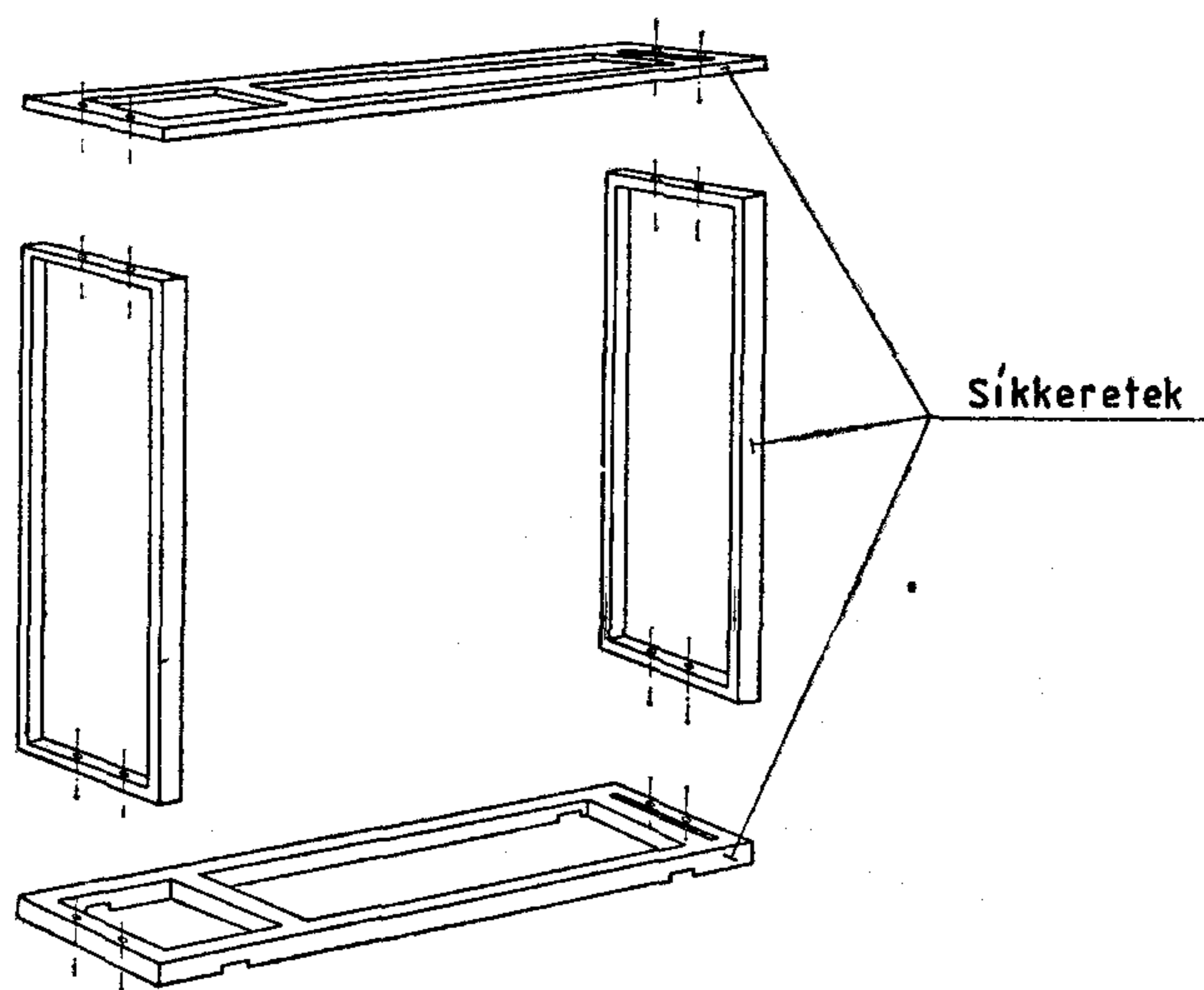
2. ábra. Szekrényváz
