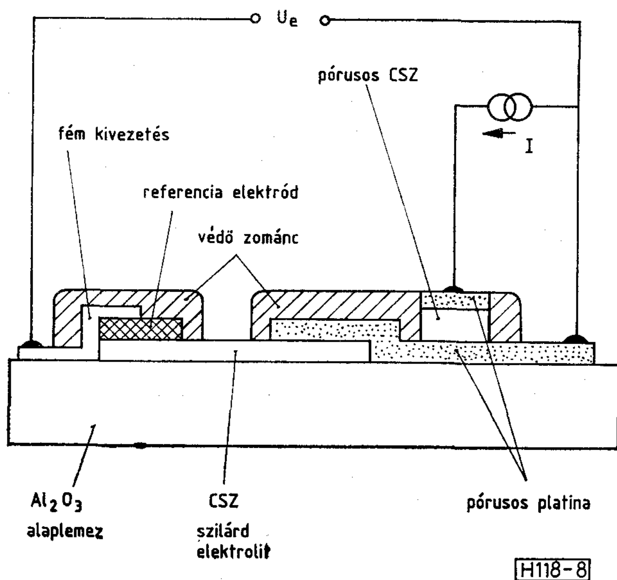
8. ábra. \lambda -szenzor felépítése
