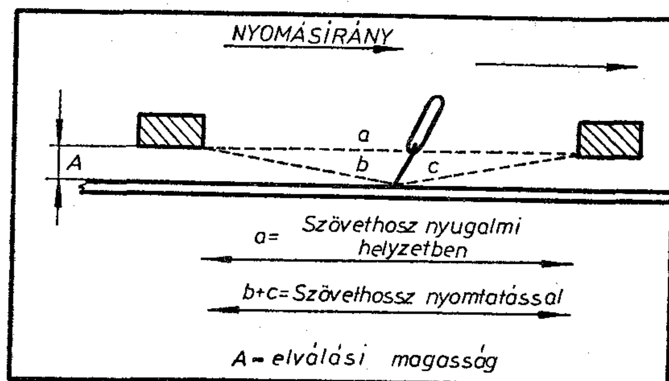
20. ábra. Nyomtatás hatására létrejövő méretváltozás
