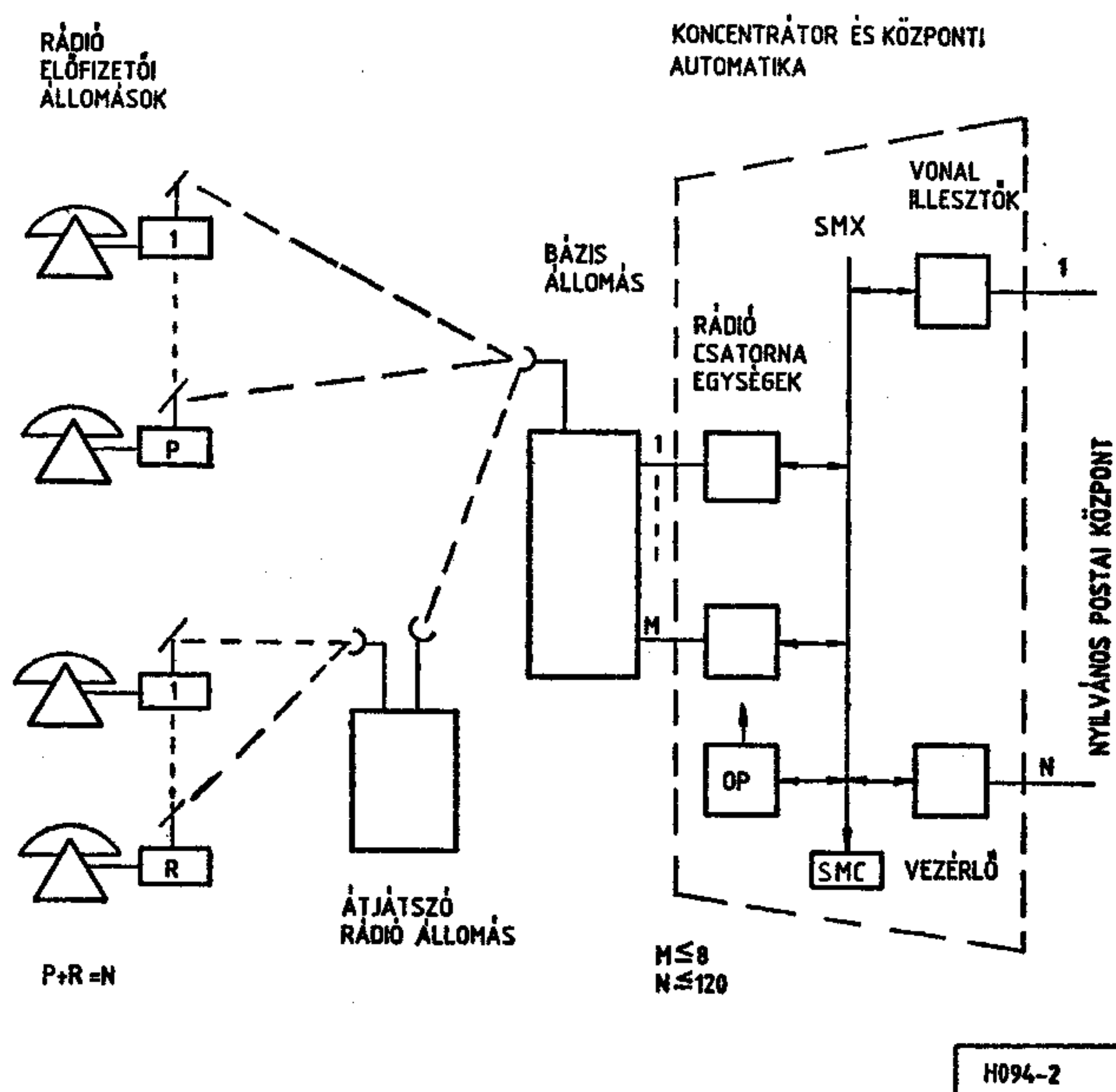
2. ábra. URH hírendszer (CLS) felépítése
