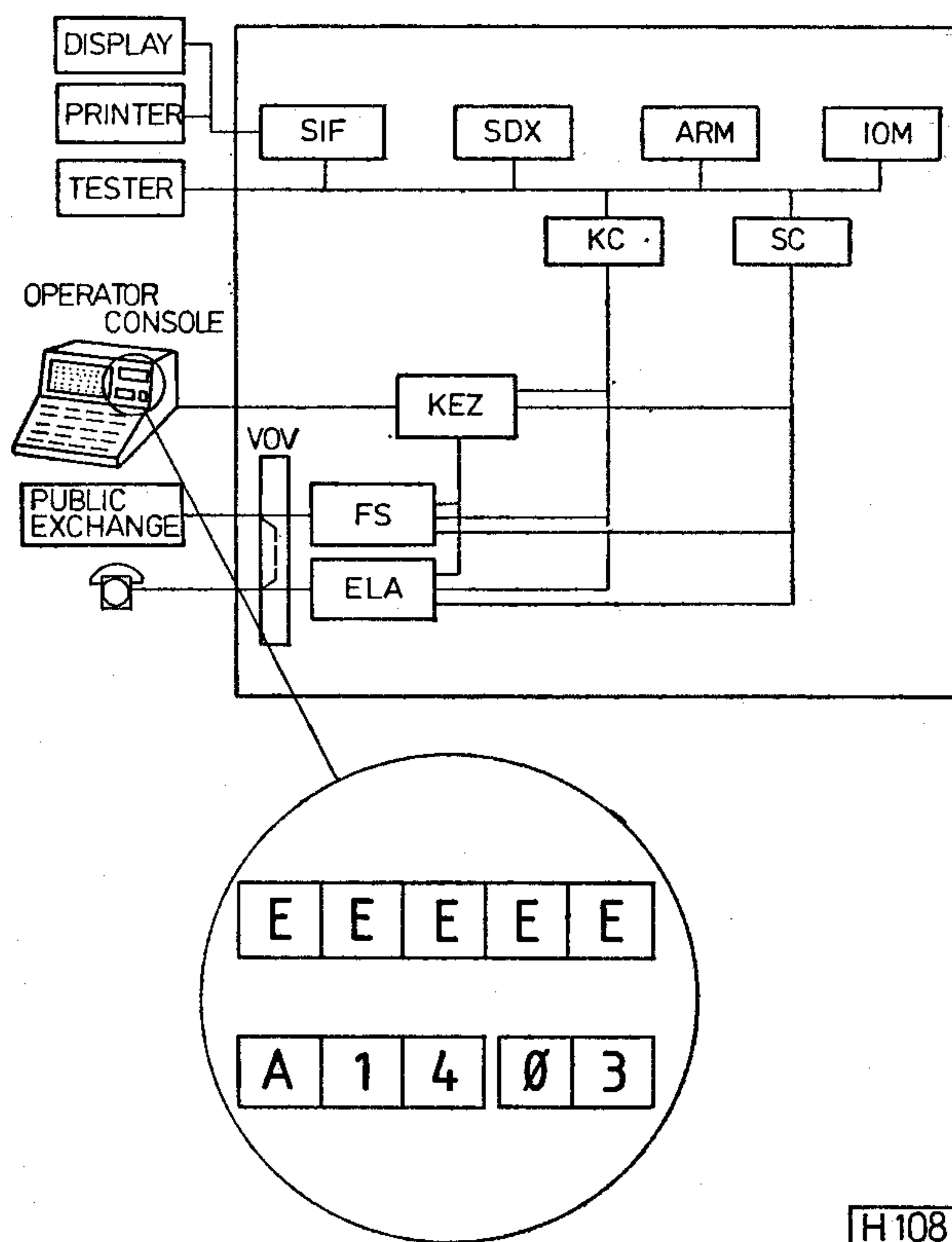
1. ábra. DIPEX 50 digitális alközpont blokkdiagramja periferiákkal együtt. Az ábra jelöléseinek magyarázata:
