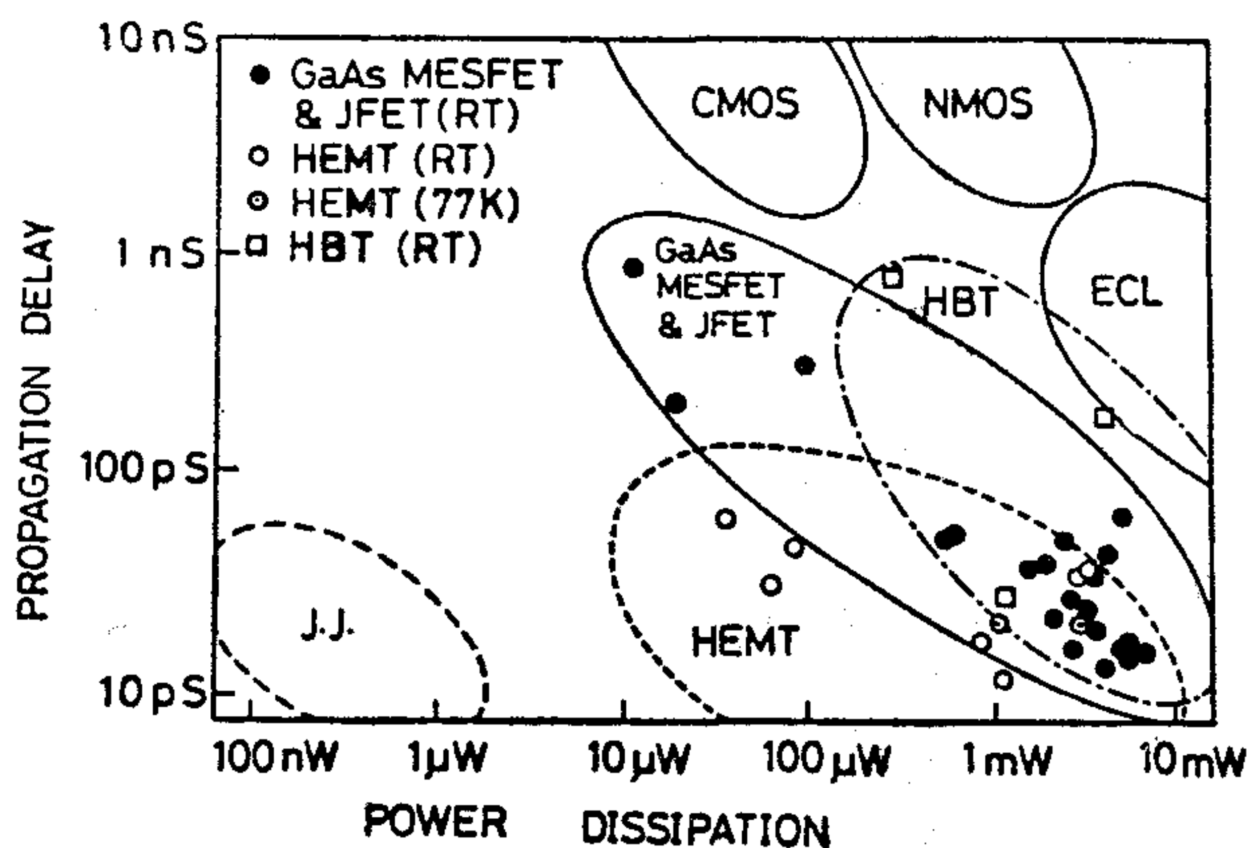
1. ábra. A Fujitsu Laboratories növekményes/kiürítéses nagy elektron mozgékonyaságú tranzistorának (HEMT) szerkezete az LSI áramkörökben és a HEMT logika a kapunkénti késleltetési idő — teljesítmény disszipáció grafikonon ábrázolt összehasonlításban szobahőmérsékleten (RT) és cseppfolyós nitrogén hőmérsékleten (77K)
