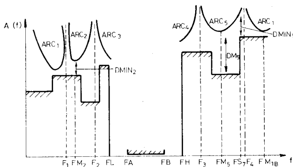
3. ábra. Sáváteresztő szűrő specifikációja, s annak zárósávbeli közelítése
