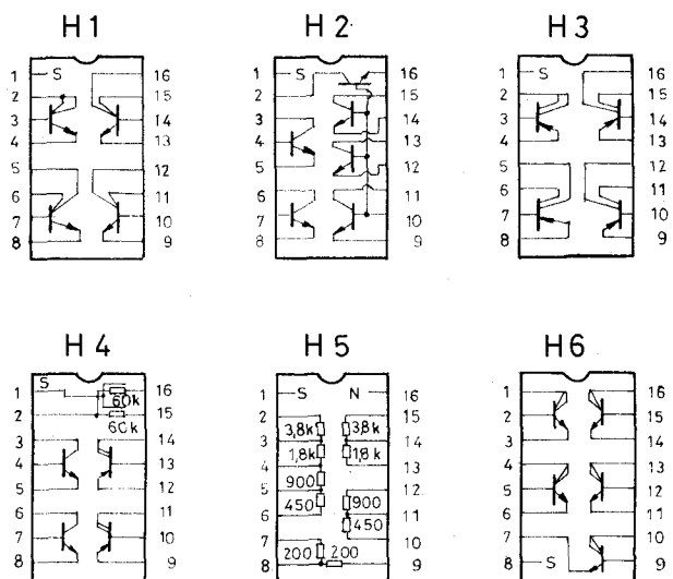
2. ábra. A LIDI-kit elemeinek bekötése
