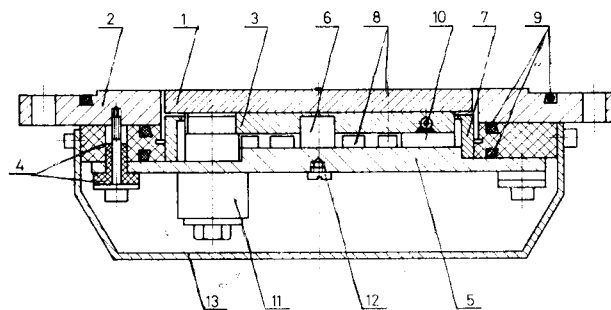
4. ábra. A PENTRON katódporlasztók felépítése (kamrafalra szerelhető változat). 1 — target; 2 — anód; 3 — hűtő; 4 — szigetelő; 5 — alaplap; 6 — főmágnes; 7 — pólus; 8 — segédma-gnesek; 9 — „0”-gyűrűs tömítés; 10 — hűtővízesatorna; 11 — hűtővízbevezető; 12 — villamos csatlakozó; 13 — burkolat
