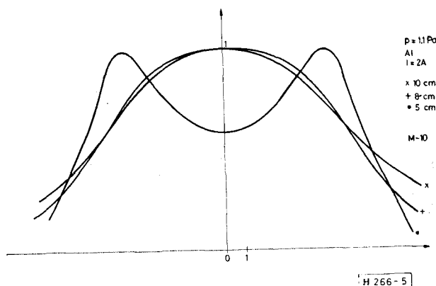
5. ábra. Különböző target-szubsztrát távolságoknál felvett rétegvastagság-eloszlás görbék
