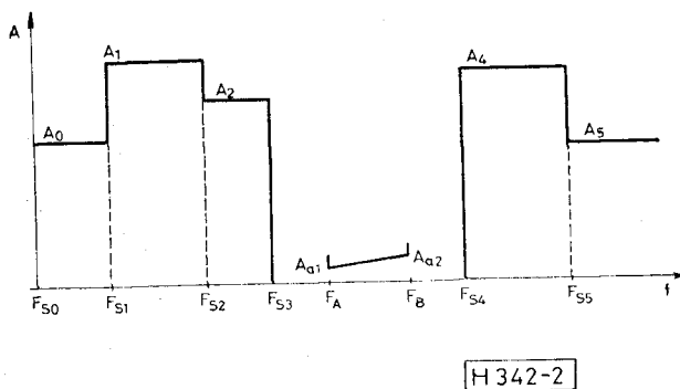
2. ábra. Általános csillapításkarakterisztika zárósávi lépcsőkkel
