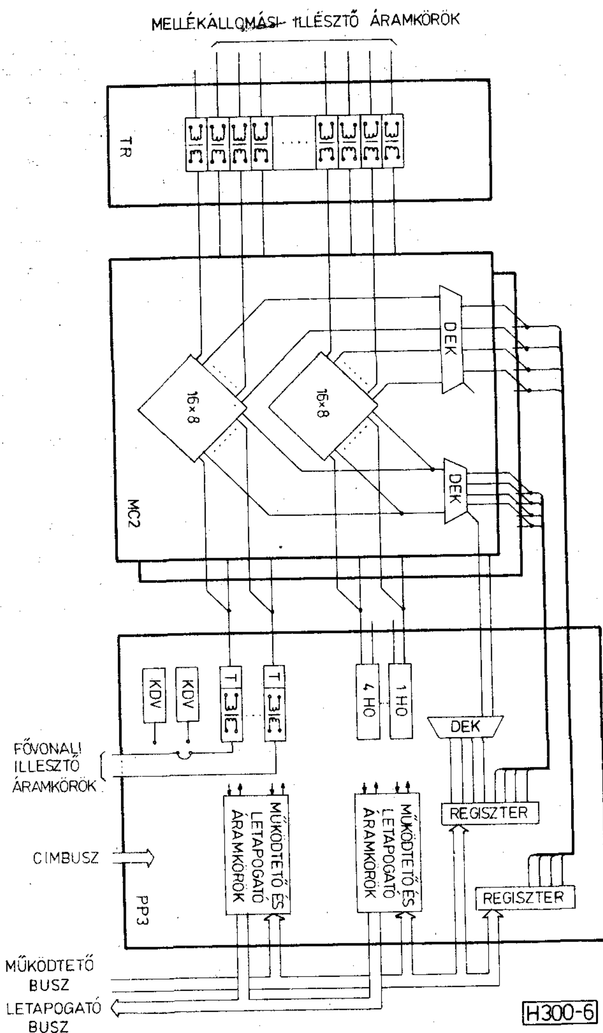
6. ábra. Az EP32M kapcsolómezőjének fizikai realizálása
