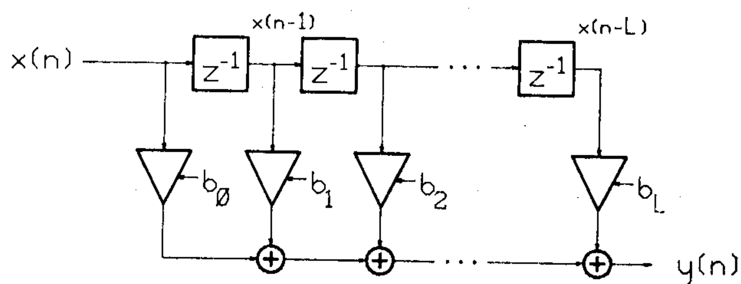
12. ábra. FIR szűrő
