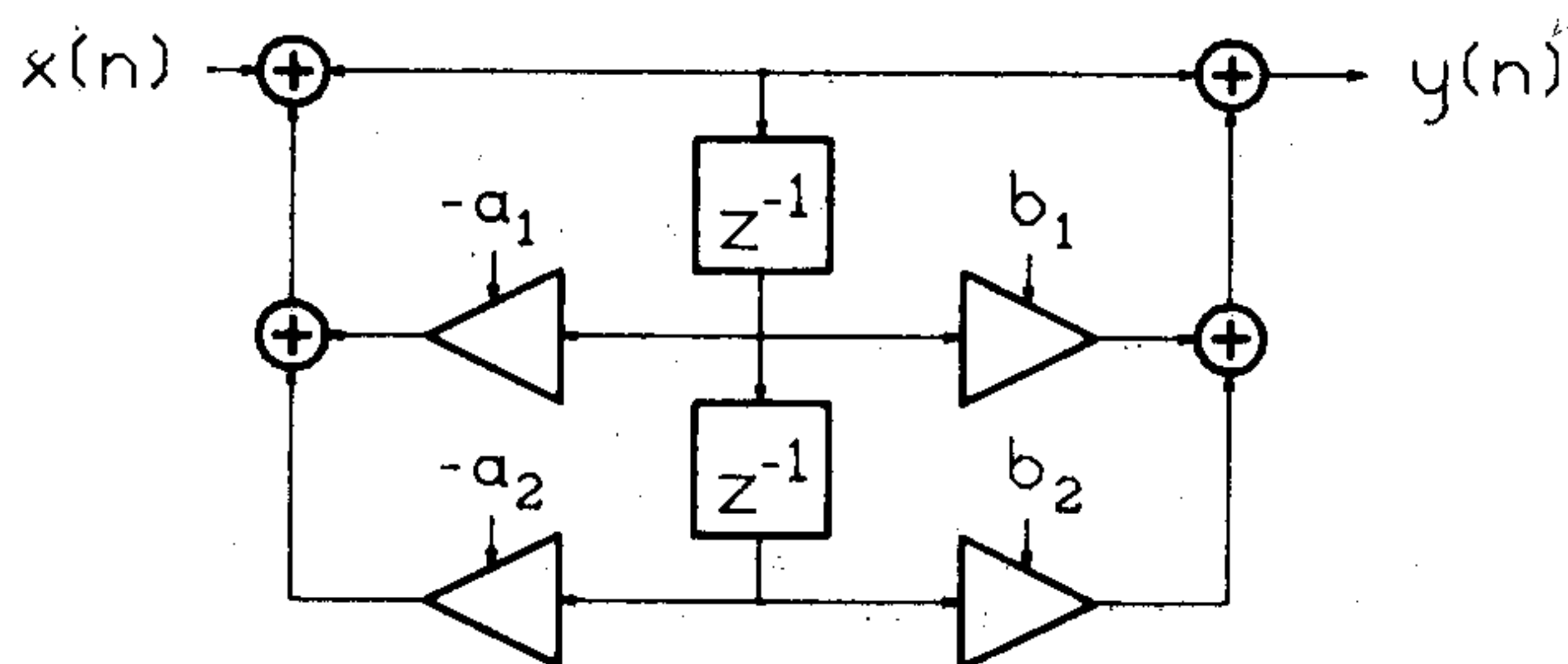
13. ábra. Csőmodelles FIR szűrő
