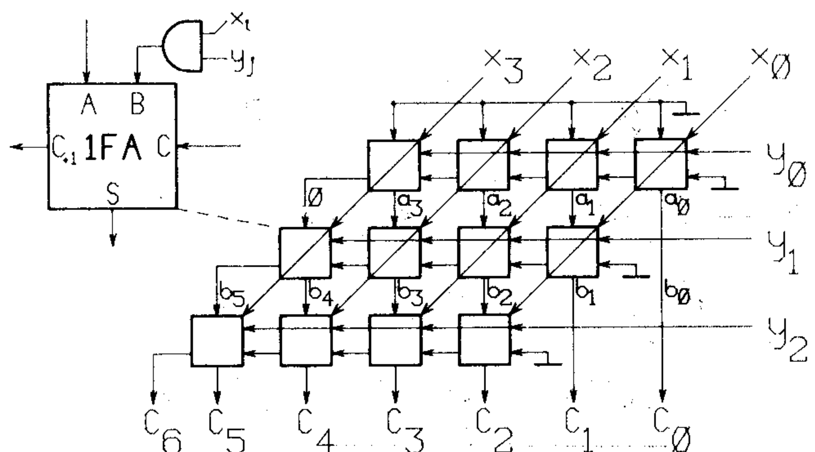
1. ábra. Párhuzamos szorzó
