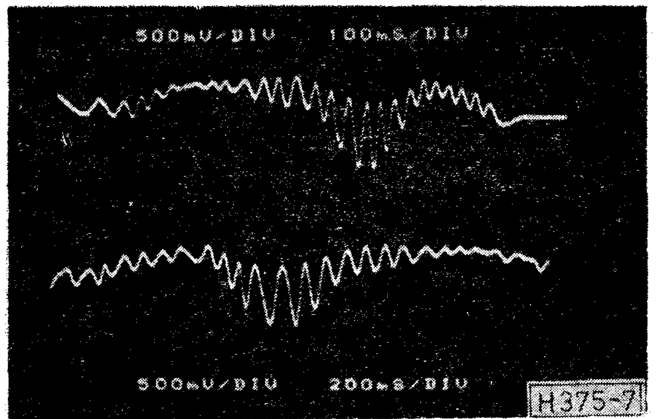
7. ábra. Diffúz felületű alumínium lemez translációs mozgásának vizsgálatakor kapott jelek; a test sebessége a mm/sec nagyságrendbe esett.
