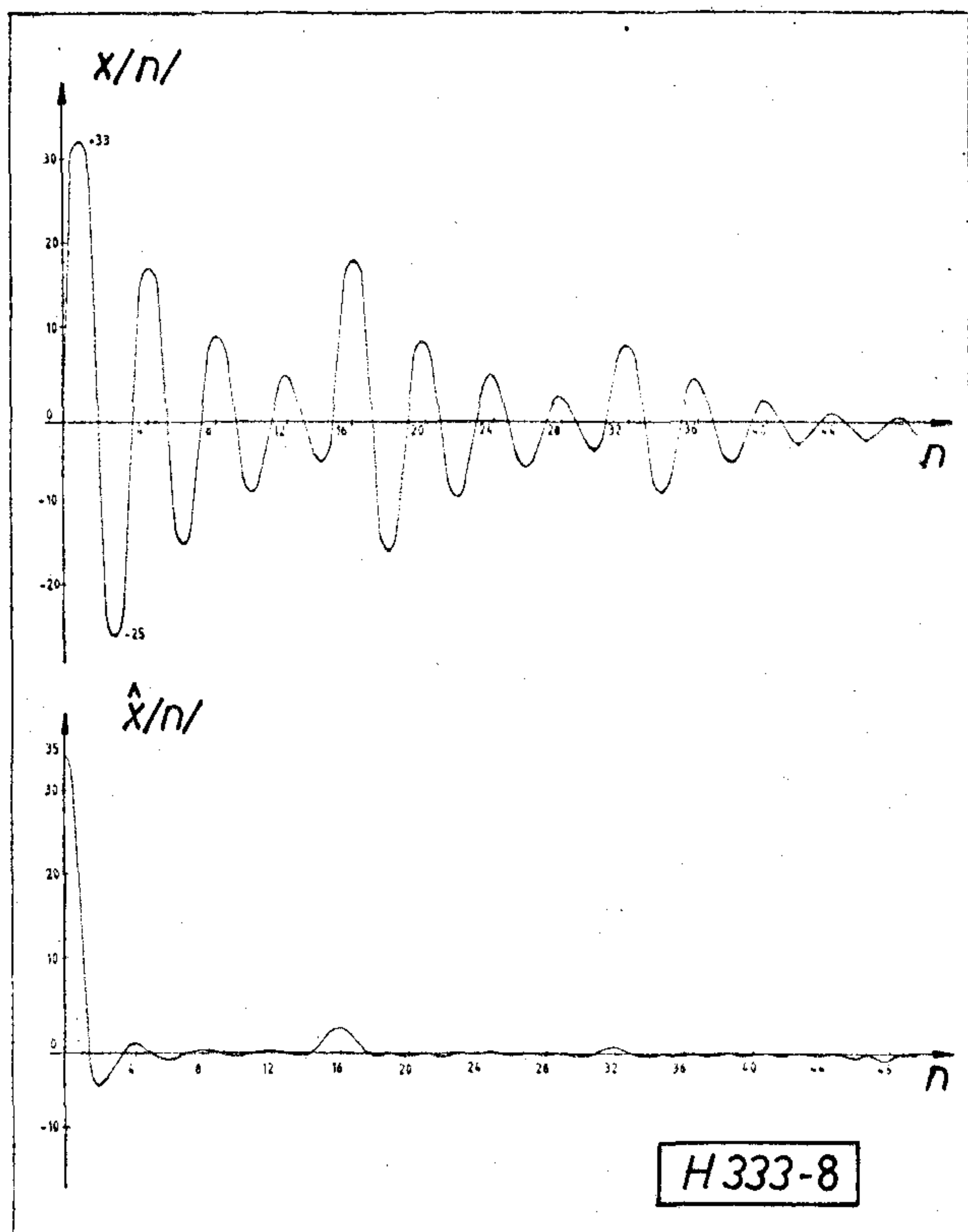
8. ábra. Lecsengő sinus-jel és kepsztuma
