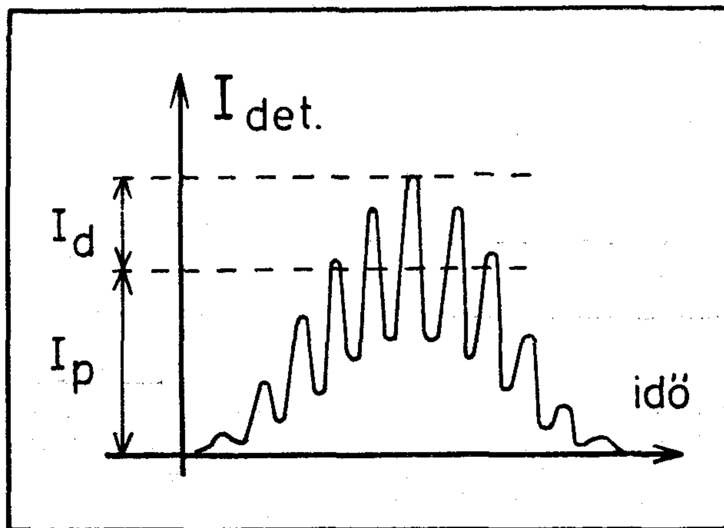
2. ábra. A differenciál lézer doppler anemométerek működési elvének modellje
