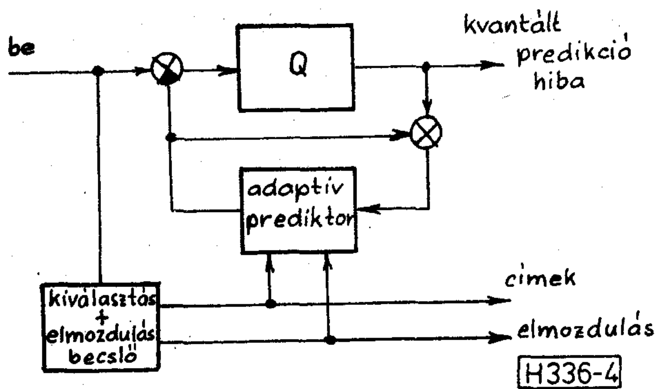
4. ábra. Blokk-illesztő mozgás-kompenzált DPCM kódoló
