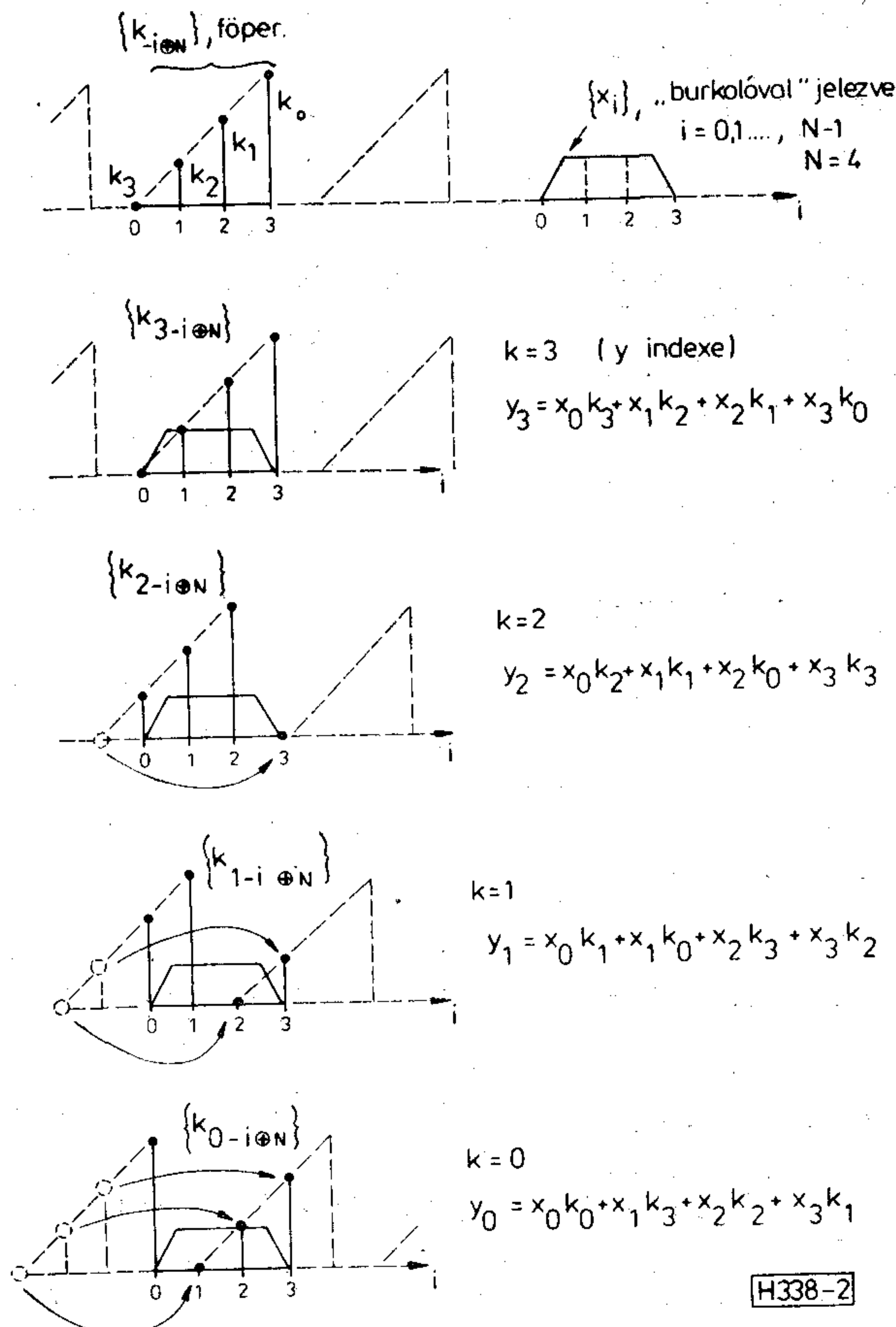
2. ábra. Diszkrét konvolúció a főperiódusok indexeivel. Jelölés +N = „\text{modulo } N” összegezés
