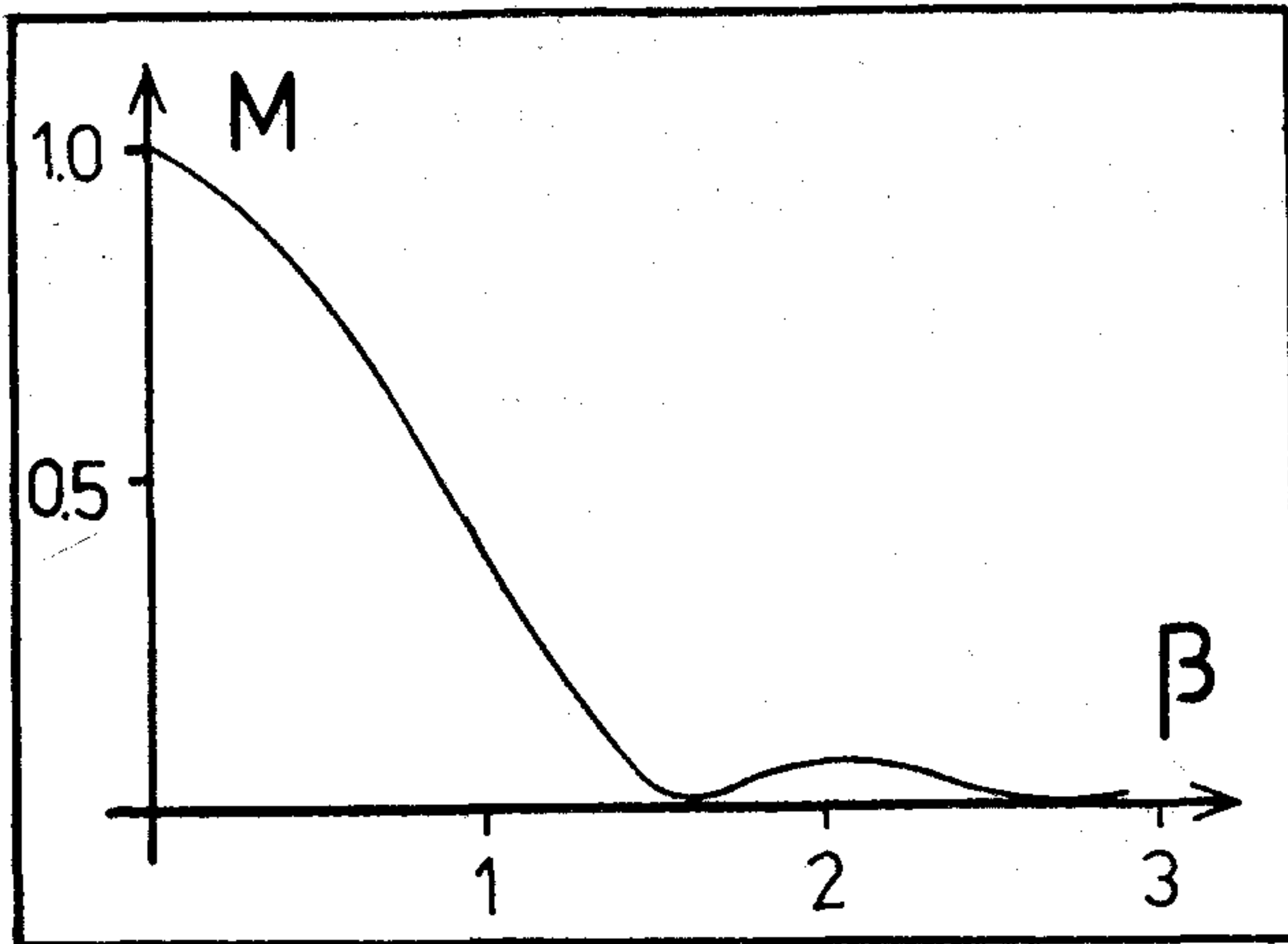
5. ábra. A detektor kimenőjelének modulációs mélysége a \beta paraméter függvényében. (Gömb alakú részecskék, és a fényhullámhosszhoz képest igen nagy detektor apertúra feltételezésével; [2] alapján.)
