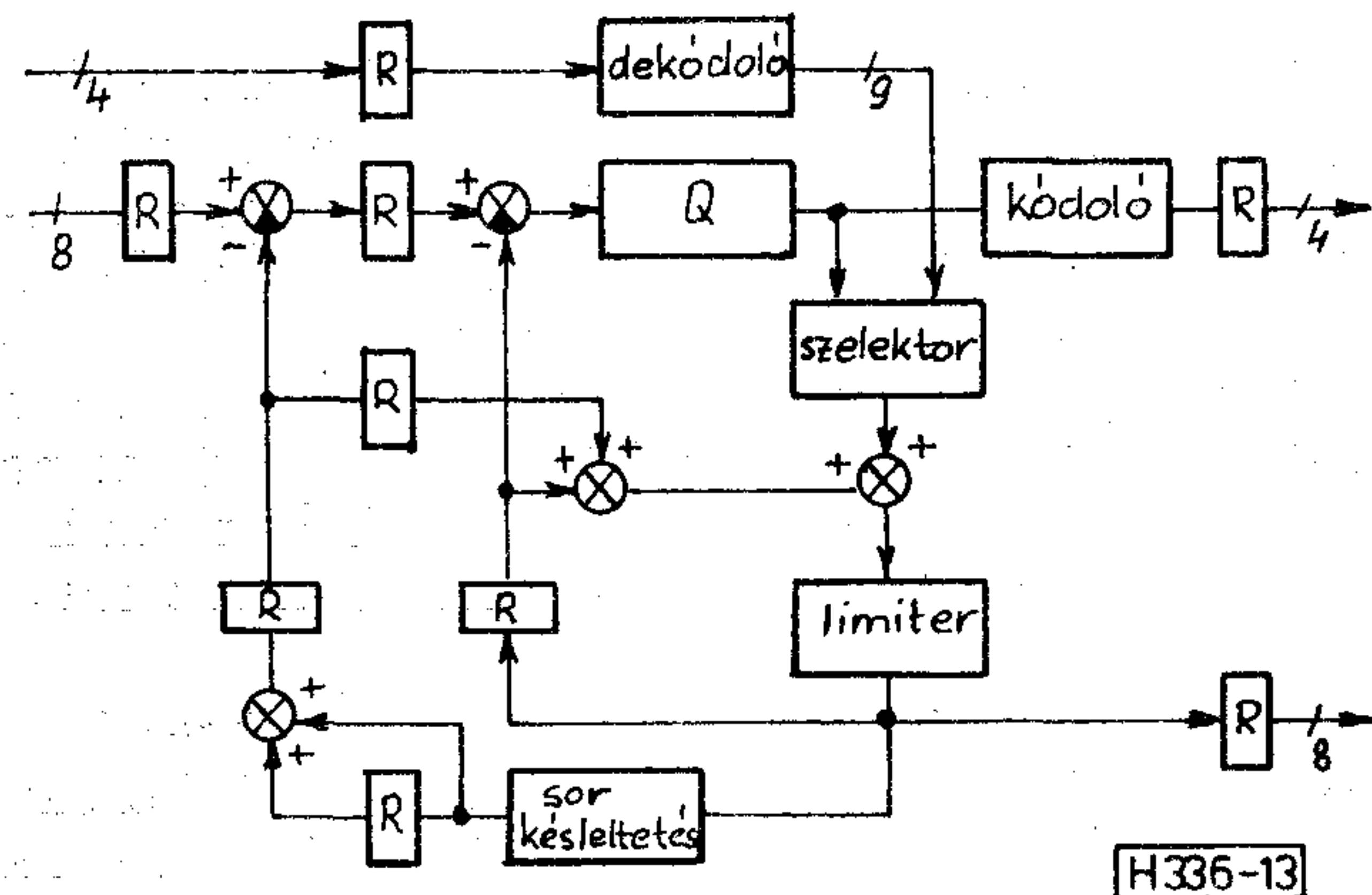
13. ábra. DPCM kodek blokkvázlata
