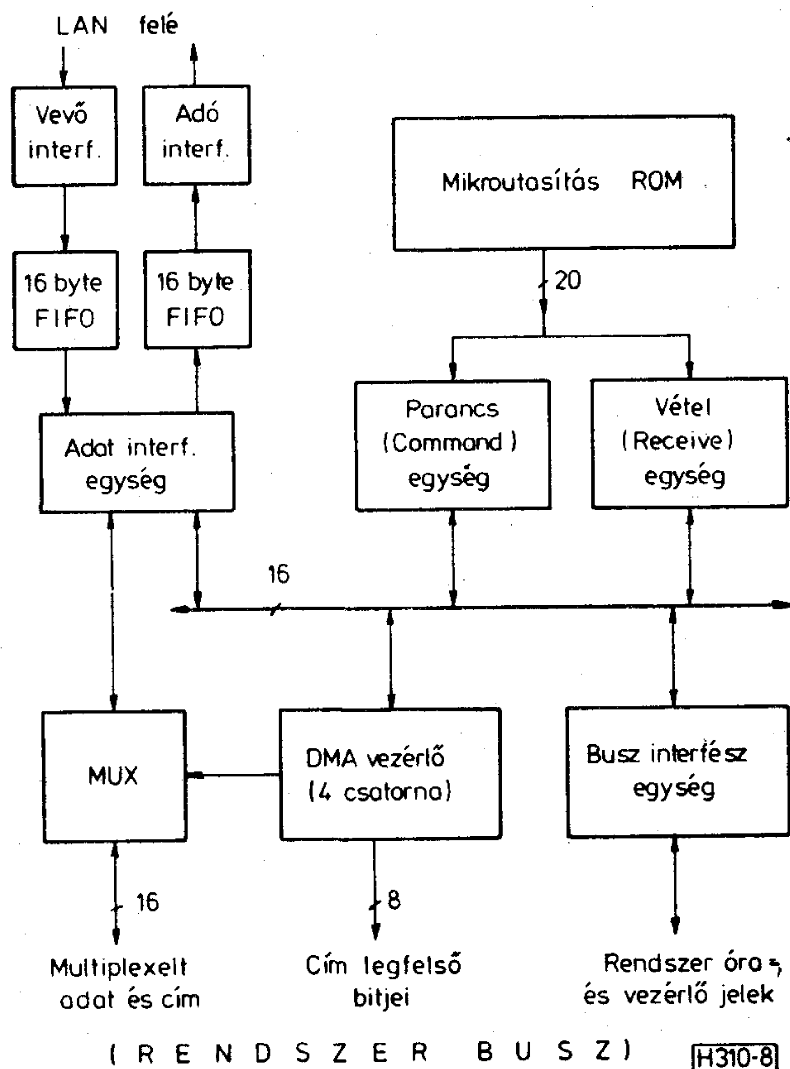
8. ábra. Az Intel 82586 társprocesszor tömbvázlata
