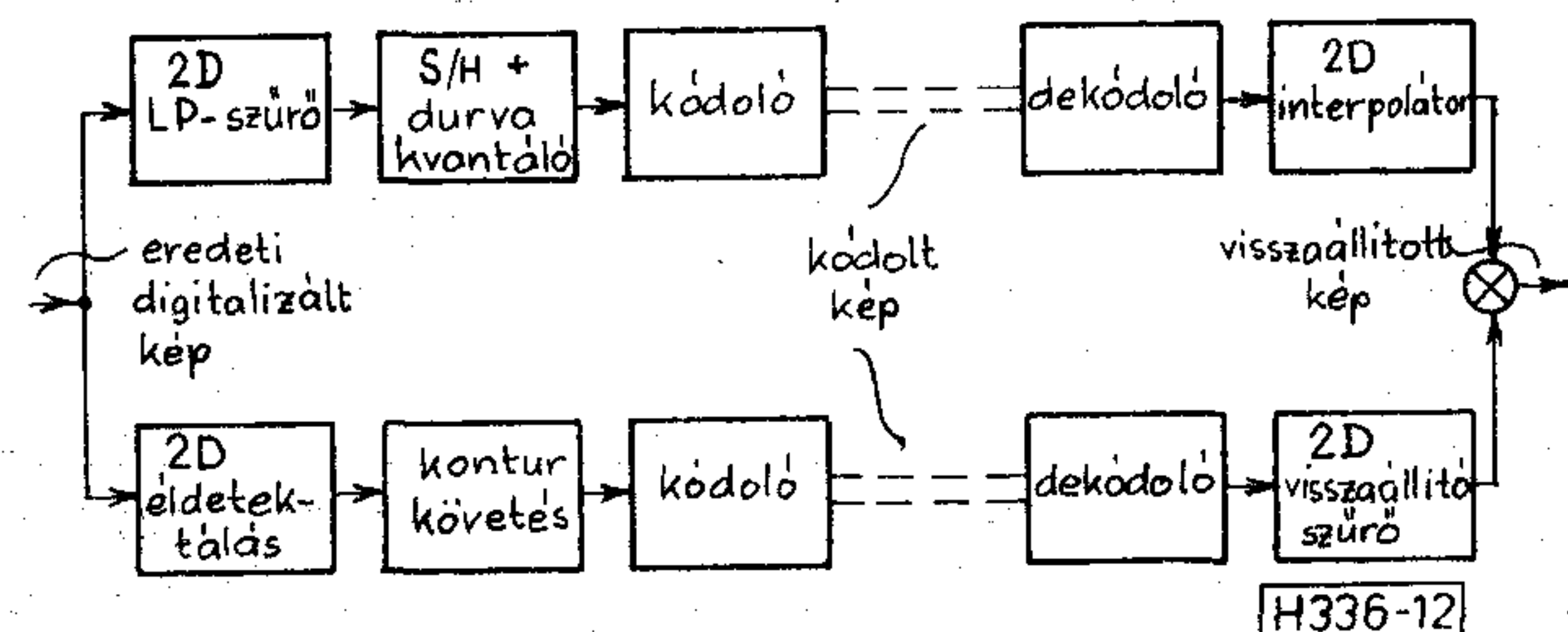
12. ábra. „Synthetic High” rendszer blokkvázlata
