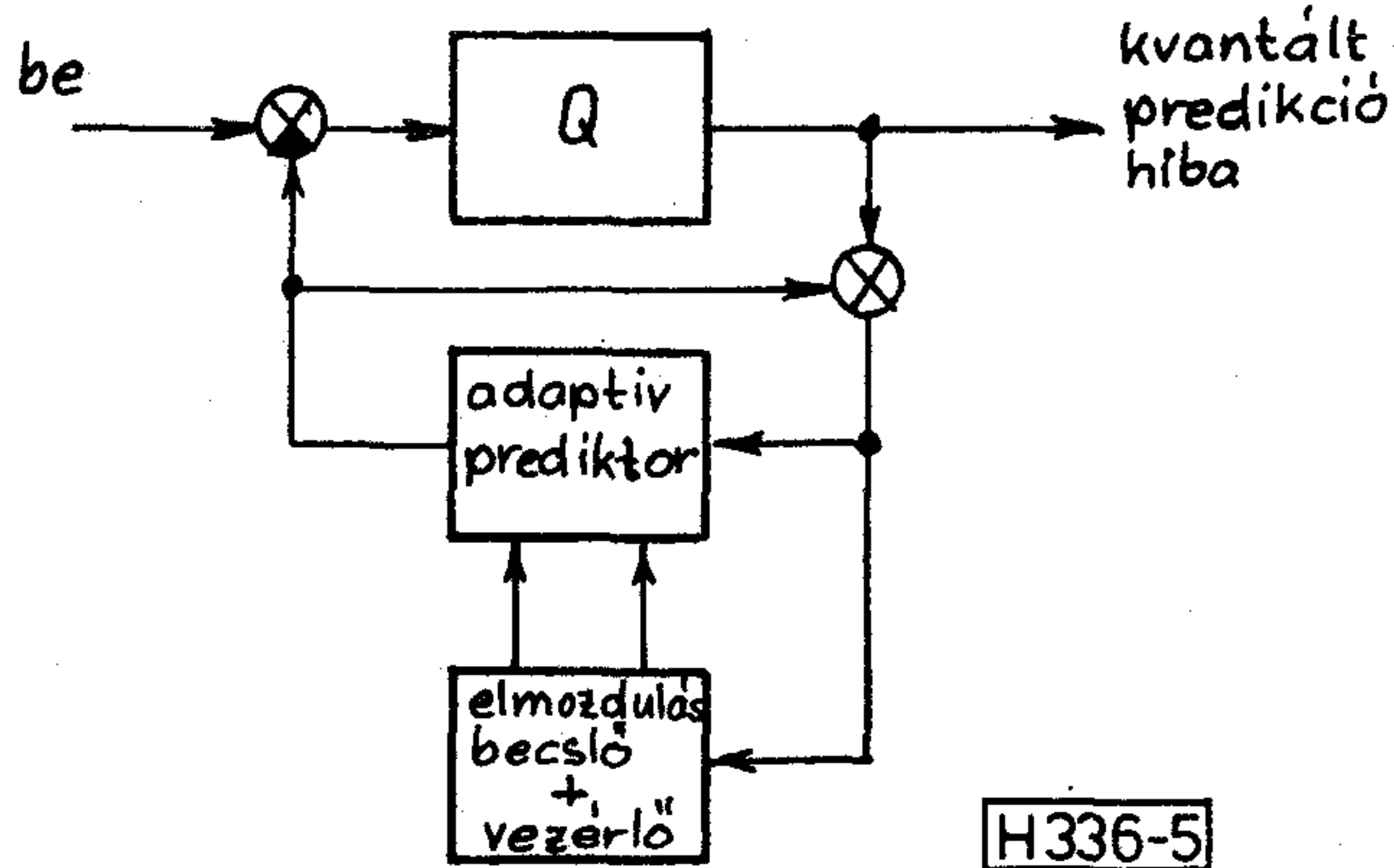
5. ábra. Rekurzív mozgás-kompenzált DPCM kódoló
