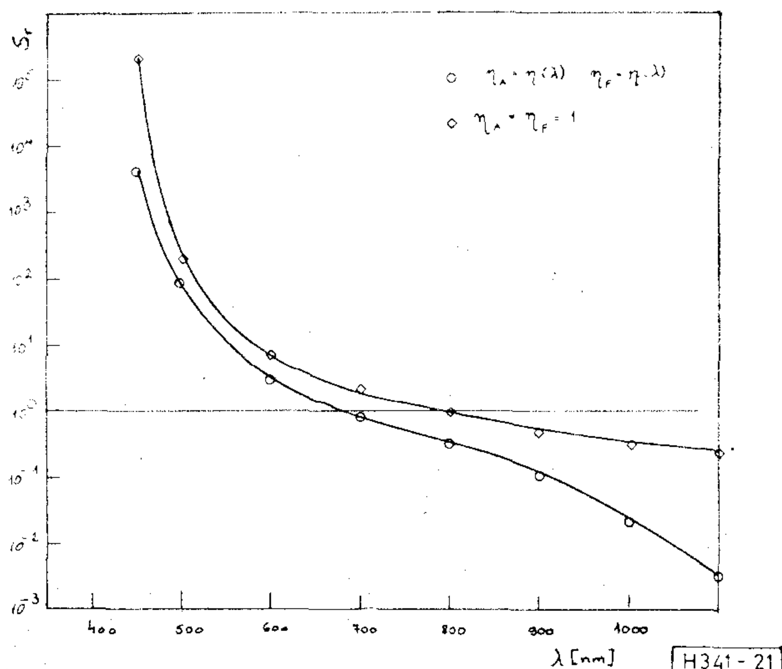
21. ábra. Spektrális karakterisztika \eta=1 illetve \eta=\eta(\lambda) figyelembevételével
