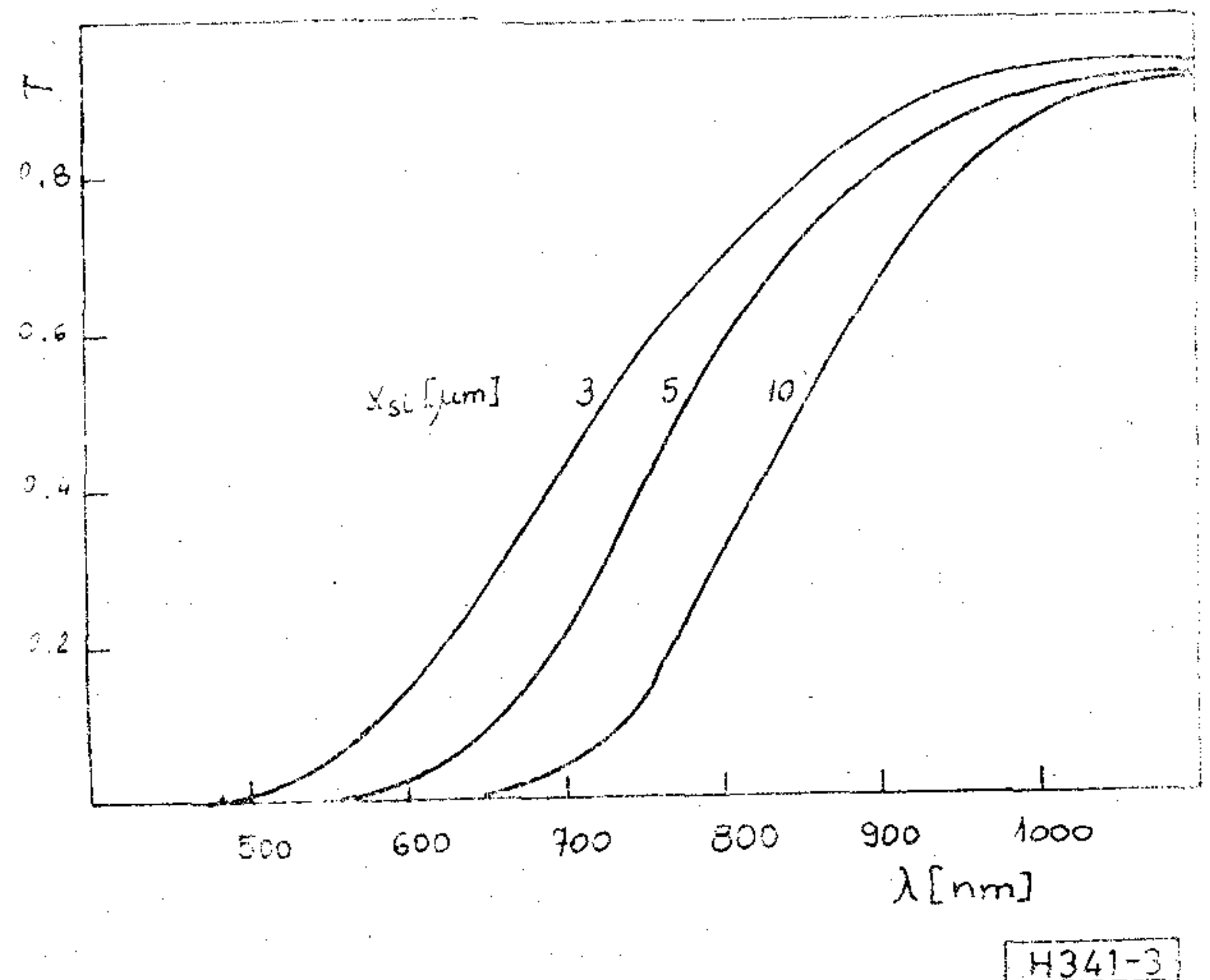
3. ábra. 150 nm vastag oxidréteggel borított Si réteg transzmissziója
