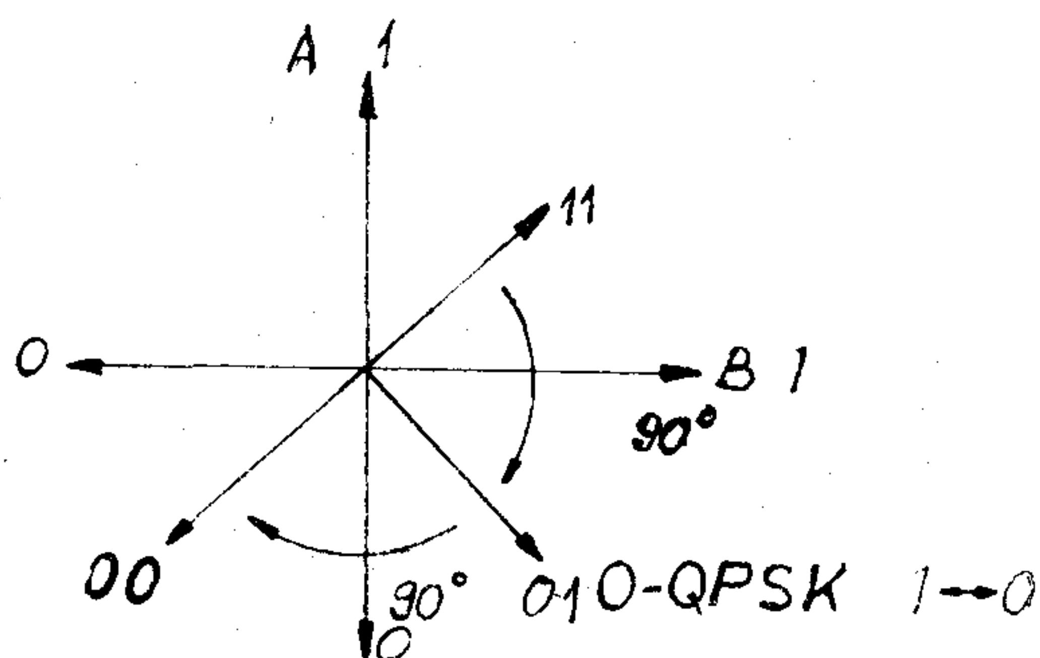
2. ábra. QPSK és O-QPSK moduláció vektorábrája
