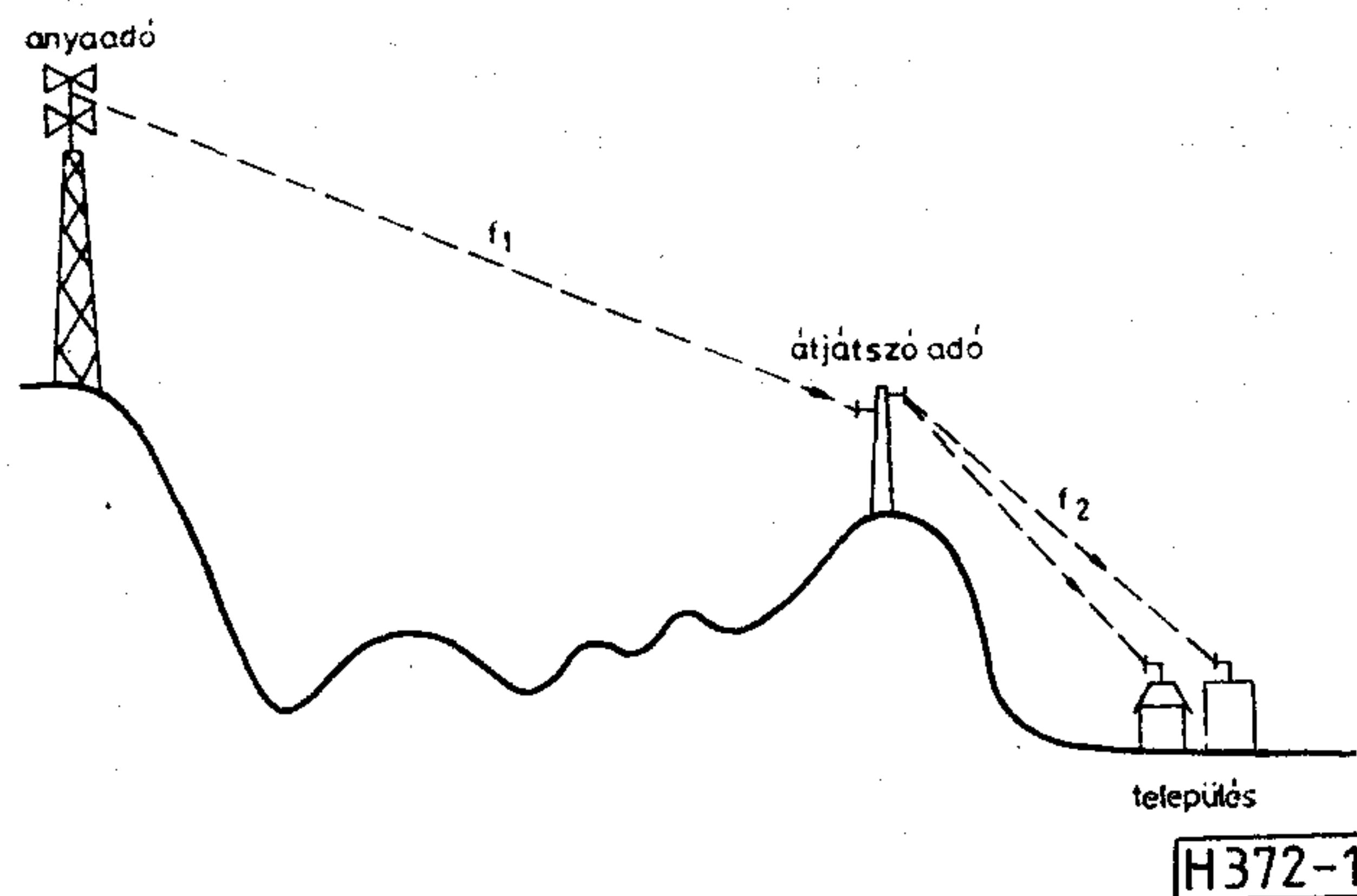
1. ábra. Átjátszás elve
