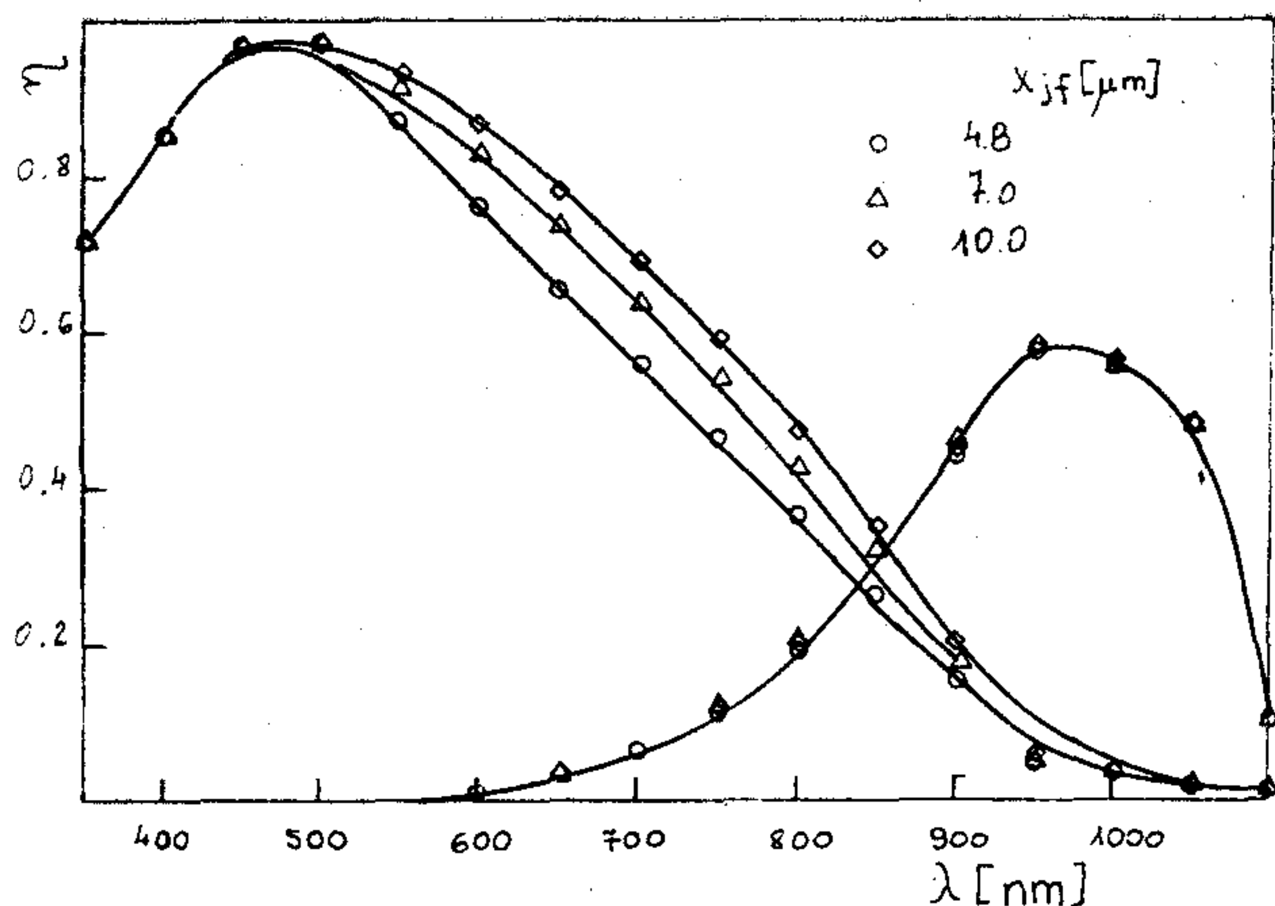
9. ábra. Kvantumhatásfok az A és F diódákban, xe = 12 \mu\text{m} , változó paraméter x_{jf}
