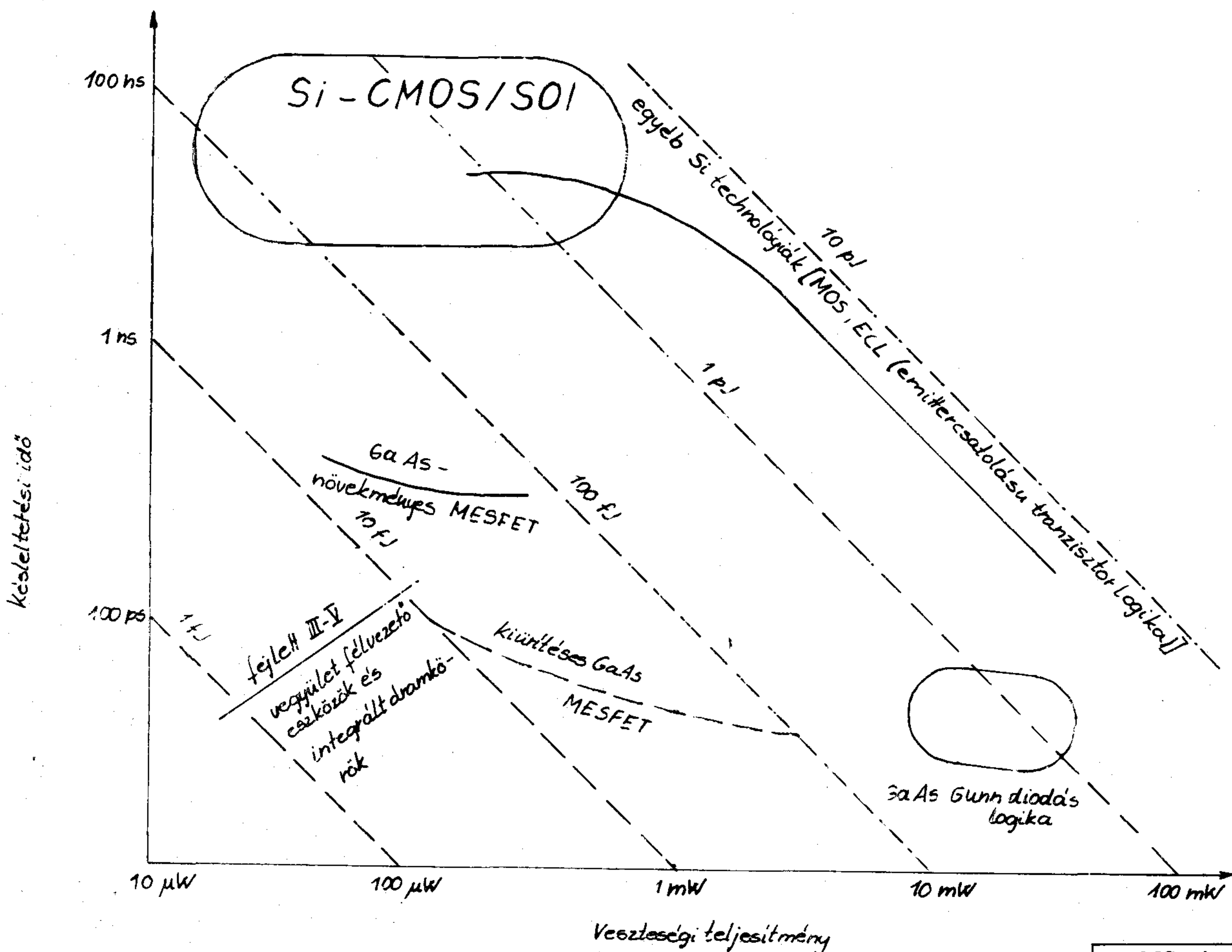
1. ábra. Késleltetési idő/veszteségi teljesítmény összefüggése
