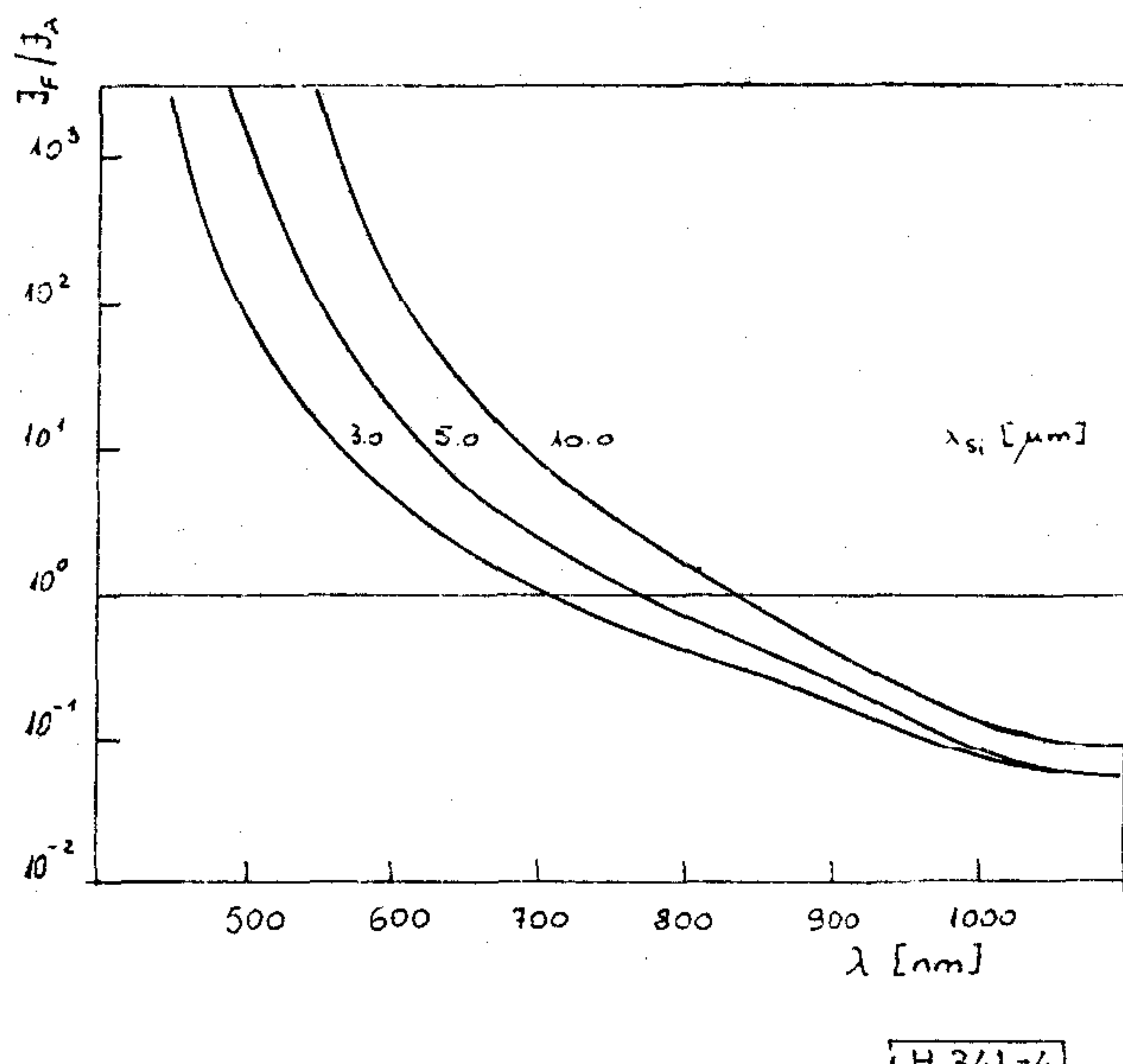
4. ábra. Ideális, \eta=1 kvantumhatásfokú diódákból felépített színérzékelő spektrális karakterisztikája
