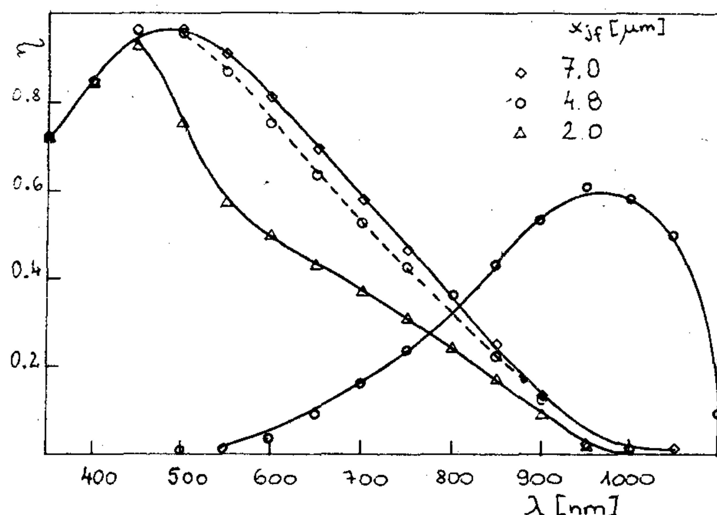
10. ábra. Kvantumhatásfok az A és F diódákban, xe = 8 \mu\text{m} , változó paraméter x_{jf}
