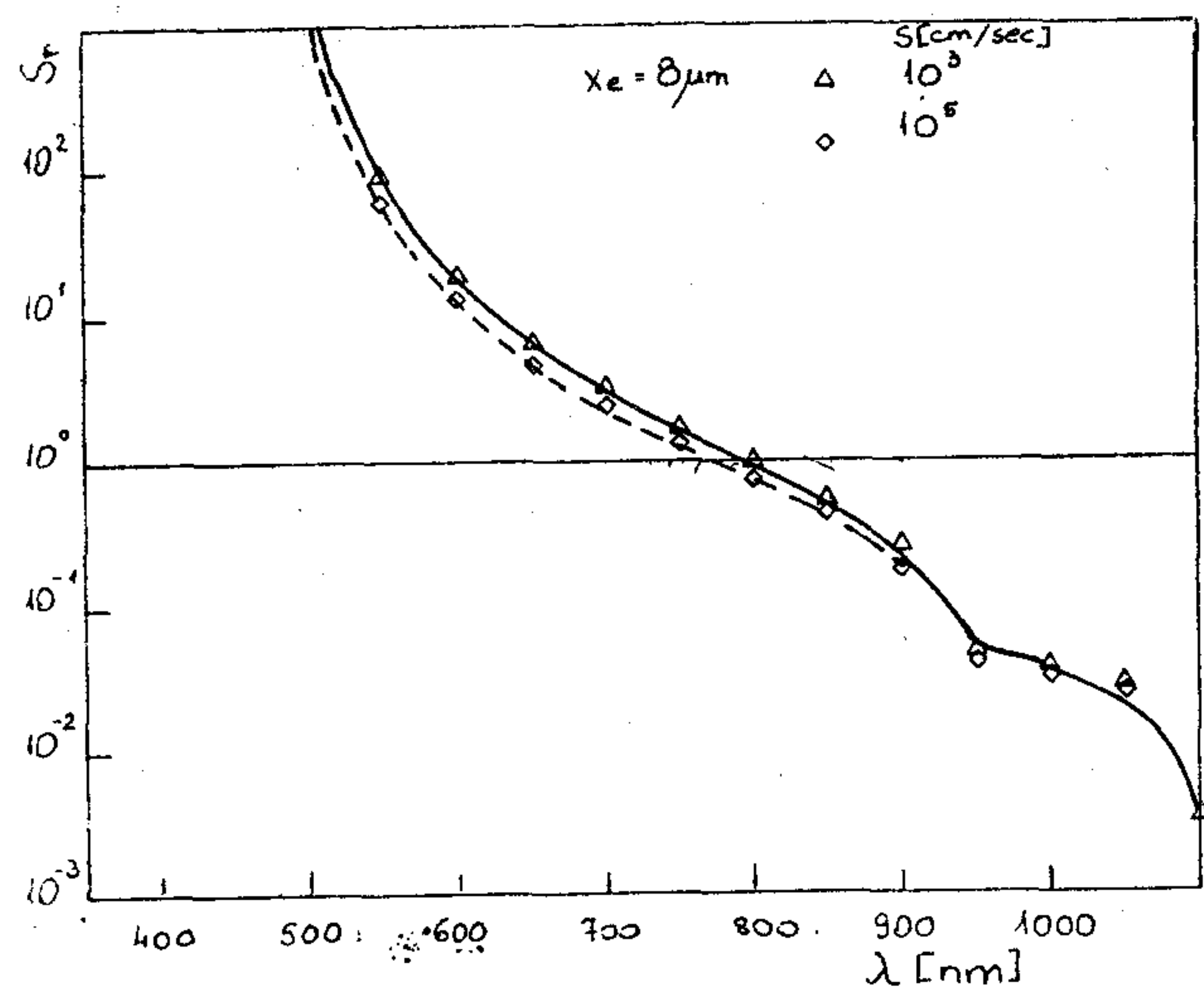
14. ábra. Spektrális karakterisztika, x_e = 8 \mu\text{m} , x_{jf} = 4,8 \mu\text{m} , változó paraméter a felületi rekombináció sebesség S
