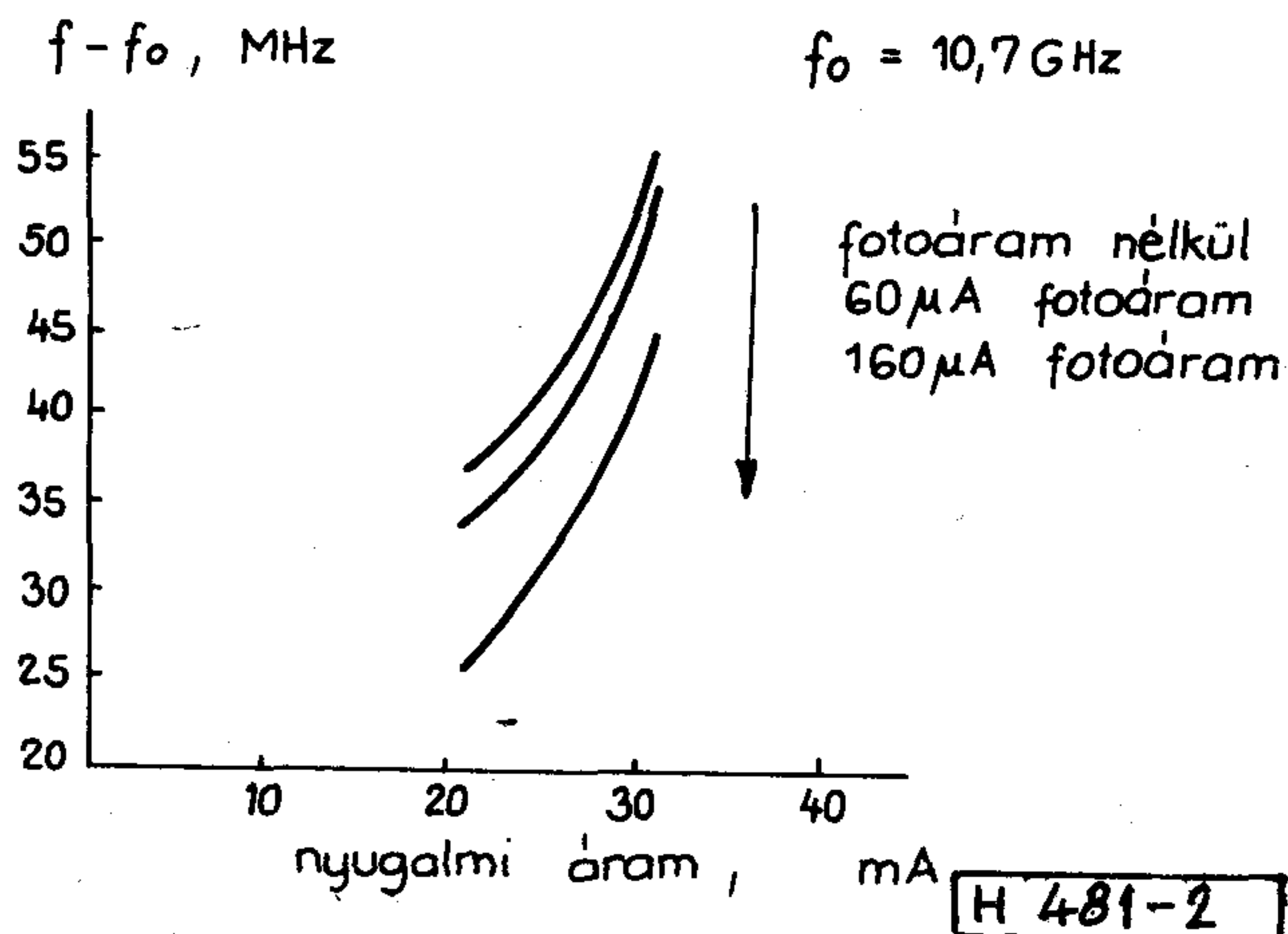
2. ábra. Egy IMPATT-diódás oszcillátor teljesítményének és frekvenciájának változása a megvilágítás függvényében [7]
