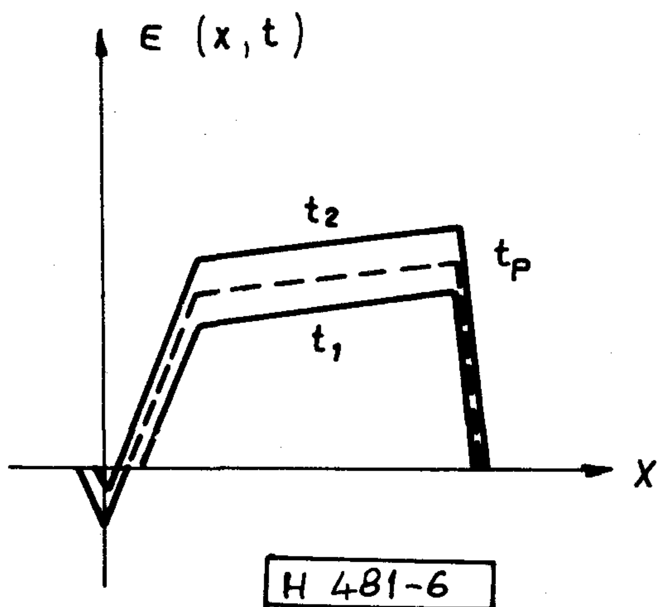
6. ábra. A Barrit dióda működéséhez
