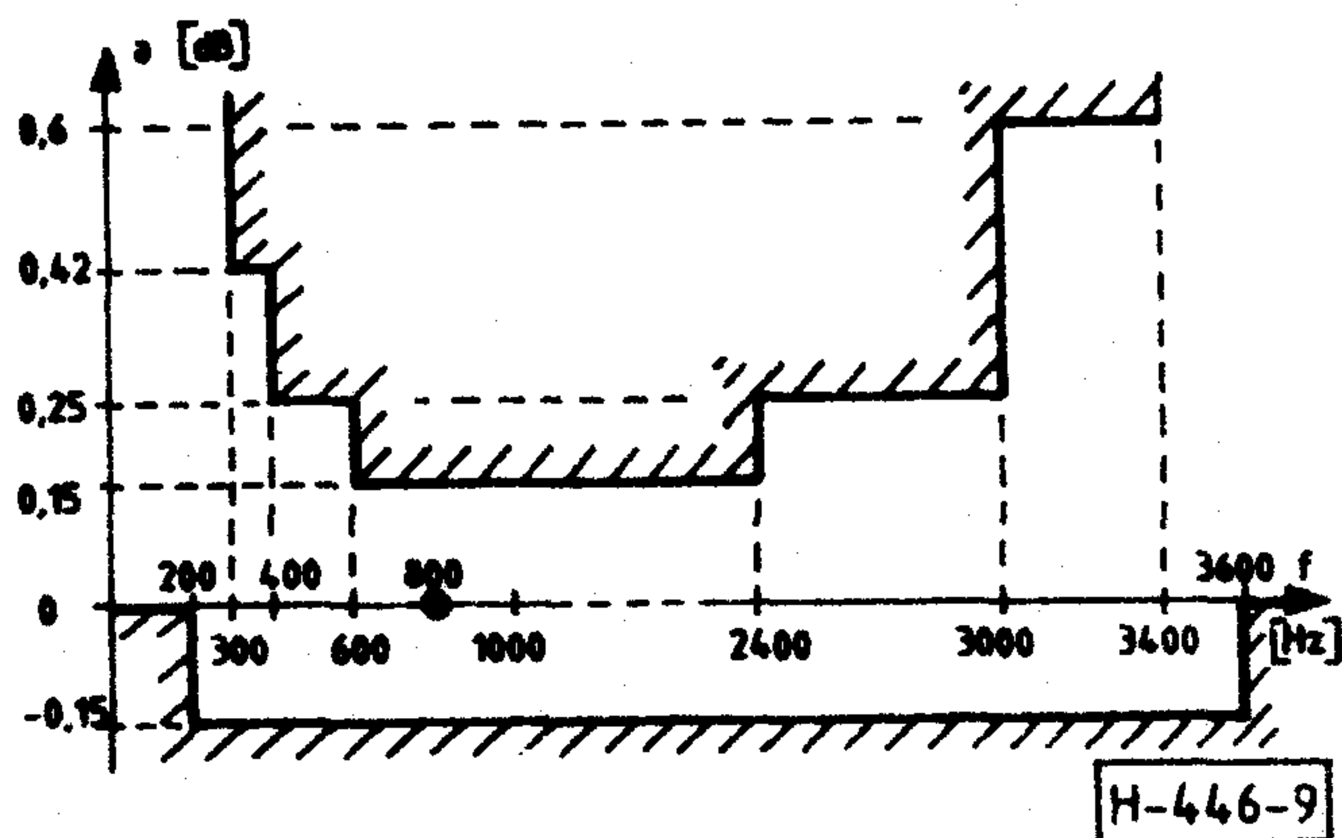
9. ábra. A szűrőbank egy irányára vonatkozó csillapítástorzítás tűrésmező
