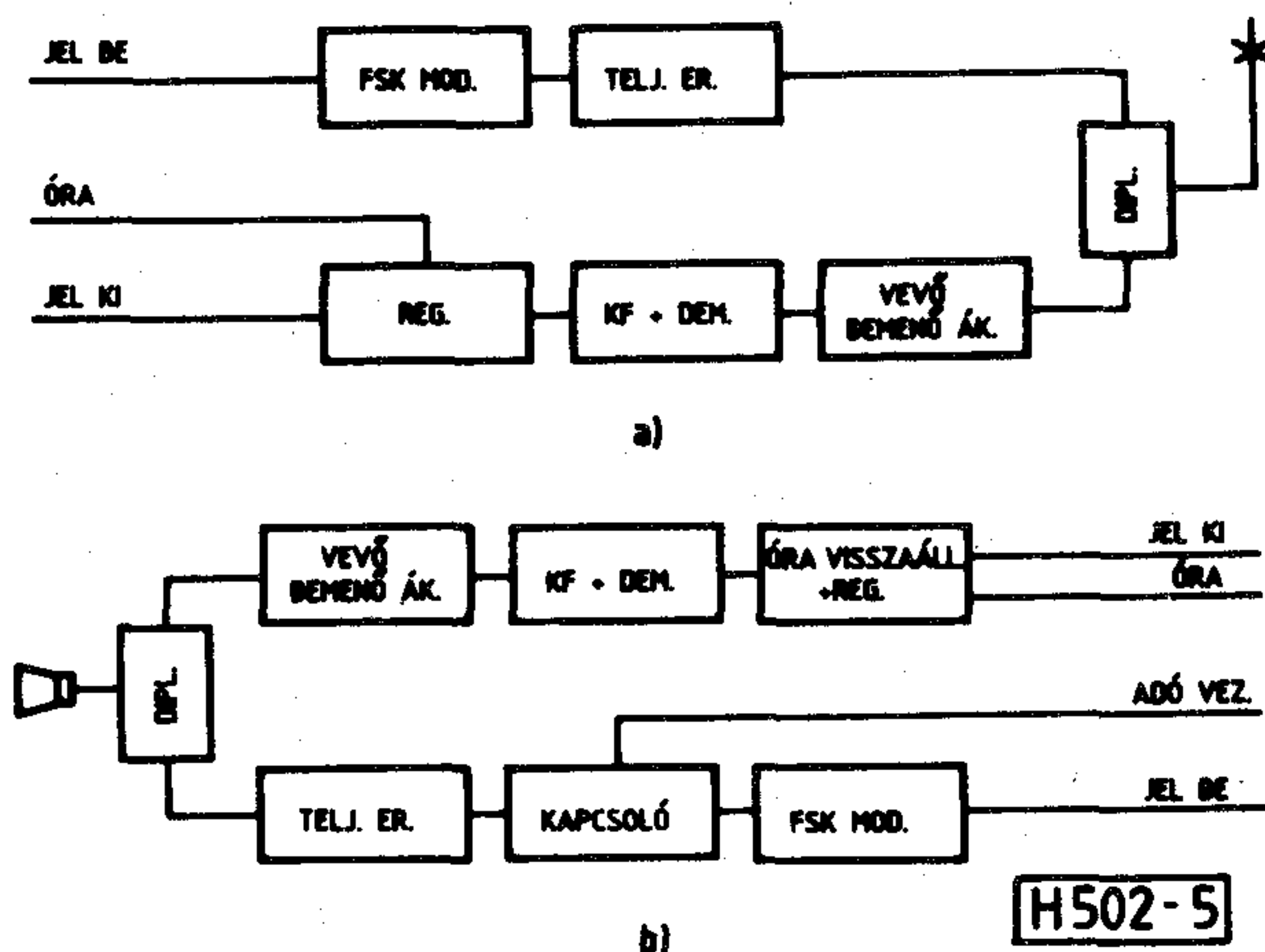
5. ábra. Központi állomási (a) ill. állomás adó-vevő blokkvázlata
