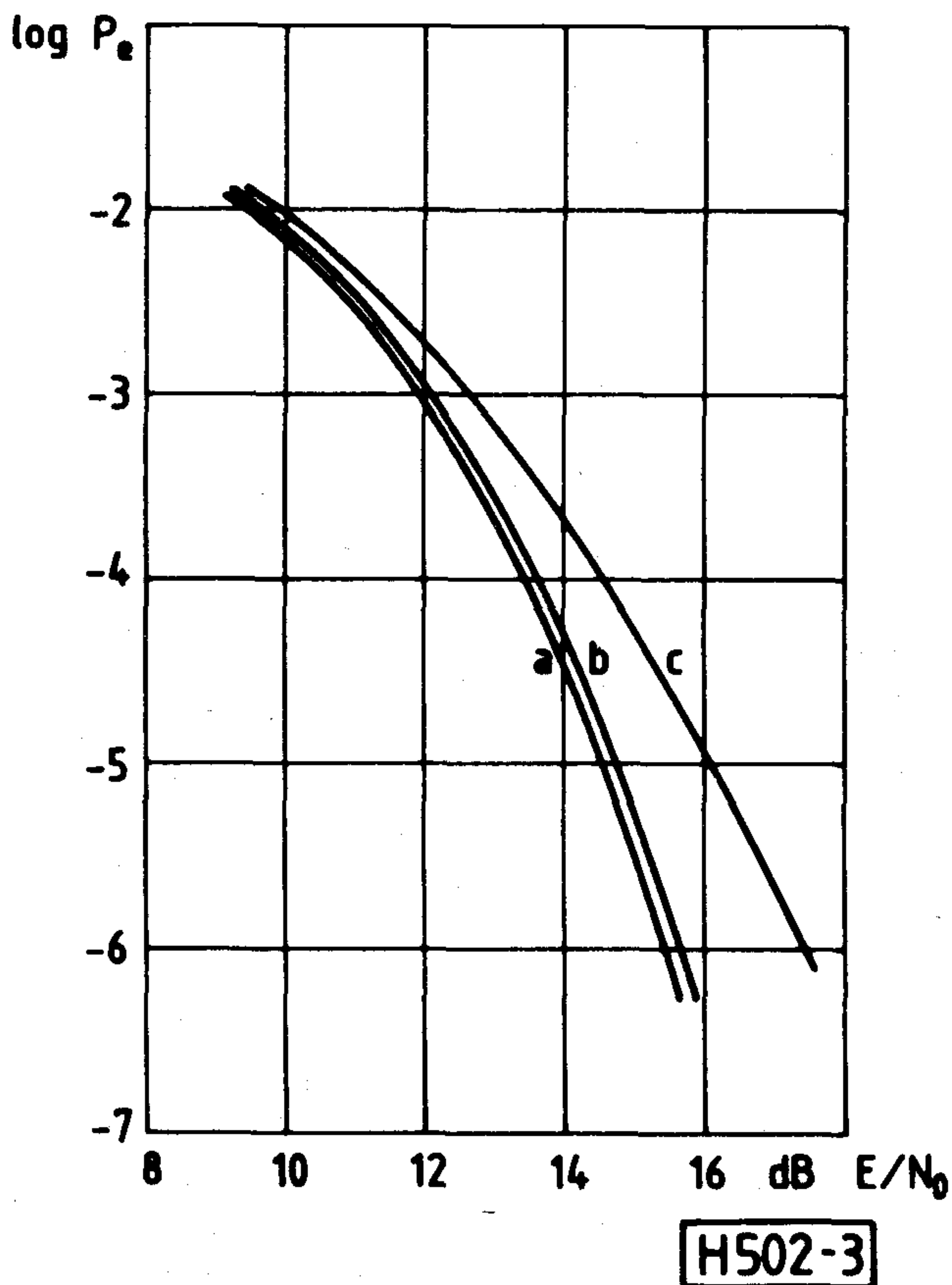
3. ábra. Hibaarány a jel-zaj viszony függvényében a) időzírtési hiba nélkül b) 100 ns, c.) 200 ns időzírtési hibával
