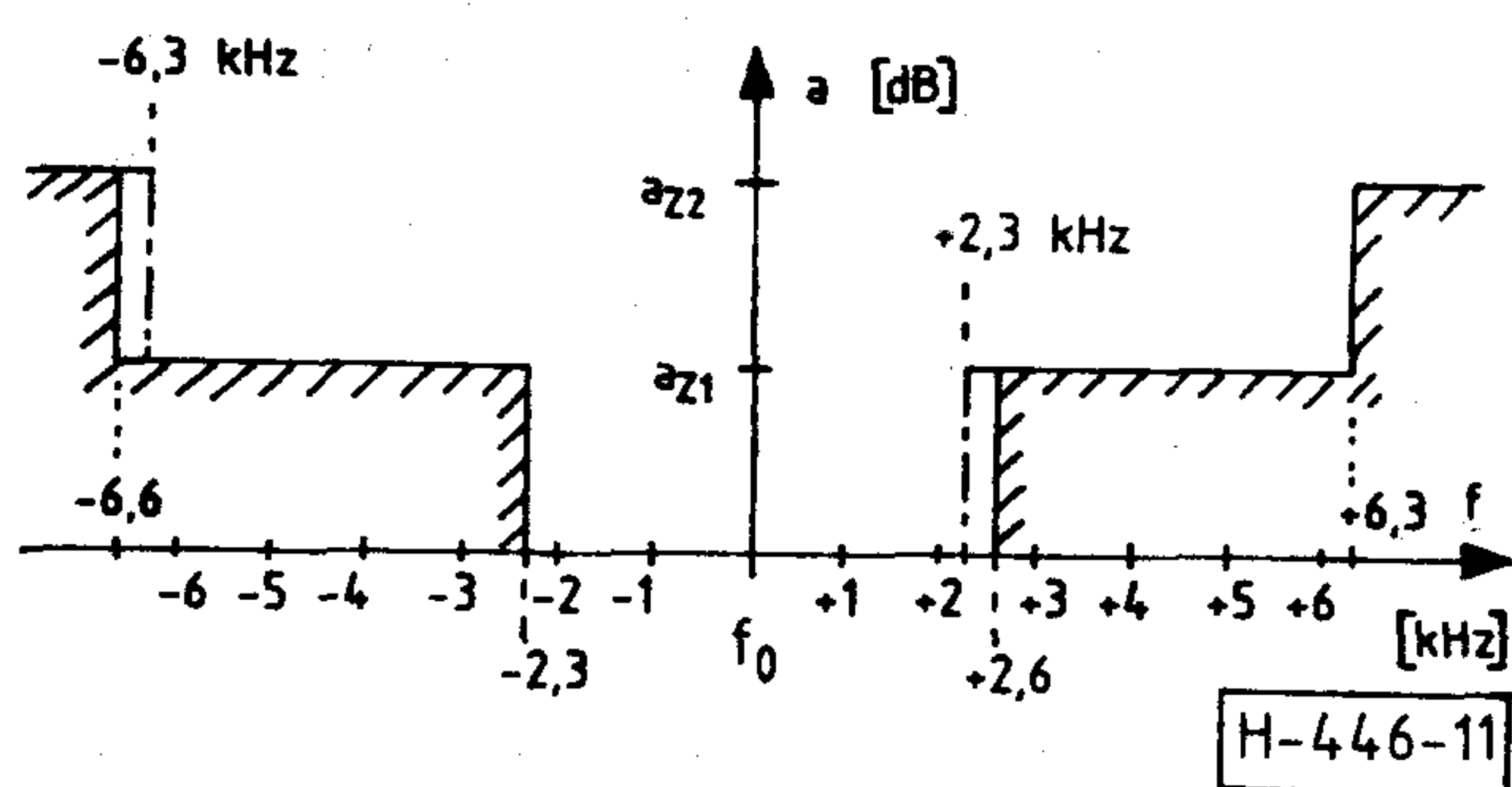
11. ábra. Az alapszűrő zárótartományi specifikációja
