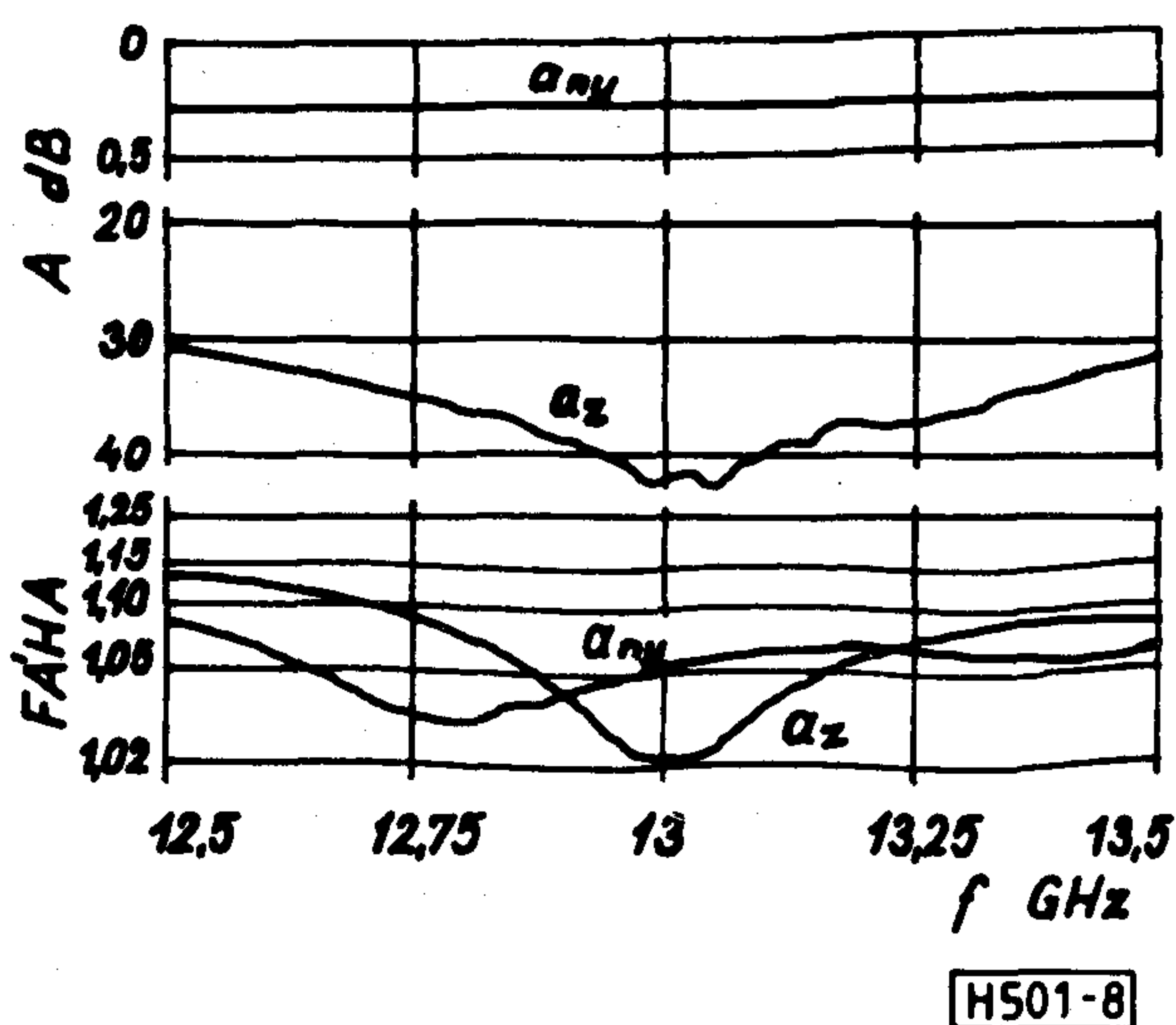
8. ábra. 13 GHz-es izolátor jelleggörbéi
