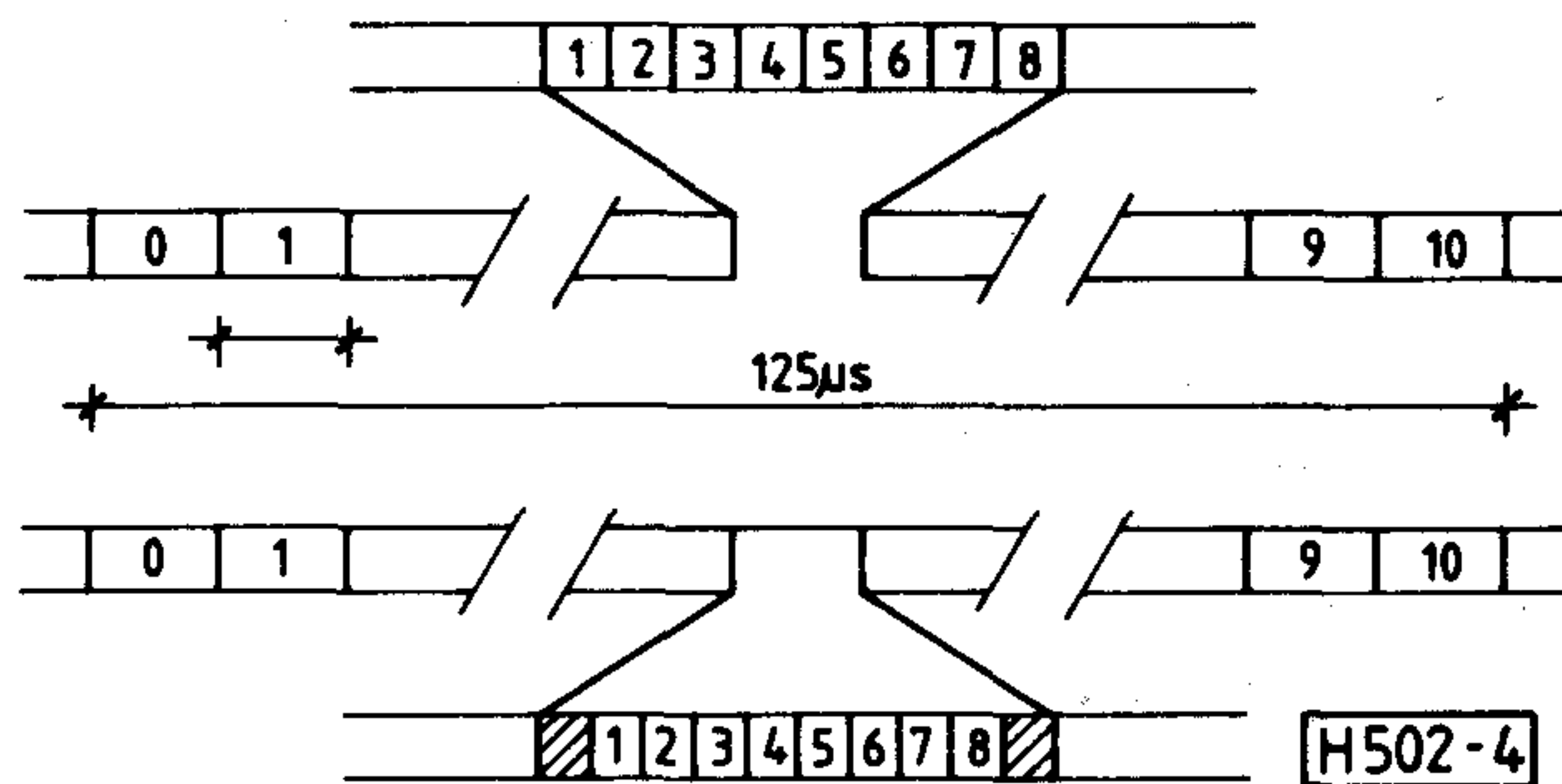
4. ábra. Jelfolyam központ-alállomás (a) és alállomás-központ (b) irányban
