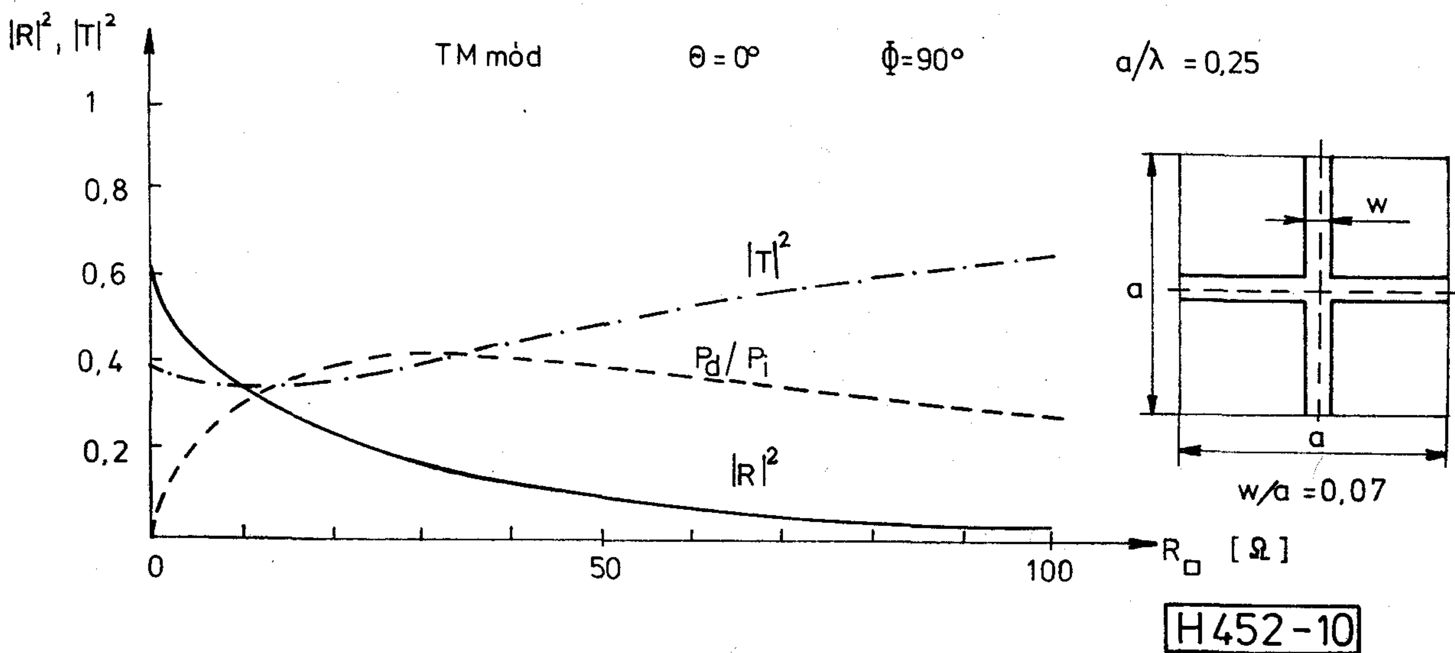
10. ábra. Teljesítményre vonatkozó szórási paraméter és P_d/P_i értékek az R_{\square} függvényében
