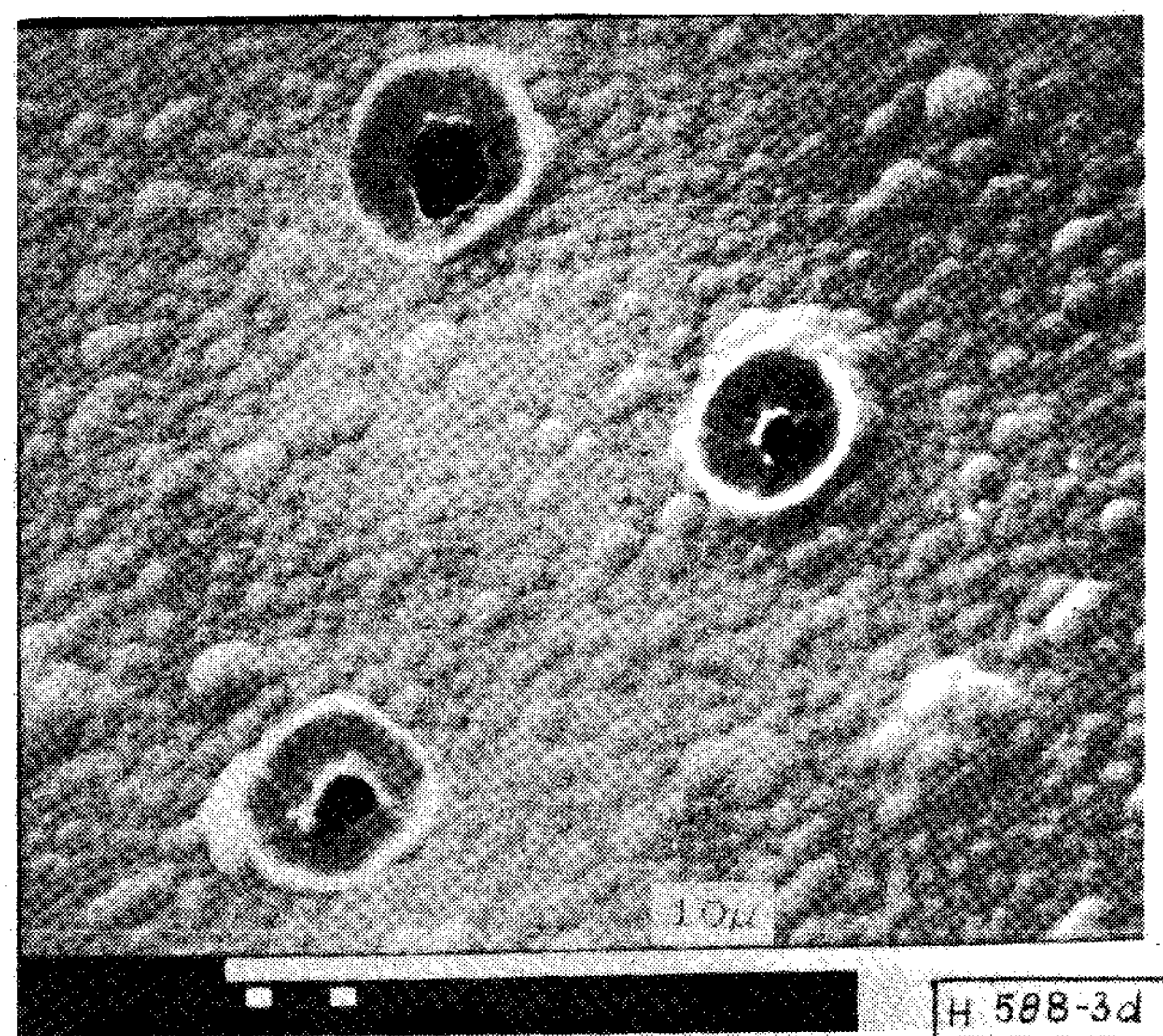
3. ábra. Plazmás nitrid szigetelőréteg felülete a felső fémszint lemarása után (3b: metszet; 3c, 3d, 3a: nézet növekvő nagyítási sorrendben)
