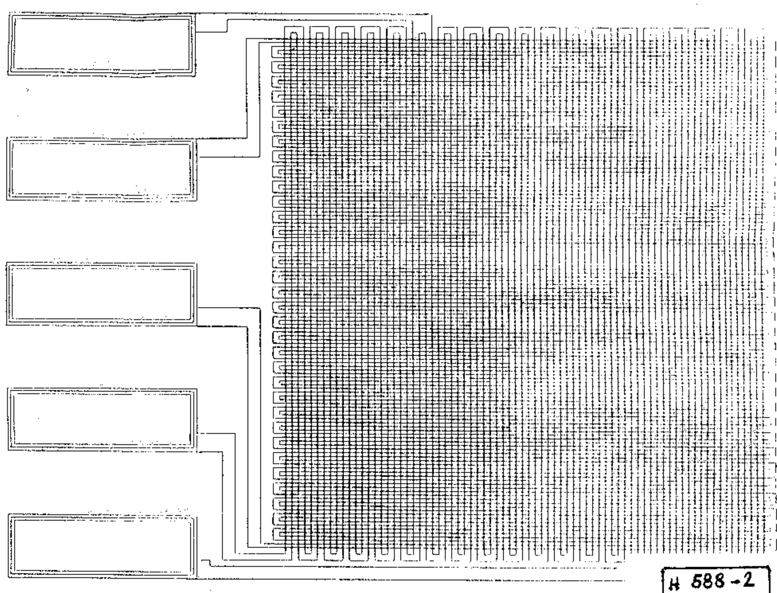
2. ábra. Merőleges fémméander struktúra layout-ja
