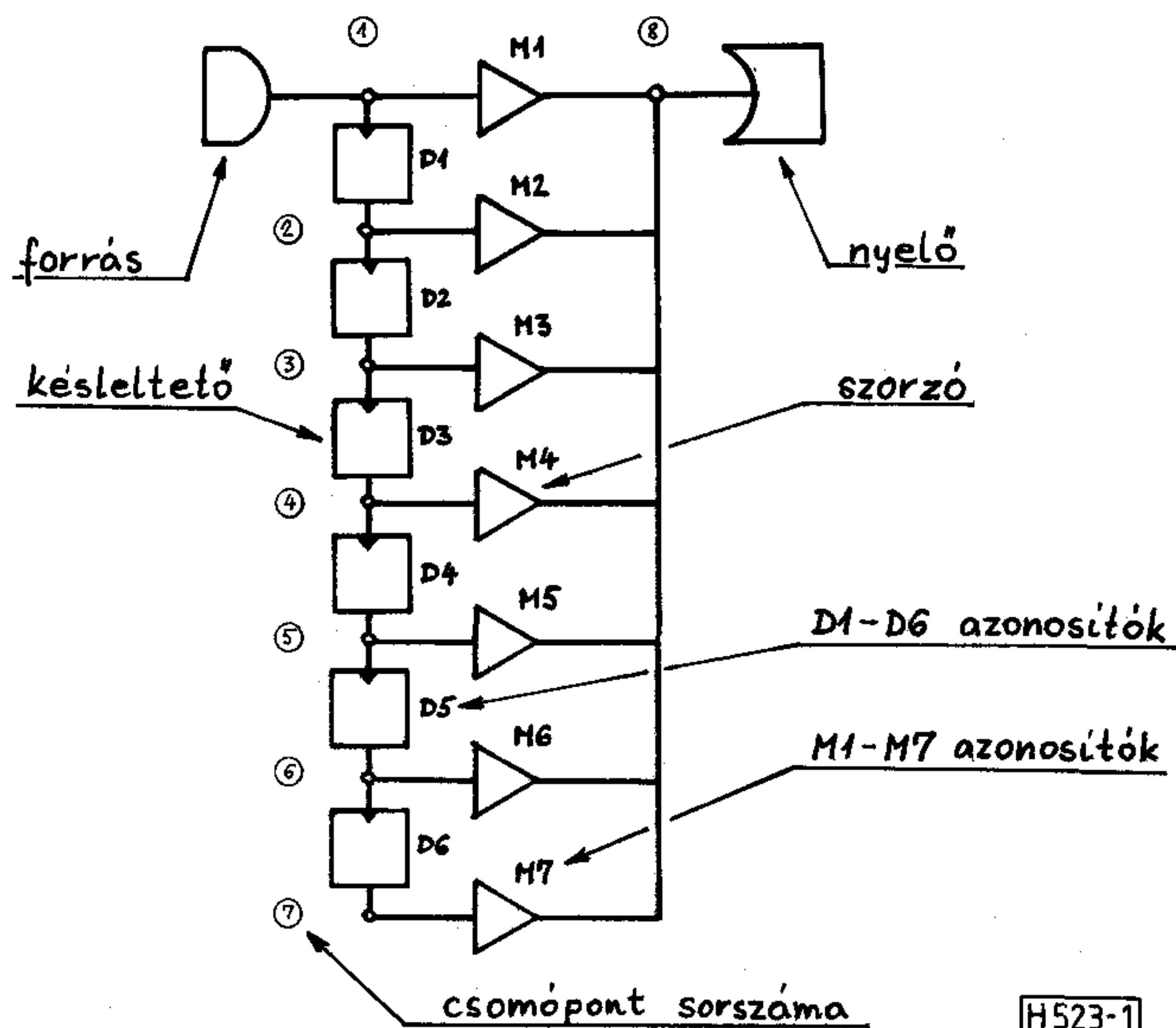
1. ábra. Diszkrét idejű, lineárfázisú aluláteresztő szűrő felépítése
