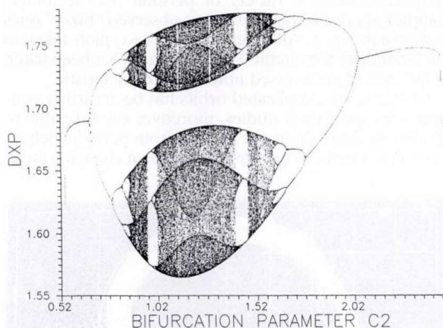
Fig. 4. C_3 bifurcation diagram (for fixed R_1=R_2=R_3=1\Omega , C_1=C_3=1F , m_0=-33,03 ; m_1=330,0 ; \sigma_{bp}=0,2 ).
