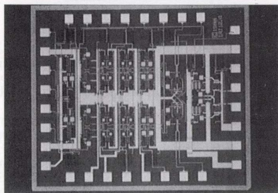
Fig. 10. PHILIPS-LEP S-band QPSK modulator
