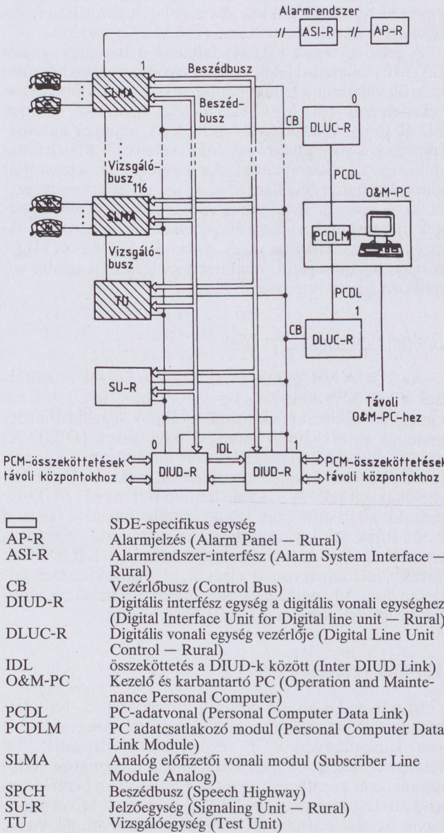
3. ábra. Az SDE digitális kisközpont struktúrája és az egyes egységek együttműködése
