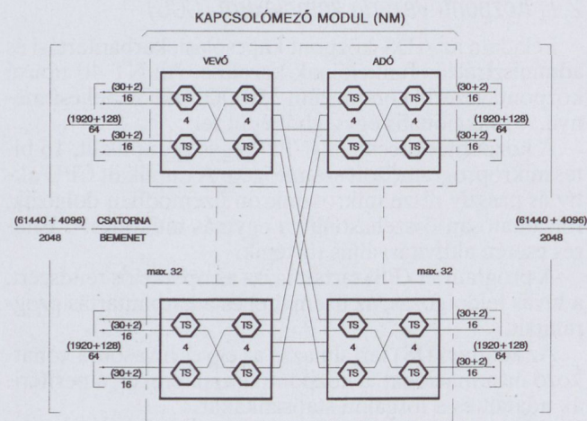
2. ábra. Kapcsolómező
