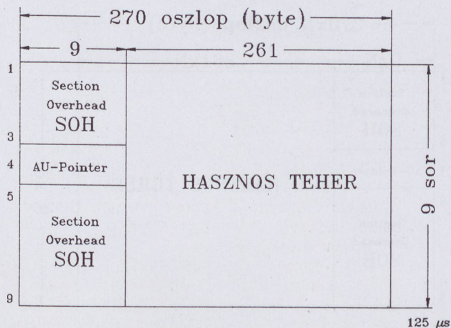
1. ábra. STM-1 keret
