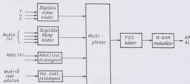
11. ábra. Digicypher kódor
