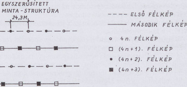
5. ábra. A MUSE rendszer mintavételezési algoritmus
