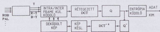
21. ábra. Kombinált, rétegzett kódoló tömbvázlata
