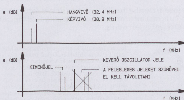
1. ábra. A kimenőjel előállításának vázlata a hagyományos eljárásnál
