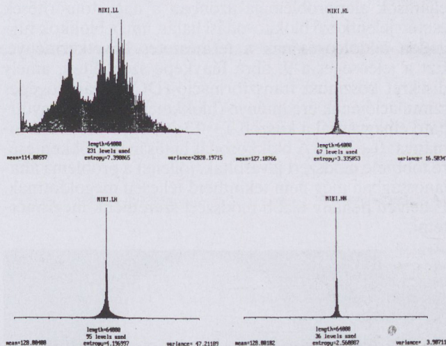
7. ábra. Részsávok hisztogramjai
