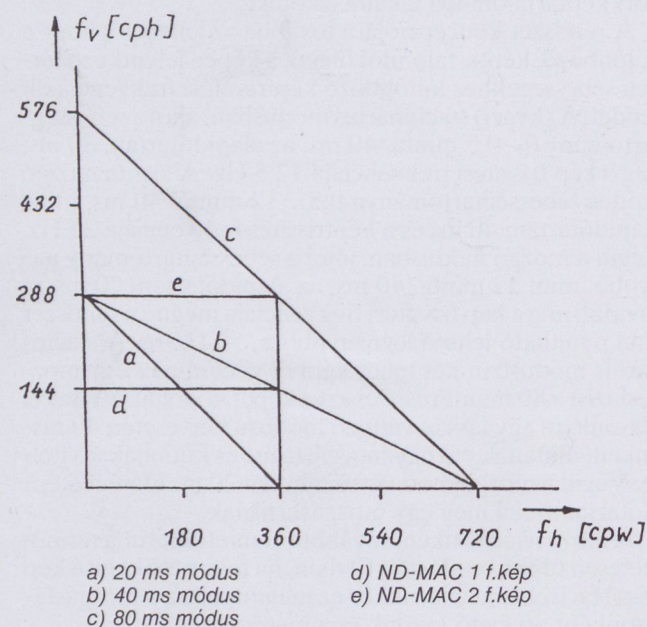
7. ábra. Világosságsjel térbeli spektrumképei
