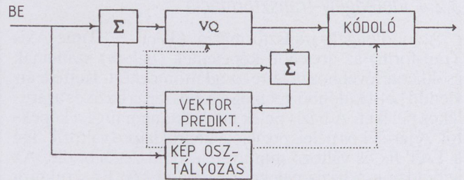
17. ábra. Prediktív VQ tömbvázlata
