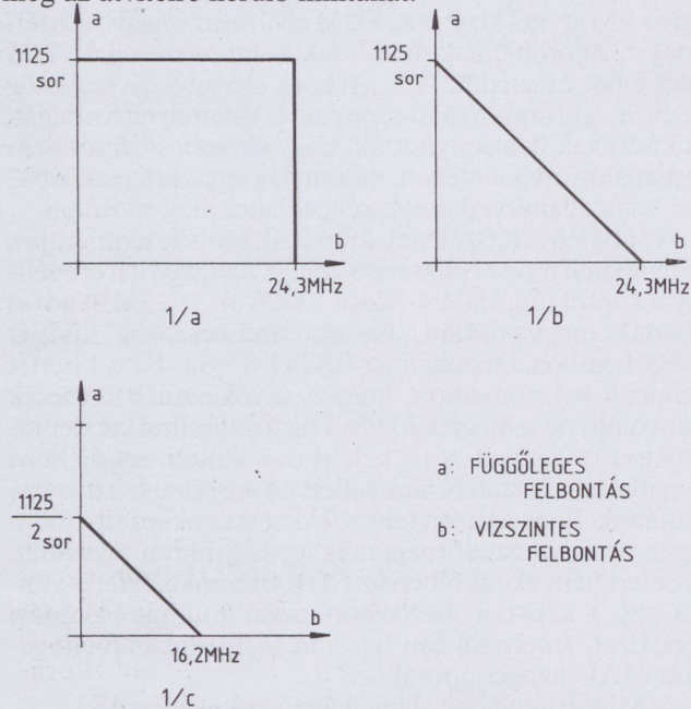
1. ábra. A MUSE rendszer kétdimenziós spektruma
