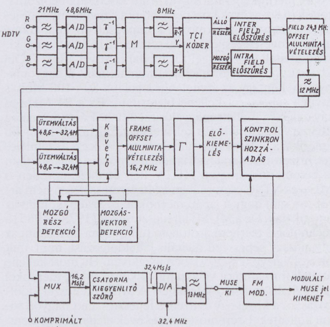
4. ábra. A MUSE kóder felépítése
