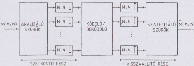
4. ábra. Részsávkodekódoló rendszer tömbvázlata
