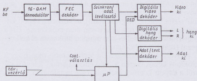
12. ábra. Digicypher dekóder
