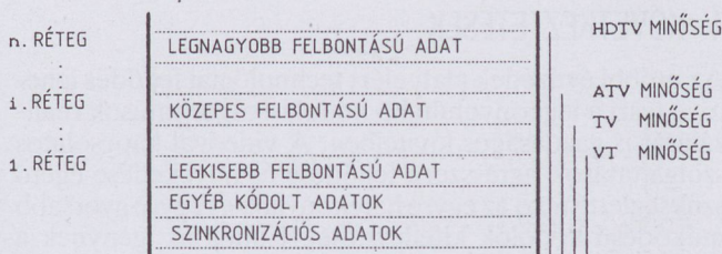
20. ábra. Rétegzett, változó bitsebességű kódolás modellje
