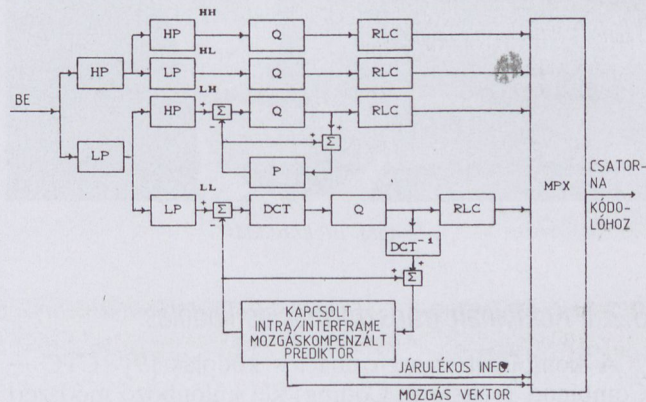
8. ábra. Részsáv kódoló tömbvázlata
