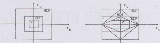
3. ábra. Felbontási szintek a Fourier-térben
