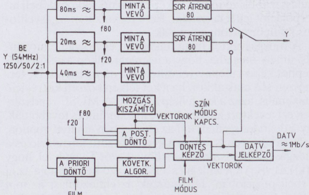
6. ábra. A mintavételei frekvencia csökkentése
