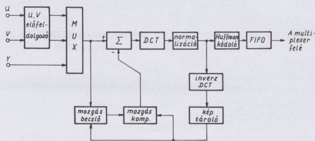
13. ábra. A digitális video-kódor tömbvázlata
