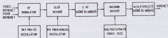
3. ábra. A programozható tv-modulátor blokkvázlata
