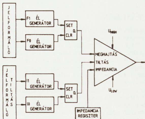
4. ábra. A késleltetés programozható finombeállítója
