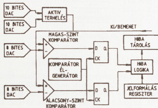
2. ábra. A komparátor/terhelés áramkör blokkvázlata
