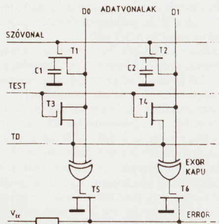
1. ábra. A dinamikus MOS memóriák párhuzamos tesztelésének egy megvalósítási formája
