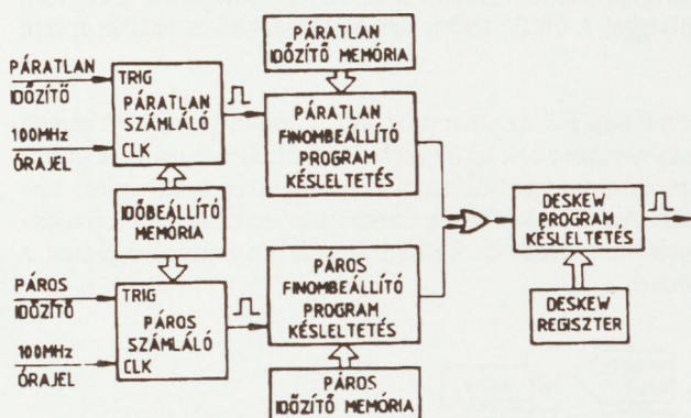
3. ábra. Az élgenerátorok áramkörei
