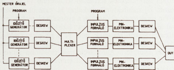
6. ábra. Teszter-Per-Pin felépítésű mérőrendszer időzítésének blokkvázlata
