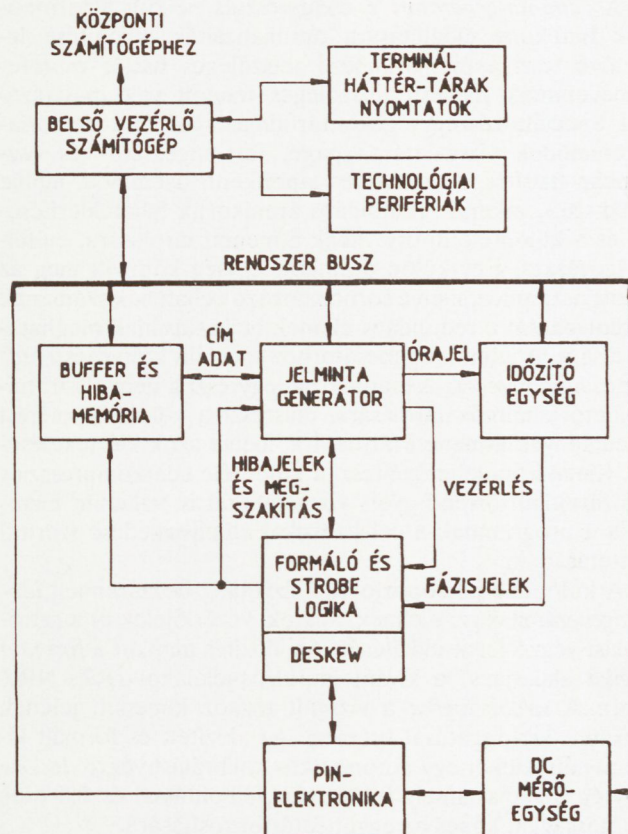
3. ábra. A hazai gyártású ICOMAT-125 típusú memóriamérő berendezés blokkvázlata
