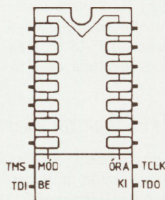
3. ábra. A BITES áramkör használata a JTAG/IEEE 1149.1 szabvány szerint
