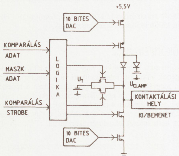
6. ábra. Az aktív terhelés áramköre
