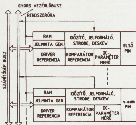
7. ábra. A pinekhez rendelt teszter blokkvázlata
