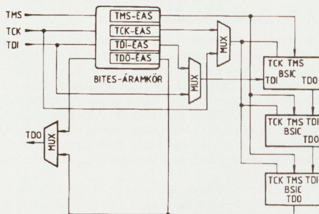
4. ábra. A BITES áramkör használata TAP vonalak előállítására
