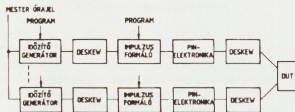
5. ábra. Osztott erőforrású (Shared Resource) mérőrendszer időzítésének blokkvázlata
