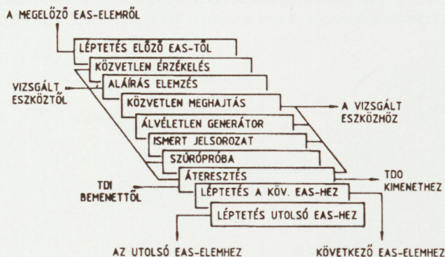
1. ábra. Boundary-scan cellák elhelyezkedése az integrált áramkör ki-, ill. bemenetein
