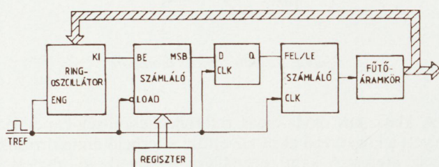
7. ábra. A hőkompenzáló rendszer vázlata
