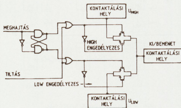
5. ábra. Az integrált meghajtó egyszerűsített blokkvázlata
