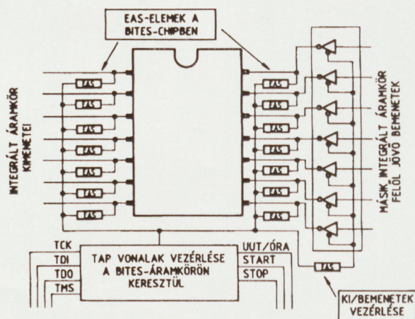
2. ábra. A BITES áramkörön belüli EAS elemek funkciói
