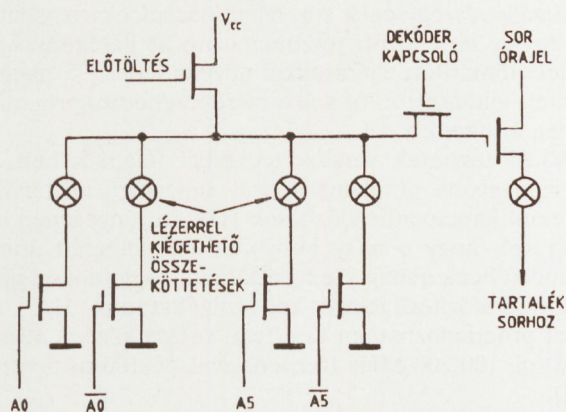
2. ábra. A beiktatott tartaléksor dekodérének programozása az összeköttetések lézeres átvágásával
