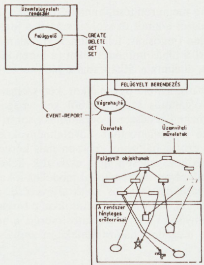
5. ábra. A központosított felügyelet szolgáltatásai és átviteli eljárása: CMIS/CMIP
