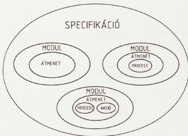
9. ábra. Az Estelle nyelv hierarchiája
