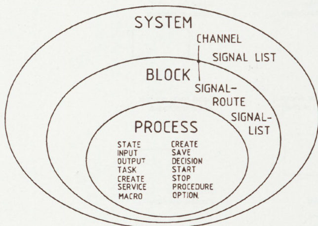
8. ábra. Az SDL nyelv hierarchiája
