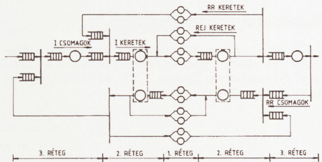
5b. ábra. X.25 protokollok szemaforos modellje
