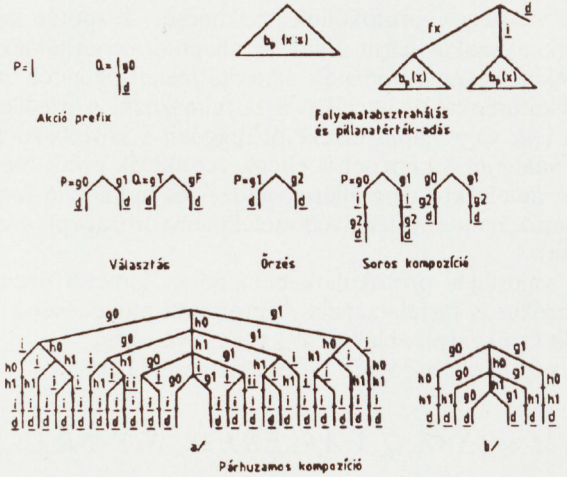
6. ábra. CCS viselkedési fák
