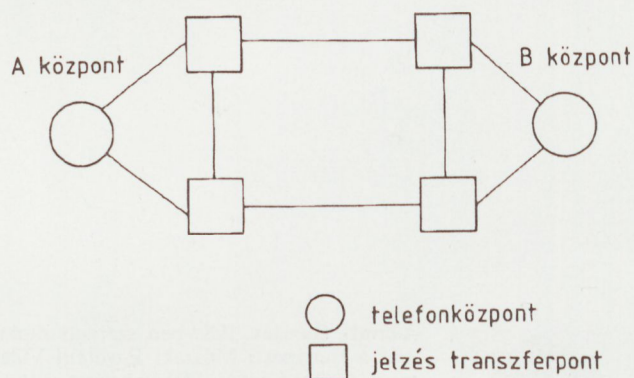
2. ábra. 7-es jelzésrendszeri hálózat
