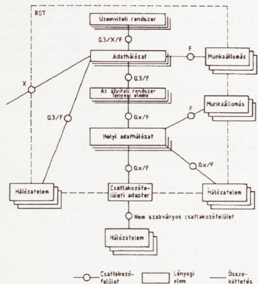
6. ábra. Az RGT fizikai felépítésének példája. (Megjegyezzük, hogy kétféle Q illesztőfelület képzelhető el: Q_3 és Q_x . Q_x Q_3 részalmazát képezi, és olyan berendezésekben használatos, amelyek vagy kevés számítási erőforrással rendelkeznek, vagy nincs szükségük Q_3 valamennyi szolgáltatására.)
