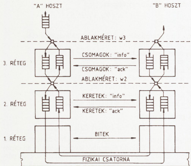
5a. ábra. X.25 protokollok
