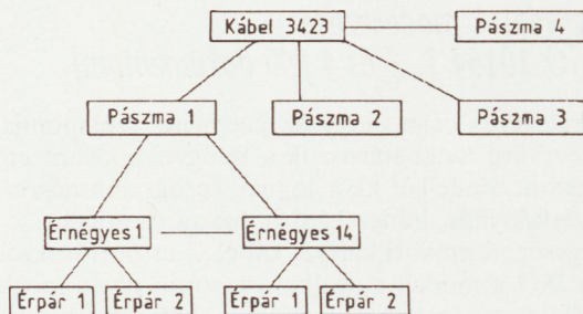
3. ábra. Beágyazódási fa. Példa: 112 érpárt tartalmazó kábel
