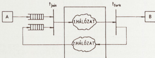
4. ábra. Szemaforos protokollmodell
