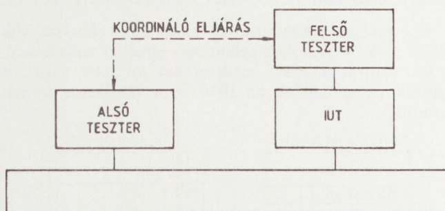
13. ábra. Az alsó és felső teszter
