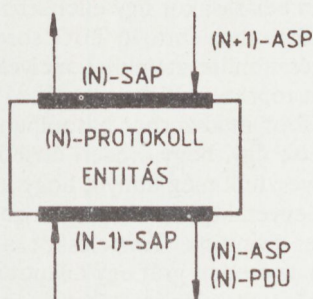
12. ábra. A vizsgálat elemei: az absztrakt szolgálati primitívek és a protokoll-adatelemek
