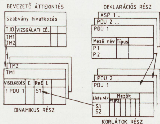
14. ábra. A TTCN táblázatok egymáshoz való viszonya
