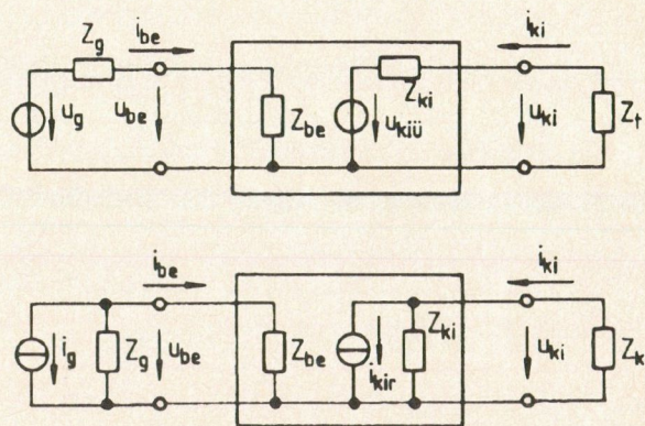
2. ábra. Aszimmetrikus erősítő helyettesítőképei (a kimeneti generátorok mérőiránya az alkalmazott passzív mérőirányrendszernek felel meg)
