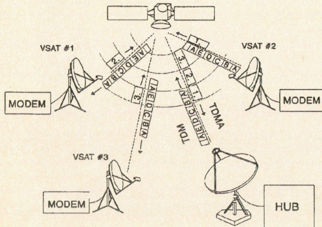
2. ábra. TDM/TDMA VSAT hálózat
