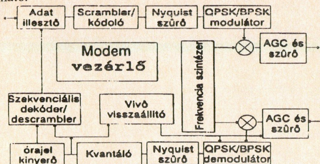
5. ábra. Modem blokkvázlat
