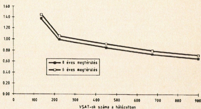
4. ábra. Fajlagos hálózati költség a VSAT szám függvényében
