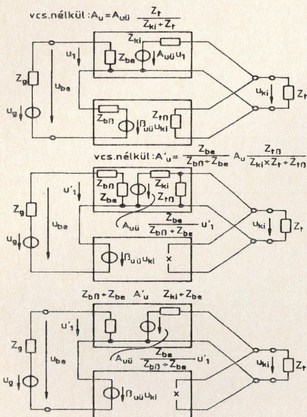
4. ábra. A visszacsatolt erősítő helyettesítőképének azonos átalakítása soros feszültségvisszacsatolás esetén, nem ideális visszacsatoló hálózat feltételezésével.
