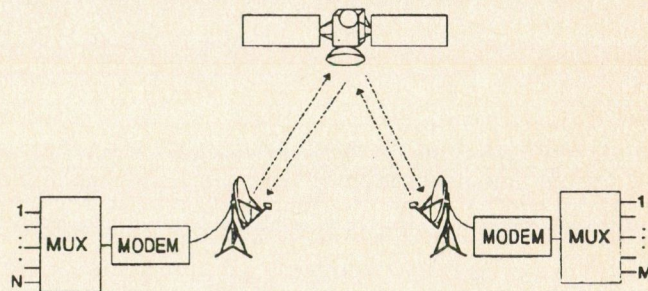
1. ábra. MCPC pont-pont összeköttetés
