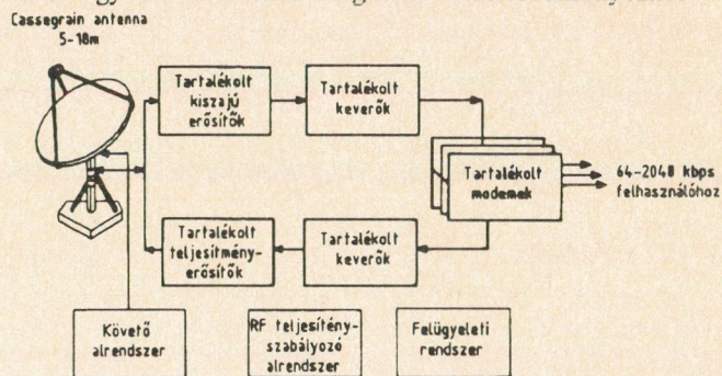
2. ábra. Nagy földi állomás blokkvázlata
