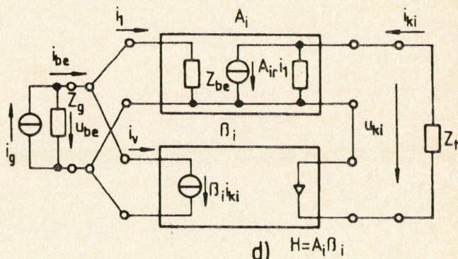
3. ábra. Visszacsatolások ideális visszacsatoló taggal: a.) soros feszültség (SF), b.) párhuzamos feszültség (PF), c.) soros áram (SÁ) és d.) párhuzamos áram (PÁ) visszacsatolás
