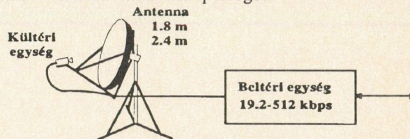
3. ábra. VSAT állomás
