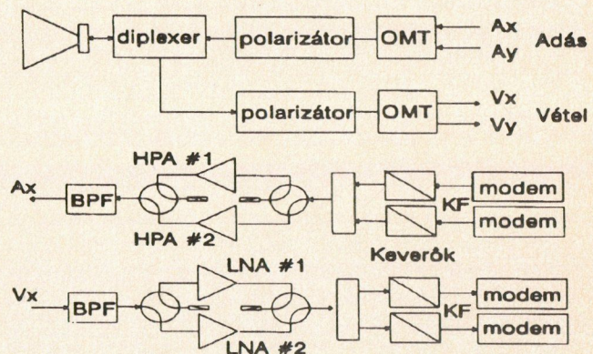
1. ábra. Általános célú földi állomás rendszertechnikai blokkvázlata
