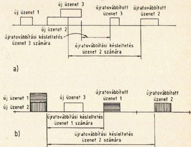
3. ábra. Az ALOHA és a Slotted ALOHA hozzáférési eljárás
