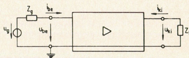
1. ábra. Aszimmetrikus erősítő
