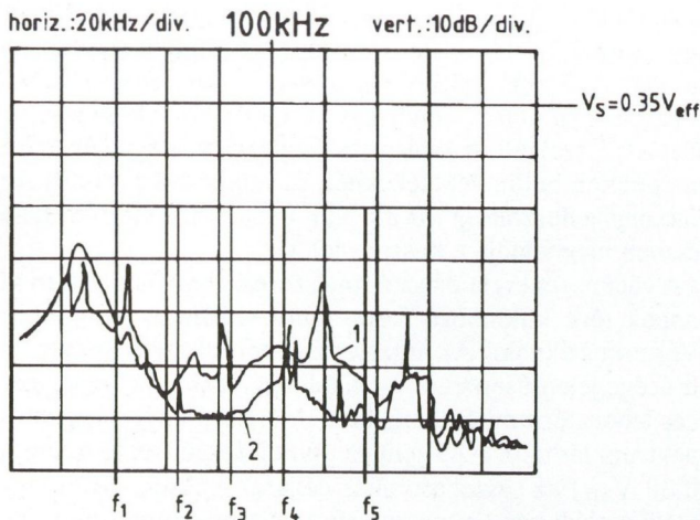
4. ábra. 1 km hosszú kábelben mért spektrum.
