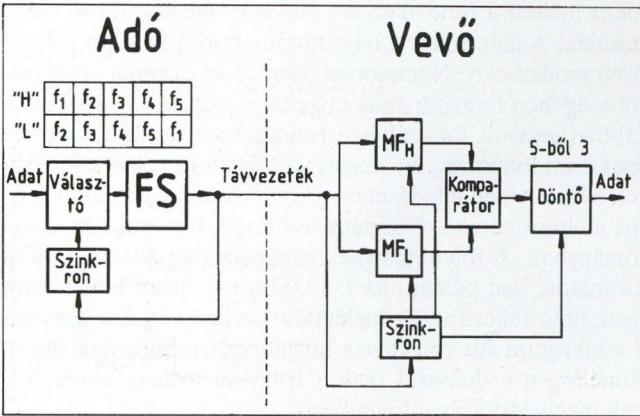
8. ábra. A frekvenciaváltásos szórt-spektrumú rendszer blokkdiagramja
