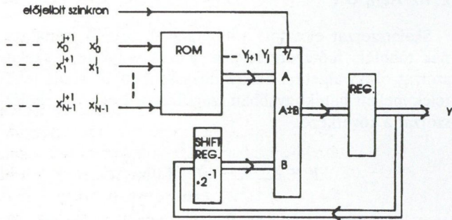
1. ábra. Peled-Liu-féle skalárszorzó blokkvázlata
