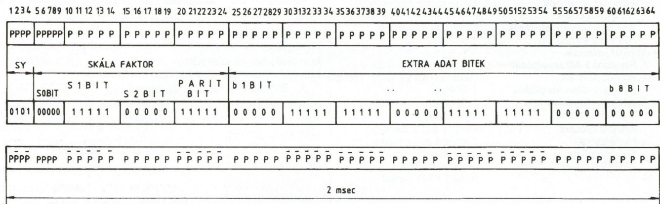
6. ábra. Jelzésátvitel a paritásbiteken
