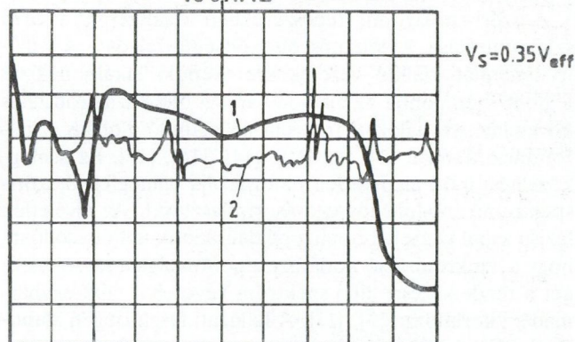
3. ábra. Gyárépületben végzett mérés.
