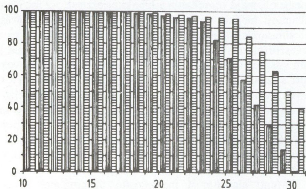
5. ábra. Hibajavító képesség (15,11) paraméterű RS kóddal 1, illetve 2 paritásszimbólummal
