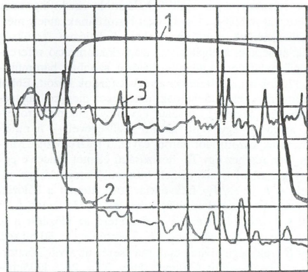
2. ábra. Interferencia spektrum házon belüli vezetékeken.
