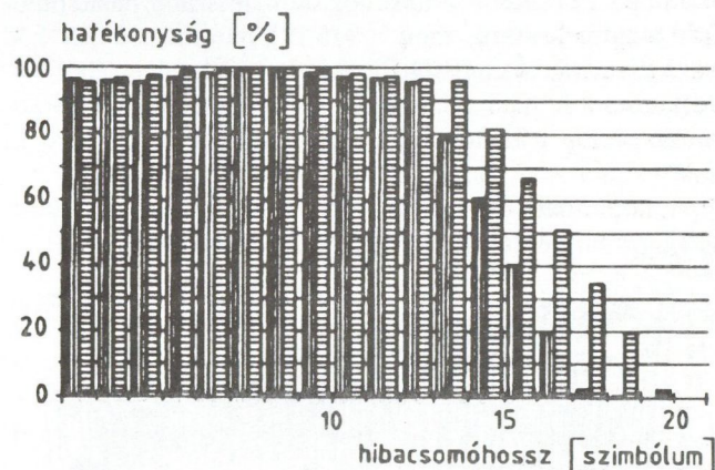
4. ábra. Hibajavító képesség (15,12) paraméterű RS kóddal 1, illetve 2 paritásszimbólummal
