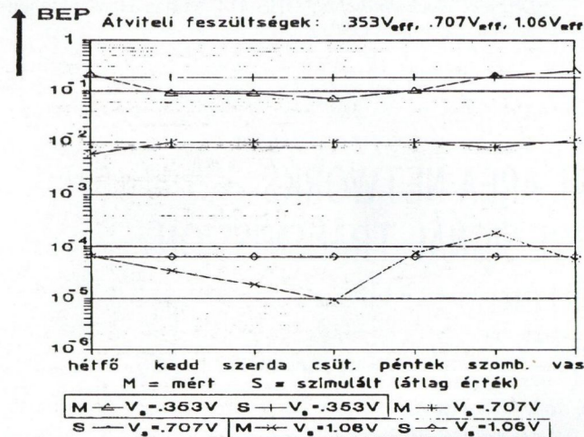
14. ábra. A mért és a számított bithiba valószínűségek összehasonlítása három különböző átviteli feszültség mellett
