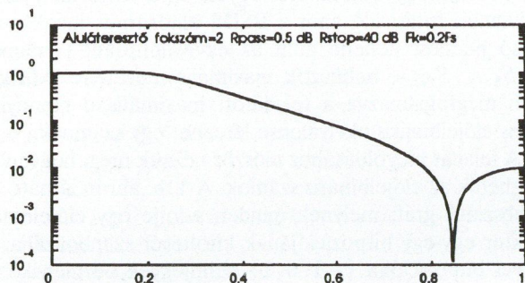
7. ábra. Elliptikus aluláteresztő szűrő amplitúdó karakterisztikája
