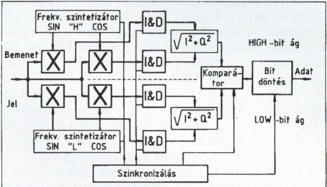
9. ábra. Az inkoherens analóg frekvenciaváltásos vevő elve
