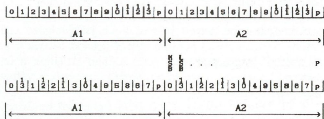
4. ábra. Egy minta közvetlen súlyozással és kiforgatott átlapolással
