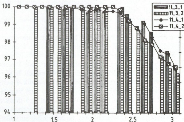
7. ábra. Az egy kódszóra vonatkoztatott hibajavító képesség összehasonlítása
