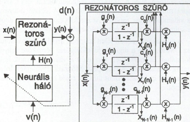
1. ábra. Neurális hálóval vezérelt rezonátoros szűrő
