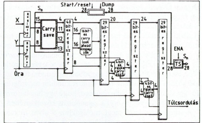
11. ábra. A megvalósított „szisztólikus” processzor mint illesztett szűrő (CMOS gate array)
