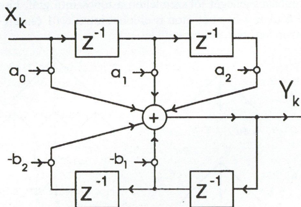
8. ábra. IIR szűrőalaptag realizálása
