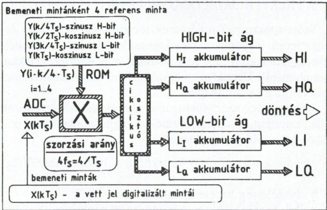
10. ábra. A digitális frekvenciaváltásos illesztett szűrő alapfunkciói
