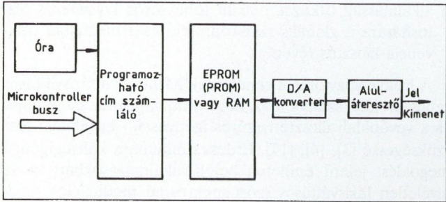
7. ábra. A digitális frekvencia-szintetizátor blokkdiagramja
