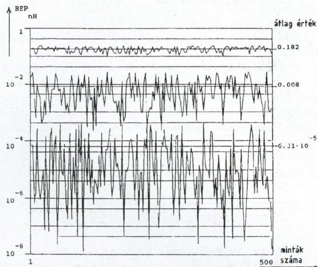
13. ábra. A bithiba valószínűség szimuláció eredményei.
