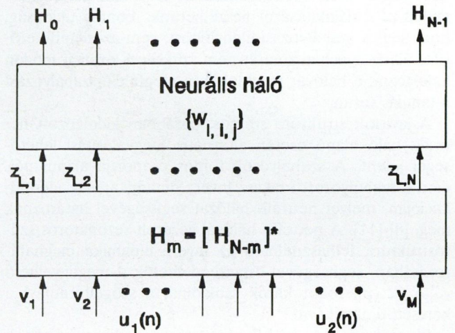
3. ábra. A neurális alrendszer kialakítása
