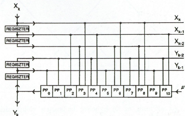
9. ábra. IIR szűrő felépítése részletsorozat számító modulokból
