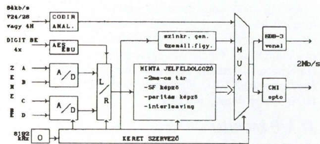
2. ábra. Az adó multiplex blokkvázlata
