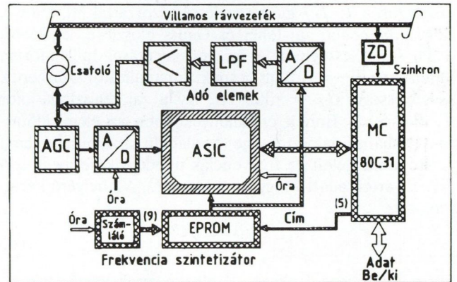
12. ábra. ASIC áramkörrel és mikrokontrollerrel megvalósított frekvenciaváltós modem prototípus
