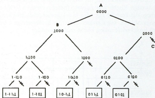
10. ábra. Az előjelbináris ekvivalensek szukcesszív approximációval történő előállításának szemléltetése
