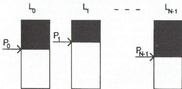
5. ábra. A nemnulla számjegyek alapján sorbarendezett listák
