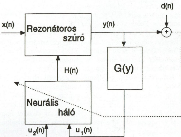
2. ábra. Neurális hálóval vezérelt rezonátoros szűrőstruktúra általánosítása
