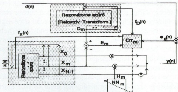
4. ábra. A kimeneti és transzformált komponenshiba kombinált használata a tanításban
