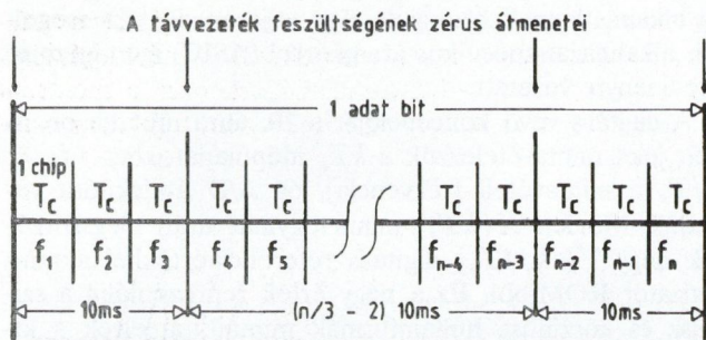
6. ábra. A hálózati feszültségen mint referencián alapuló időzítés
