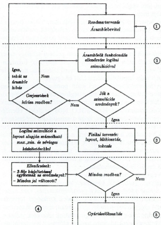
1. ábra. Egy integrált áramkör tervezésének folyamatábrája
