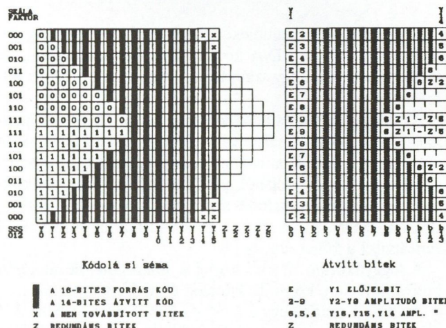
5. ábra. A lebegőpontos kompresszió sémája. a) Kódolási séma; b) Átvitt bitek.
