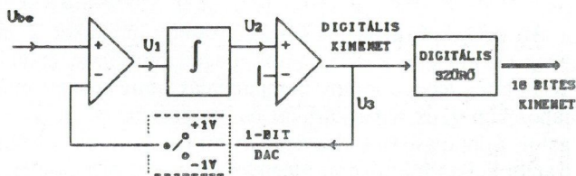
1. ábra. Az A/D konverter blokkvázlata
