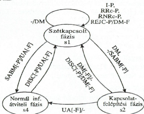
5. ábra. A P' részgráf
