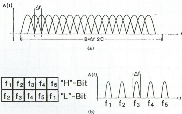
5. ábra. (a) Spektrum hasznosítás ortogonális jelekkel;
