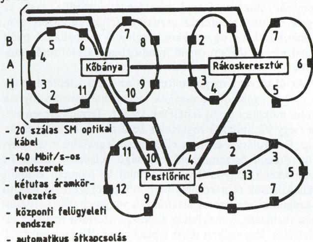
4. ábra. Az EPT hálózatstruktúrája
