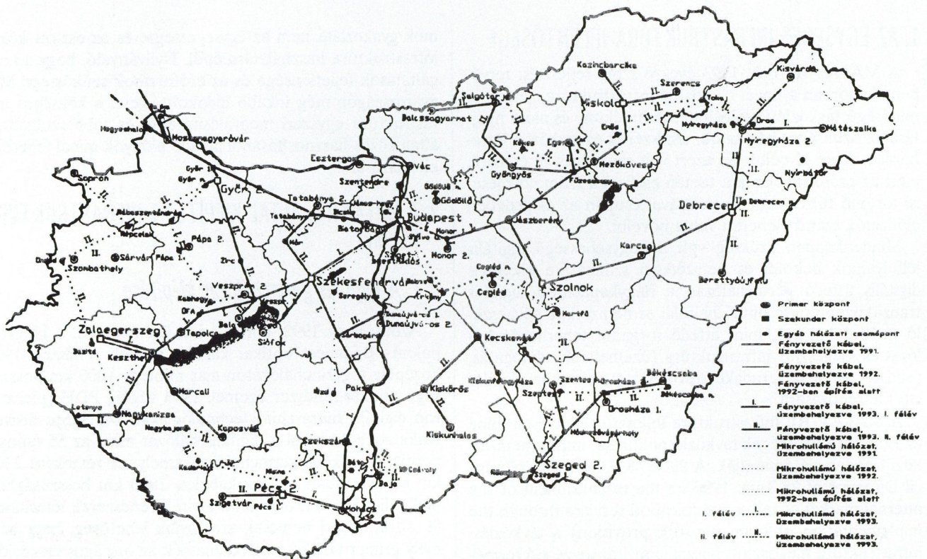
1. ábra. Az optikai és mikrohullámú gerinchálózat fejlesztése
