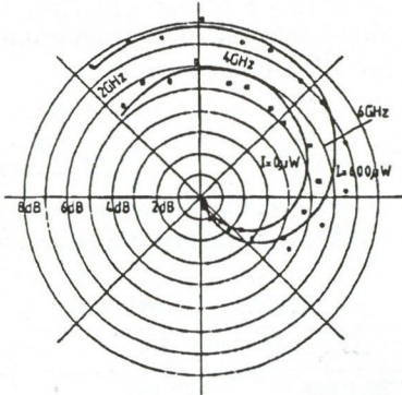
Fig. 2. S_{21} parameters
