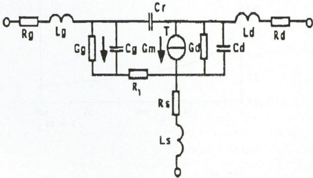
Fig. 4. MESFET equivalent circuit
