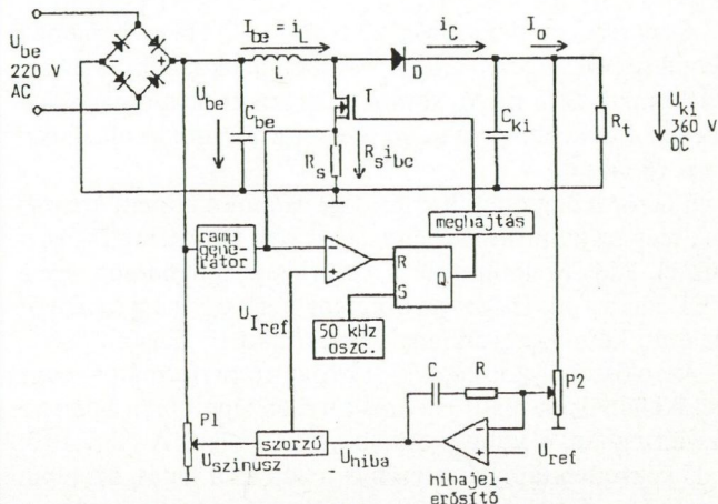
5. ábra. A 400 VA-es modell blokkvázlata
