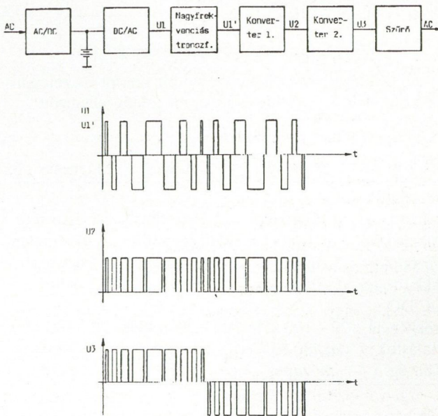
5. ábra. UPS nagyfrekvenciás transzformátorral
