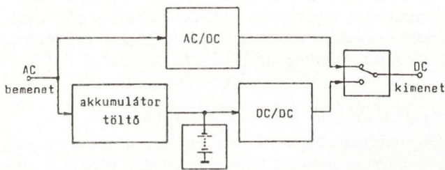
3. ábra. Standby UPS
