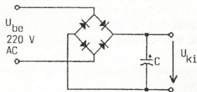
1. ábra. Tipikus tápegység-bemenőfokozat
