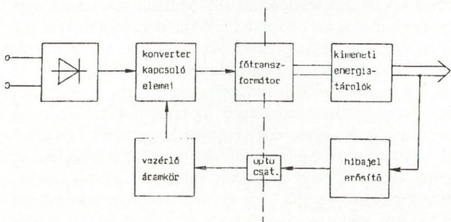
7. ábra. A hagyományos IBM tápegység blokkvázata
