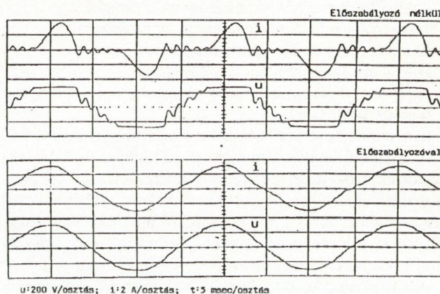
7. ábra. Időtartománybeli mérési eredmények
