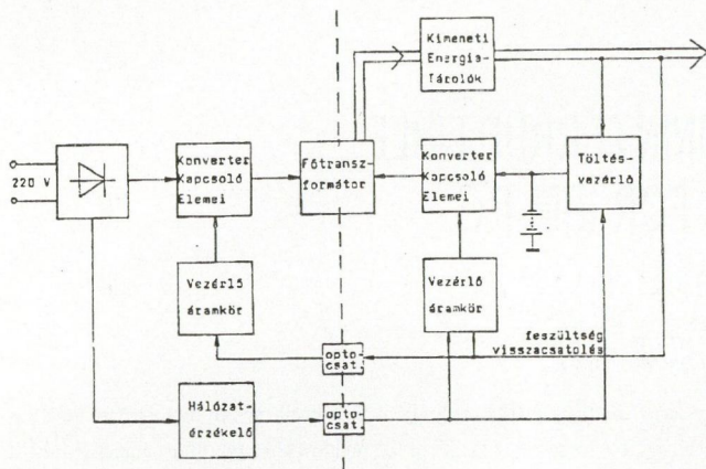
8. ábra. Az IBM PC DC UPS felépítése
