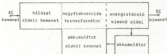
6. ábra. A mágneses alkatrészeiben összegző UPS
