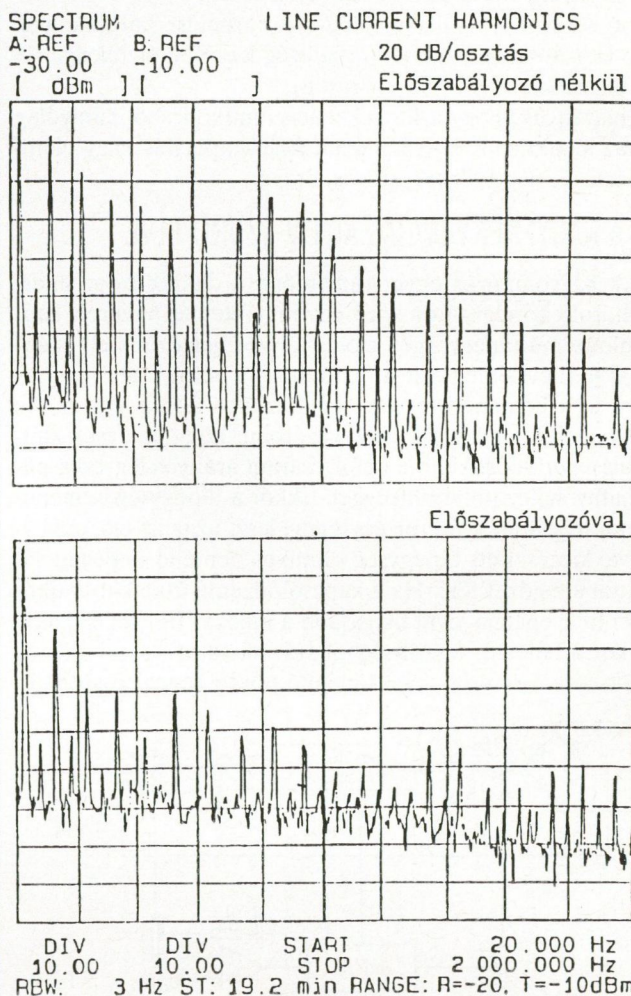
8. ábra. Frekvenciatartománybeli mérési eredmények
