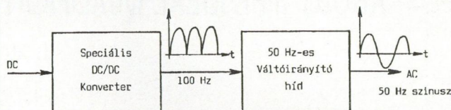
2. ábra. Tiszta elektronikus inverter
