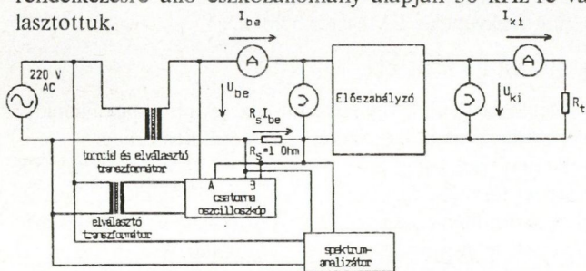
6. ábra. Mérési elrendezés
