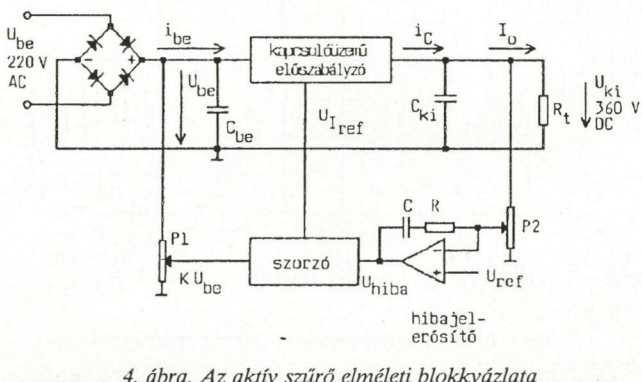
4. ábra. Az aktív szűrő elméleti blokkvázlata
