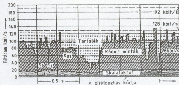
13. ábra. Az ISO/MPEG-Audio kód II. RÉTEG-ének tipikus bitáram-képe (hibavédelem nélkül). A pontozott rész azt a tartalékok mutatja, amely 128 kbit/s bitáramnál adódik.
