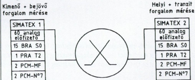
6. ábra. Tesztkonfiguráció
