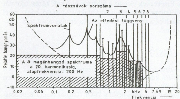
12. ábra. A 200 Hz alapprofrendenciájú a (angol) magánhangzó 20 harmonikusának spektruma és az abból számítható dinamikus elfedési görbe. A vonalkázott területre eső kvantálási zaj nem hallható (az annak megfelelő hangerő esetén).
