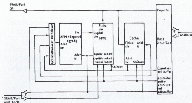
2. ábra. Az ARMProcessor blokkvázlata
