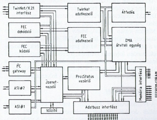
3. ábra. A MainMemoryController blokkvázlata
