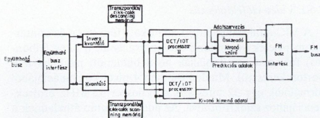
5. ábra. A Blockprocessor blokkvázlata
