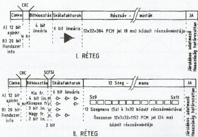
6. ábra. Az ISO/MPEG-Audio kód I. és II. RÉTEG-ének kimenő jelformátuma
