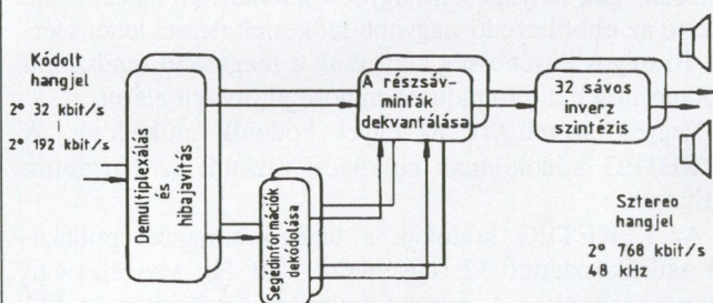
9. ábra. Az ISO/MPEG-Audio kód I. és II. RÉTEG-ének kétszámú dekódolója
