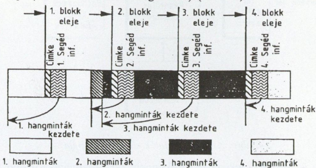
8. ábra. Az egyenetlenül terhelte blokkok terhelés-kiegyenlítése az ISO/MPEG-Audio kód III. RÉTEG-ének kódolójában
