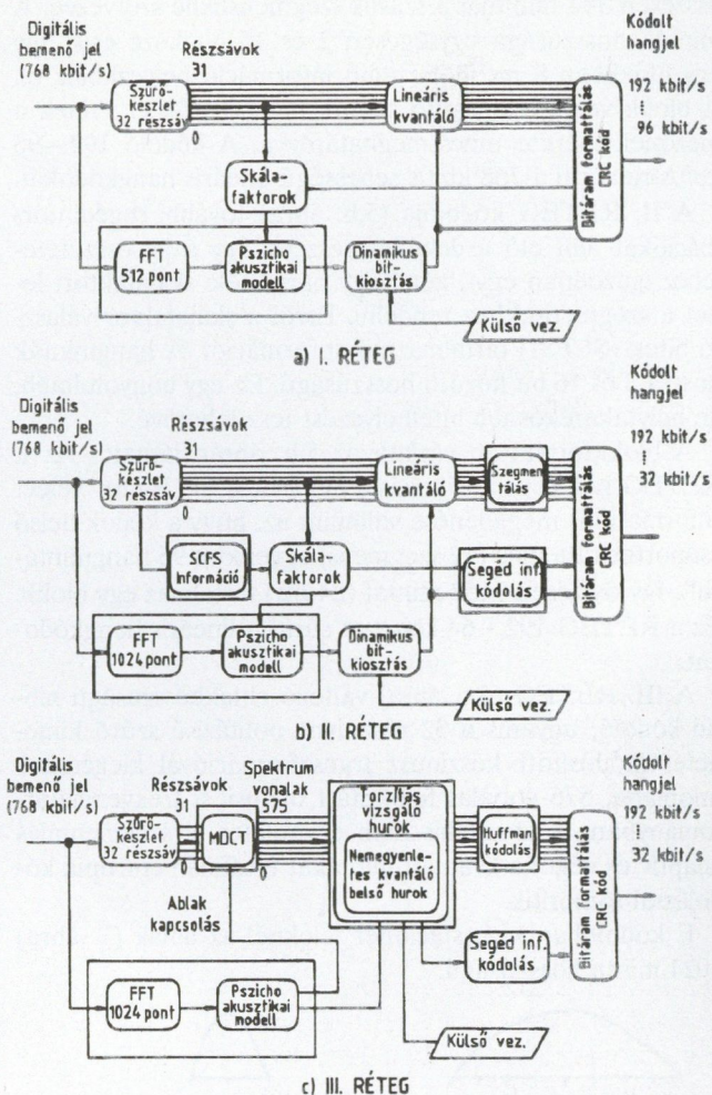
5. ábra. Az ISO/MPEG-Audio kód három rétegének kódolója (szóló csatorna). (A RÉTEG-ek közötti bővítéseket kettős kerettel jelöljük.)
