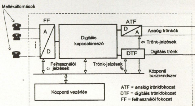
2. ábra. Harmadik generációs alközpont funkcionális felépítése
