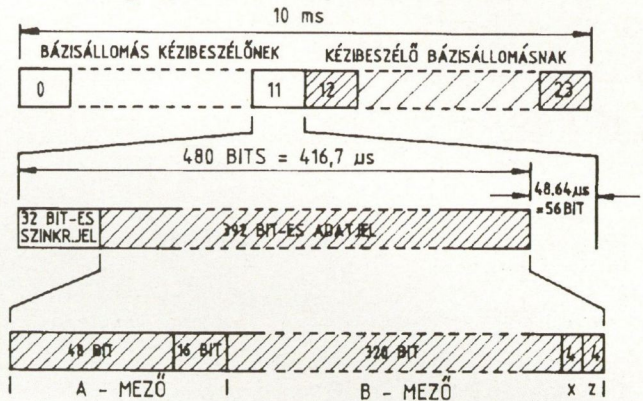
2. ábra. DECT TDMA adatsomagstruktúra
