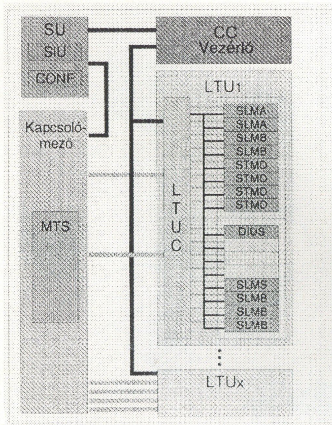
5. ábra. A kapcsolóegység felépítése
