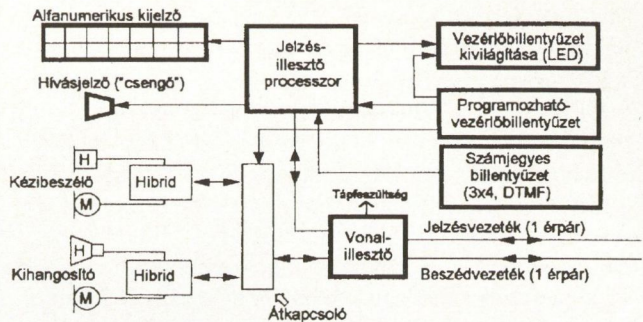
4. ábra. Rendszerkészülék funkcionális vázlata
