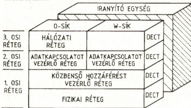
1. ábra. DECT rétegstruktúra
