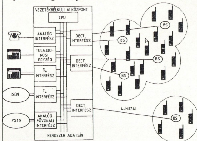
3. ábra. Első generációs vezetéknélküli alközpont tipikus konfigurációja
