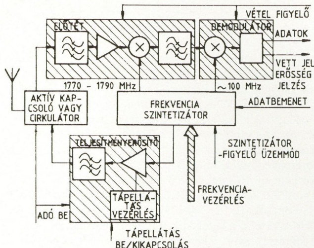
9. ábra. A DECT kézügytermínál rádiófrekvenciás részének alaparchitektúrája
