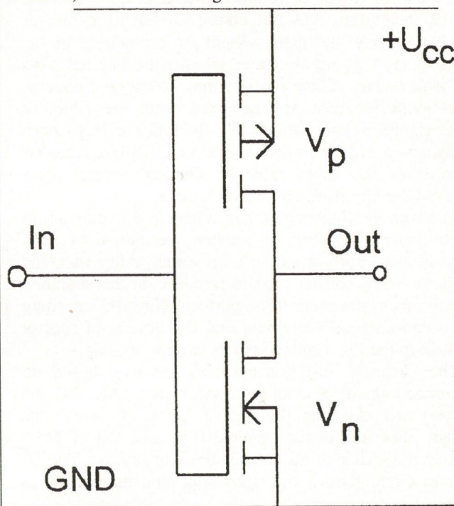
Fig. 1. A CMOS inverter
