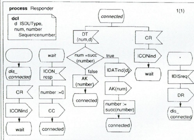
19. ábra. A Responder processz
