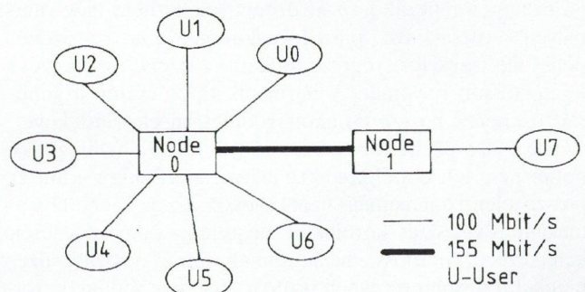
4. ábra. A szimulációs modell
