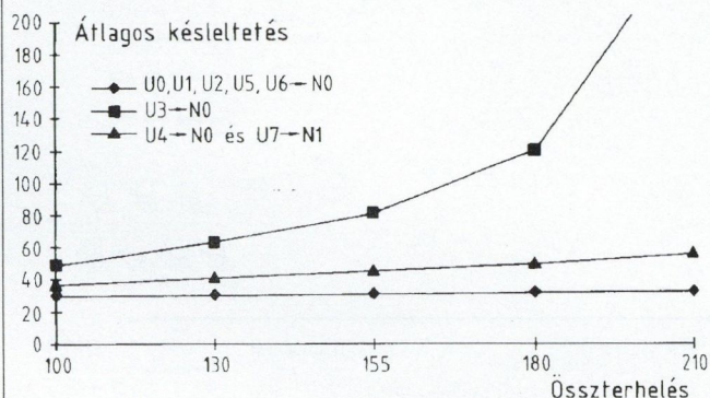
5. ábra. Összerhelés — átlagos késleltetés USER-NODE típusú linkek esetén
