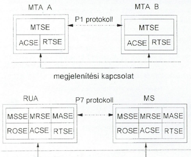
3. ábra. Az X.400-as protokollokat alkotó szolgálati elemek
