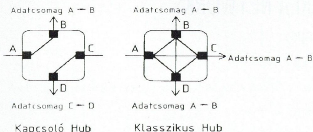
1. ábra. A kapcsoló és klasszikus hub egyszerűsített működési elve. a) kapcsoló hub; b) klasszikus hub
