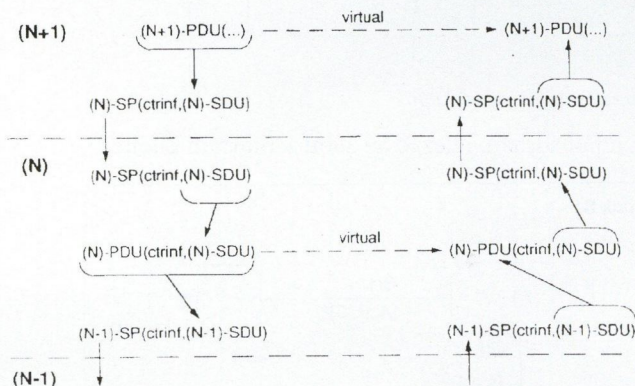
8. ábra. Kapcsolat a szolgálati primitívek (SP – Service Primitive), a szolgálati adatalemek (SDU – Service Data Unit) és a protokoll adatalemek (PDU – Protocol Data Unit) között
