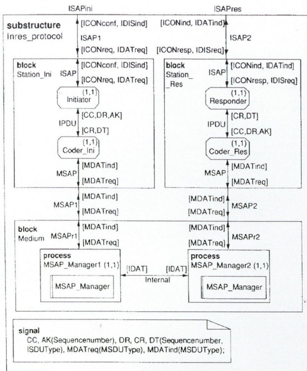
16. ábra. Az INRES protokoll specifikációja
