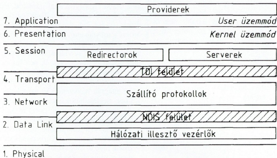
1. ábra. A Windows NT hálózati felépítése az ISO/OSI tükrében
