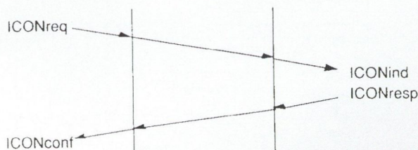
12a. ábra. Sikeres kapcsolatfelépítés
