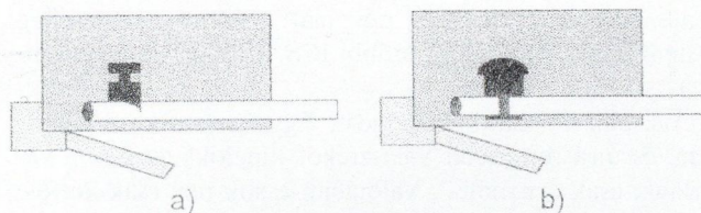
3. ábra. RJ45 típusú csatlakozó a) sokeres kábelhez; b) egyes kábelhez
