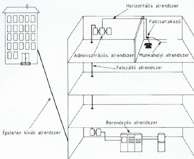
1. ábra. Strukturált hálózat felépítése
