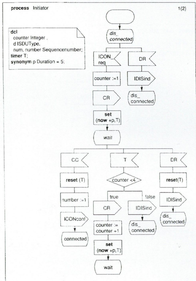
17. ábra. Az Initiator processz (1)
