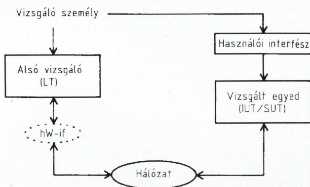
2. ábra. Alkalmazás vizsgálati elrendezés
