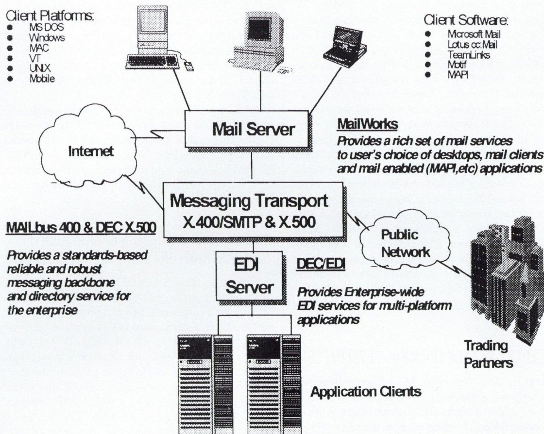
1. ábra. Digital Messaging Integration Framework szerkezete
