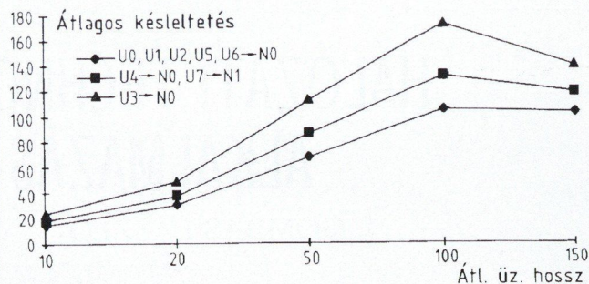
7. ábra. Átlagos üzenethossz — átlagos késleltetés USER-NODE típusú linkek esetén
