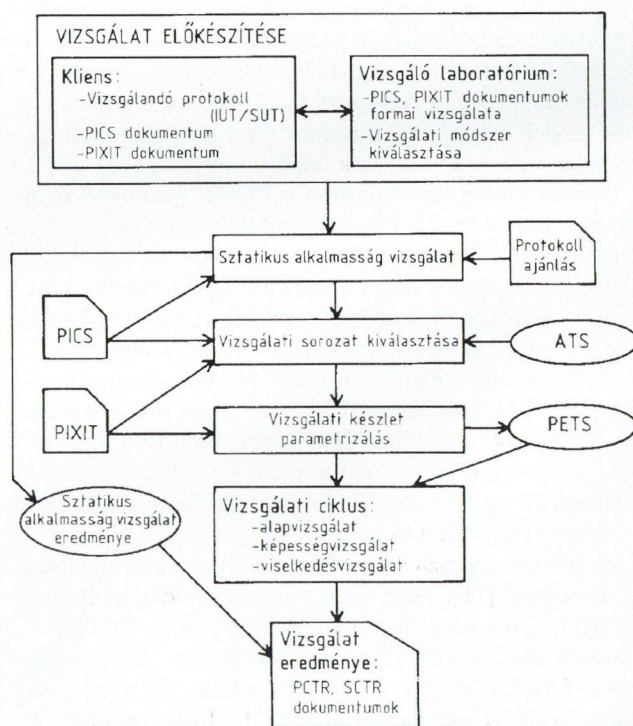
3. ábra. Alkalmasság vizsgálat
