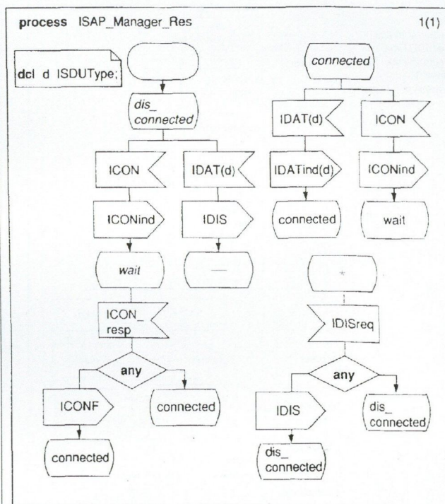
15. ábra. Az ISAP_Manager_Res processz
