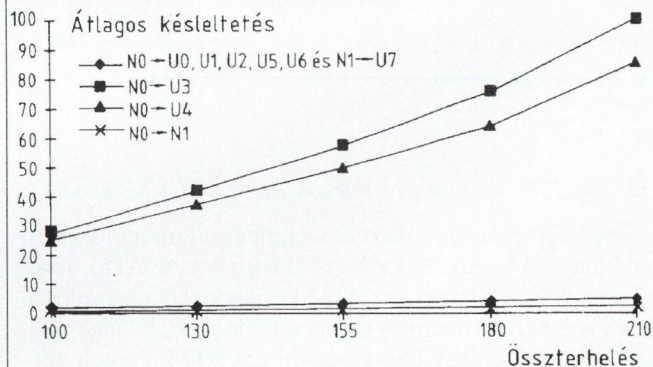
6. ábra. Összerhelés — átlagos késleltetés NODE-USER típusú linkek esetén
