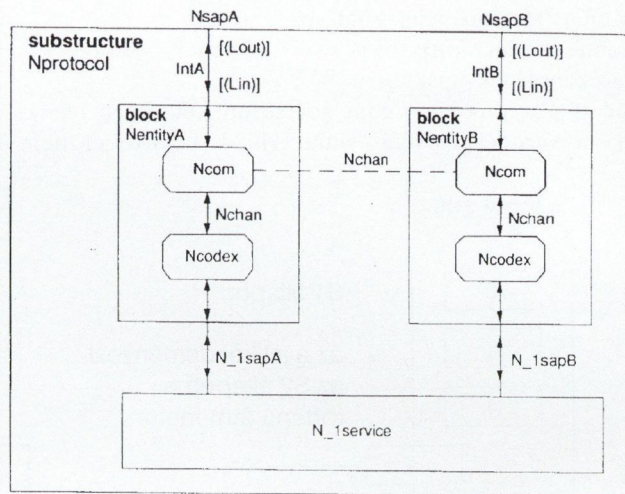
10. ábra. OSI protokoll SDL-beli specifikációja
