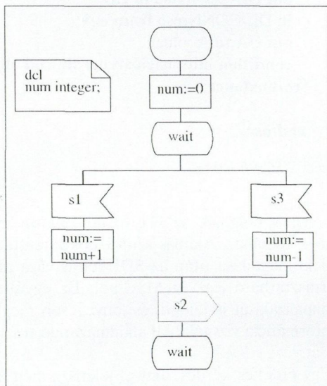
3. ábra. Példa SDL/GR és SDL/PR leírásra
