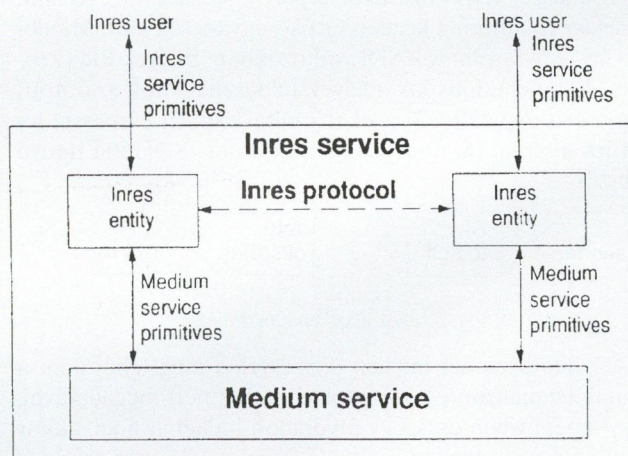
11. ábra. Az INRES rendszer felépítése
