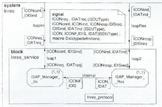
13. ábra. Az INRES rendszer
