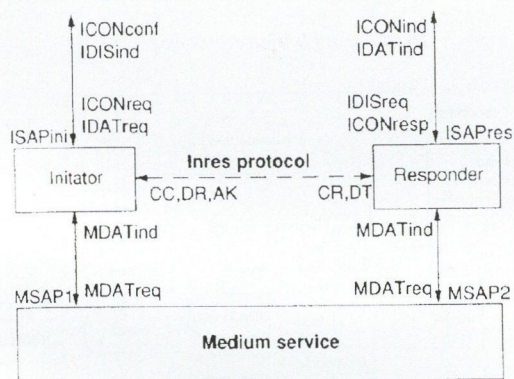
12d. ábra. Az INRES protokoll
