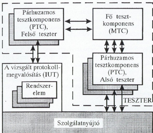
5. ábra. A többoldalú tesztelési módszer
