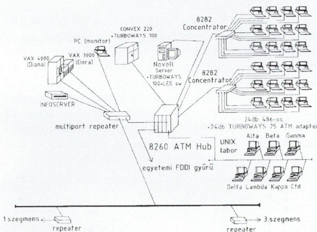
3. ábra. Példa az ATM gépészeti hálózatba történő bevonására
