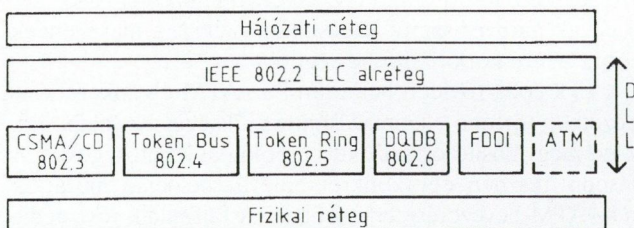
1. ábra. IEEE 802 LAN protokollok és az ATM MAC alréteg. DLL (Data Link Layer) — Adatkapcsolati réteg; LLC (Logical Link Control) — Logikai kapcsolatvezérlő
