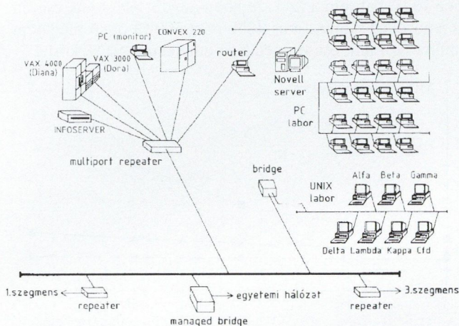
2. ábra. BME Gépészmérnöki kar számítógép-hálózatának vázlata
