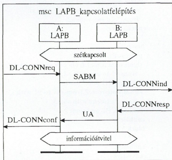
2. ábra. Példa MSC/GR diagramra és MSC/PR leírására
