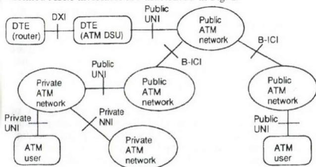
Fig. 1. ATM interfaces
