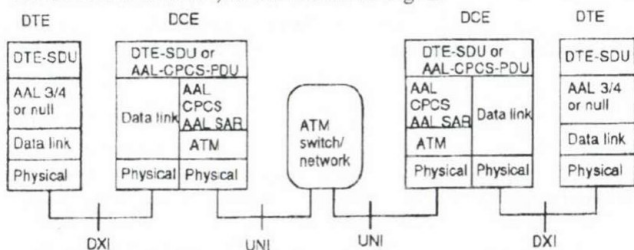
Fig. 2. DXI framework
