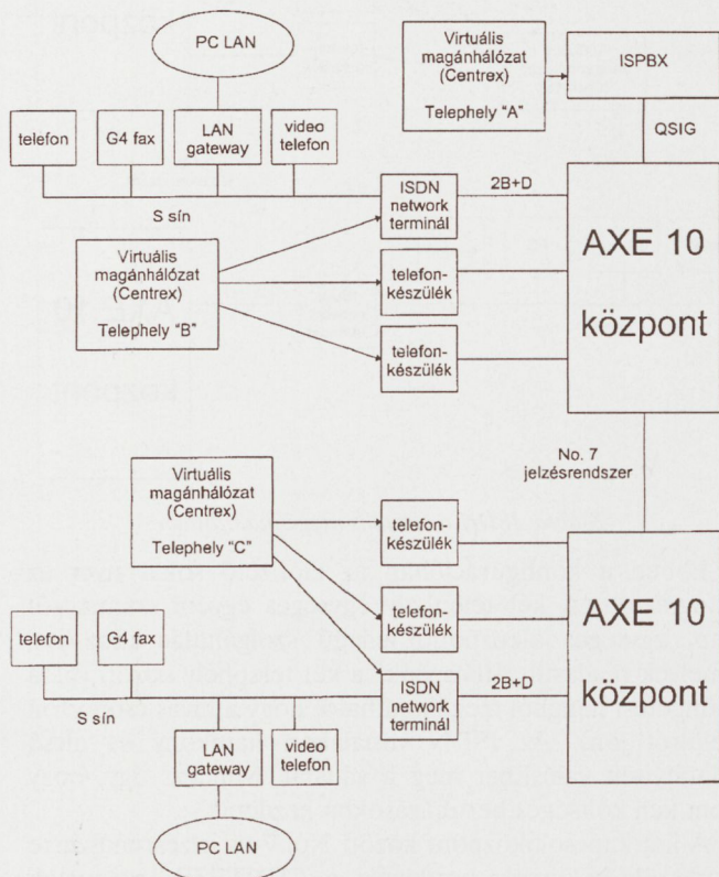
3. ábra. ISDN a virtuális magánhálózatban — többszállítós környezet
