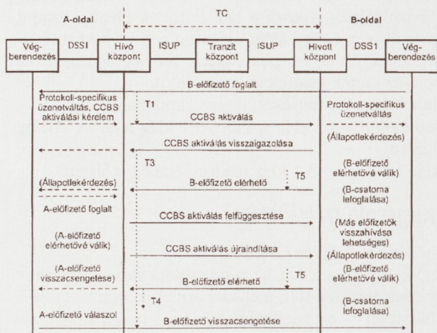
1. ábra. Üzenetváltások a központok és a végberendezések között (funkció-protokoll esetén)
