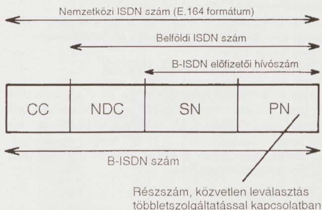
3. ábra. A B-ISDN hívószám szerkezete CC: Országjelölő kód (Country Code); NDC: Nemzeti rendeltetési cím (körzetszám) (National Destination Number); SN: Előfizetői hívószám (Subscriber Number); PN: Részszám (Partial Number)
