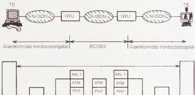
6. ábra. Áramkörmódú hordozószolgáltatási együttműködés, B-ISDN-en keresztül
