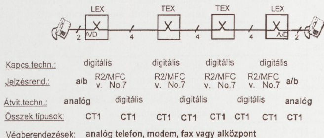
1. ábra. A digitalizált távbeszélő-hálózat
