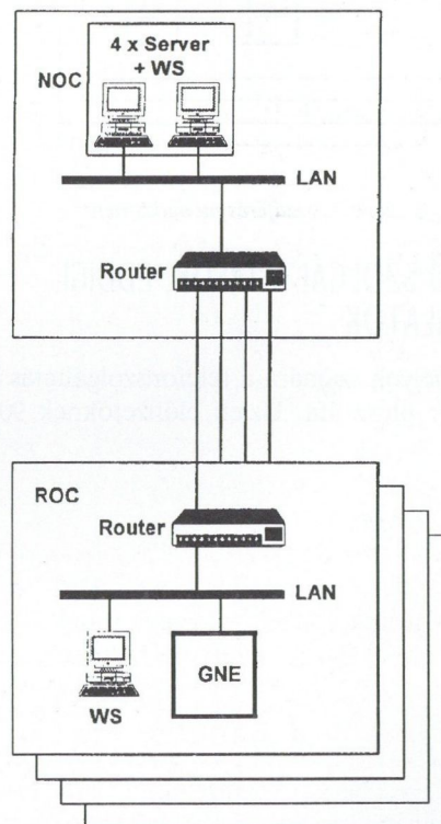
2. ábra. Átviteltechnika menedzsment
