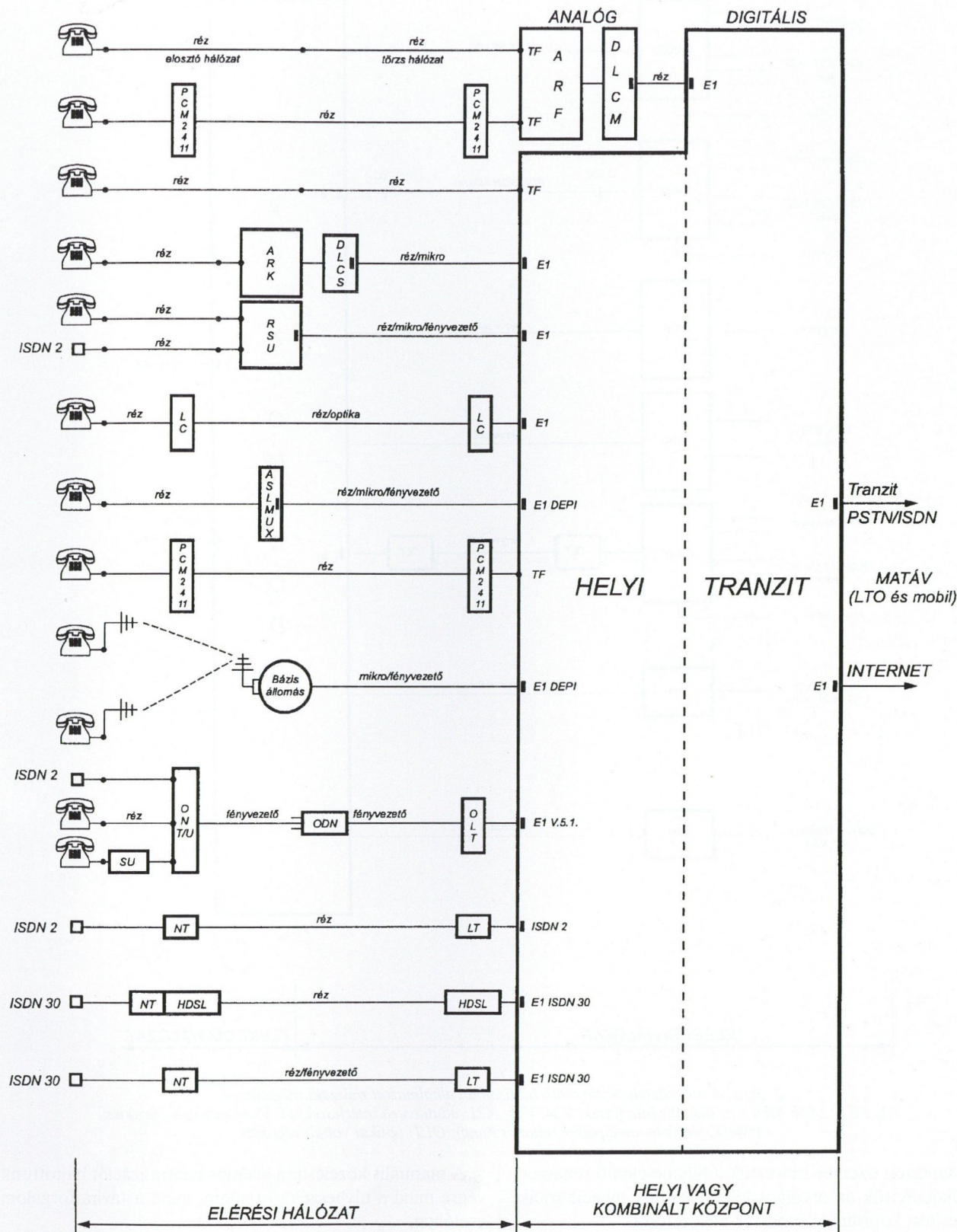
1. ábra. Távközlő- és ISDN-hálózati megoldások a Matáv szolgáltatási körzeteiben DLCM és DLCS: AR központokhoz kifejlesztett digitális vonalcsatlakozók; LC: vonali koncentrátor; ASLMUX: előfizetői PCM multiplex; OLT, ODN, ONT/U, SU: optikai elérési hálózat elemei; NT, LT: ISDN vonali végződések; HDSL: nagysebességű digitális vonali rendszer; E1: 2,048 Mbit/s-os digitális interfész; TF: hangfrekvenciás interfész; DEPI, V5.1: digitális 30 csatornás interfészek
