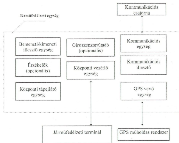
4. ábra. A járműfedélzeti egység belső felépítése
