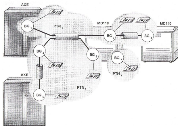
8. ábra. Al- és főközpontokkal megvalósított centrex-hálózat
