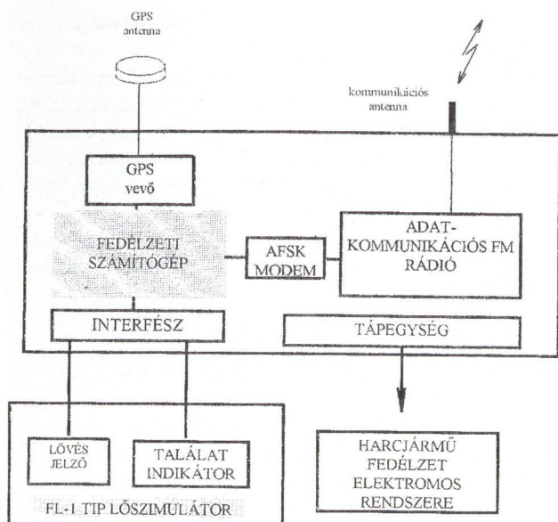
2. ábra. Harcjármű-fedélzeti egység blokksémája
