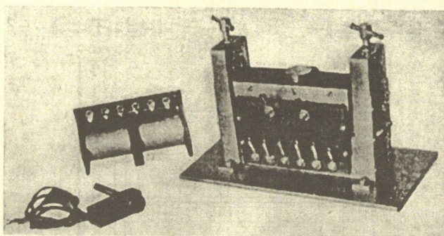
5. ábra. A nagy iga fényképe. Az iga felső részén az iránytű látható. Középen egy hozzátartozó tekercs van, melynek középső válaszfalában látható a furat a baloldali, csőbeszerelt iránytű részére.
