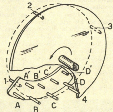
6. ábra. Forgó szikraköz.
