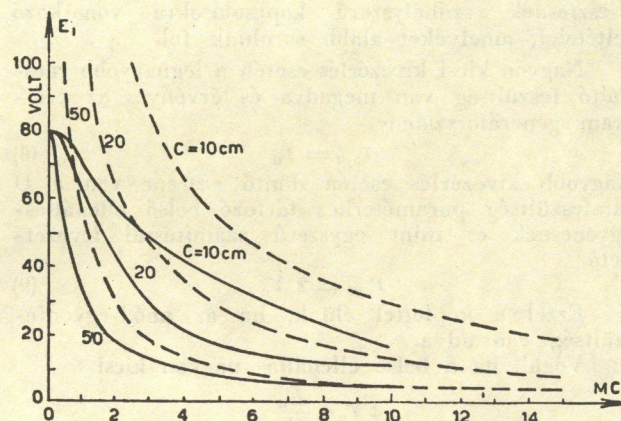
6. ábra. A megengedett legnagyobb bemenő feszültség a frekvencia függvényében 6AC7 ill. EFF50 csőnél, 10.000 Ohm katódelőellenállással, különböző kimenő kapacitások esetében. A kihúzott görbék trióda, a szaggatott görbék pentóda kapcsolásra vonatkoznak.
