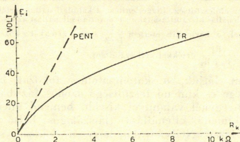
4. ábra. A megengedett legnagyobb bemenő feszültség a külső ellenállás függvényében 6AC7 ill. egyik EFF50 rendszer esetén. A kihúzott görbe trióda, a szaggatott görbe pentóda kapcsolásra vonatkozik.
