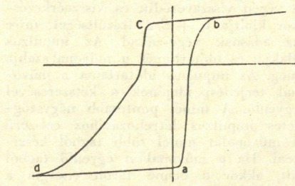
11. ábra. A vasmagos modulátortekercs mágneszési görbéje Peterson szerint 2)
