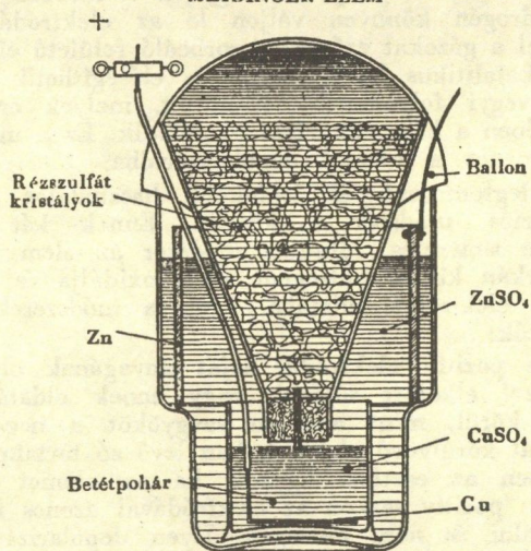
MEIDINGER ELEM
