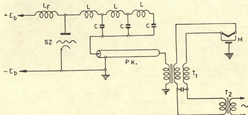
4. ábra. Művonalas modulátor elvi áramköre.
