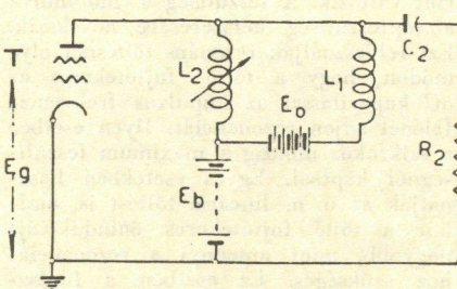
9. ábra. Vasmagos tekercs-modulátor elvi kapcsolása
