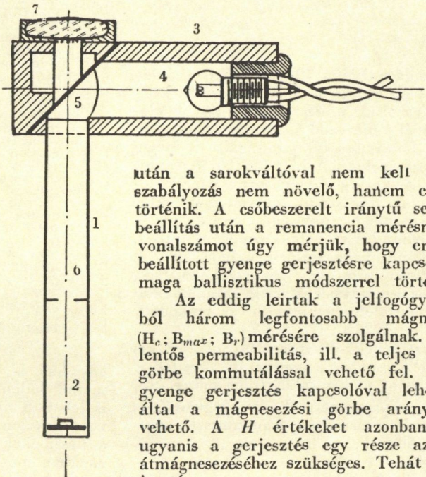
11. ábra. Csőbeépített iránytű, szerkezet az igazi remanencia méréséhez
