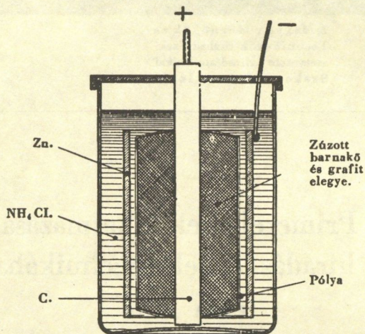
ZACSKÓS ELEM
