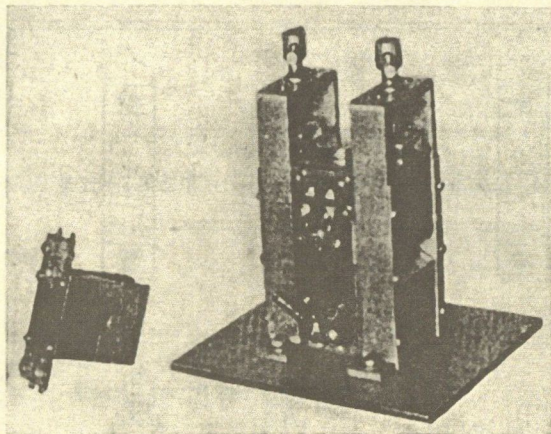
6. ábra. A kis iga fényképe. Jobboldalt az iga, baloldalt egy hozzátartozó tekercs van.
