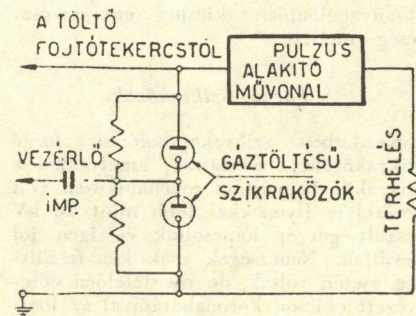
7. ábra. Sorbakapcsolt gáztöltésű szikraközzök begyújtása vezérlő feszültséggel.
