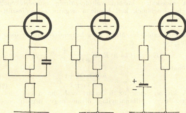
3. ábra. Az előfeszültség függetlenítése a katóddenállás értékétől. A bemenő ellenállás kiszámításánál a rácslevezető ellenállást az első esetben névértékével, a harmadik esetben \frac{1}{1-A} szoros értékkel a középső esetben \frac{1}{1-A} \cdot \frac{R_1}{R_1 + R_2} értékkel kell számítani.
