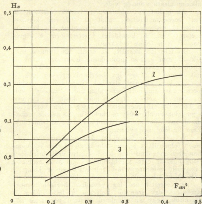
7. ábra. Bemért igakorrekciók a próbakeresztmetszet és az anyag függvényében a nagy igára. 1 = avédvas; 2 = Si-vas; 3 = permalloy.
