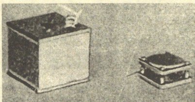
4. ábra Sávszűrő-tekeres vas-nikkel és „Ferroxcube”-maggal.
