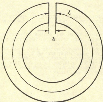
2. ábra. Légrés mágneses körben.
