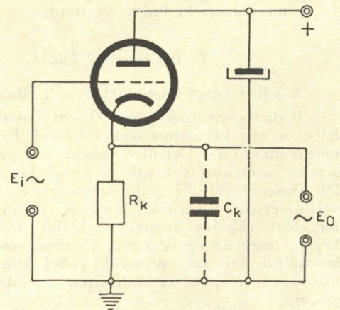
1. ábra. A katódcsatolás elvi kapcsolása.
