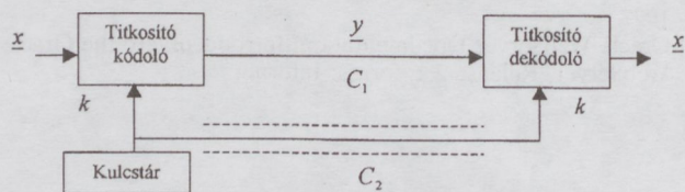
1. ábra. konvencionális titkosító blokkvázlata
