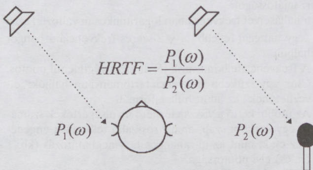
6. ábra. A (monaurális) HRTF mérési elve
