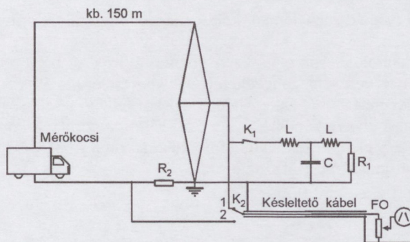
10. ábra. A lökőfeszültség vizsgálat és mérésnek elrendezése
