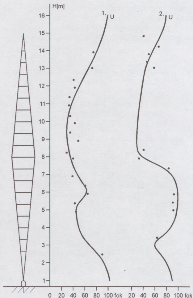
6. ábra. A mért feszültségeloszlás alakulása a sima modellen és a földelt kialakításban
