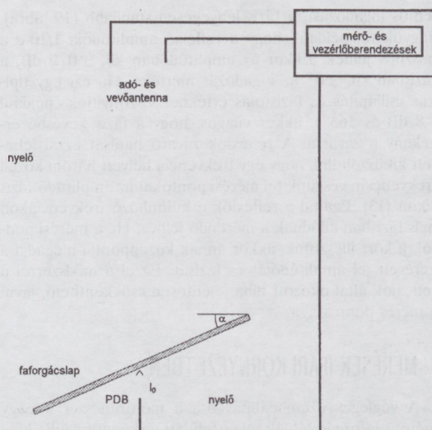
18. ábra. A laboratóriumi mérési elrendezés
