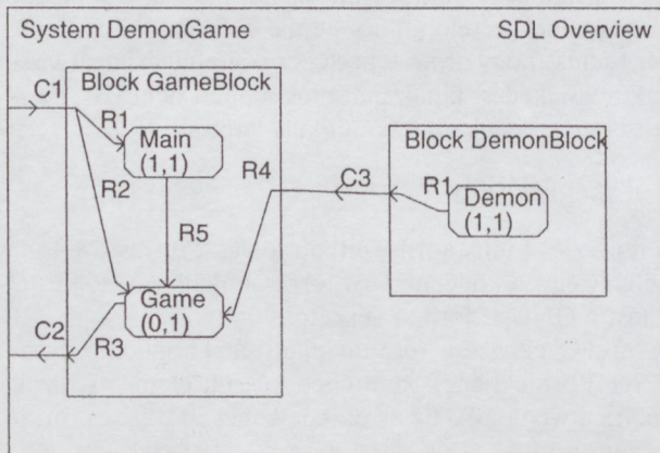
4. ábra. A Demon Game játék specifikációjának áttekintő nézete SDL/GR-ben
