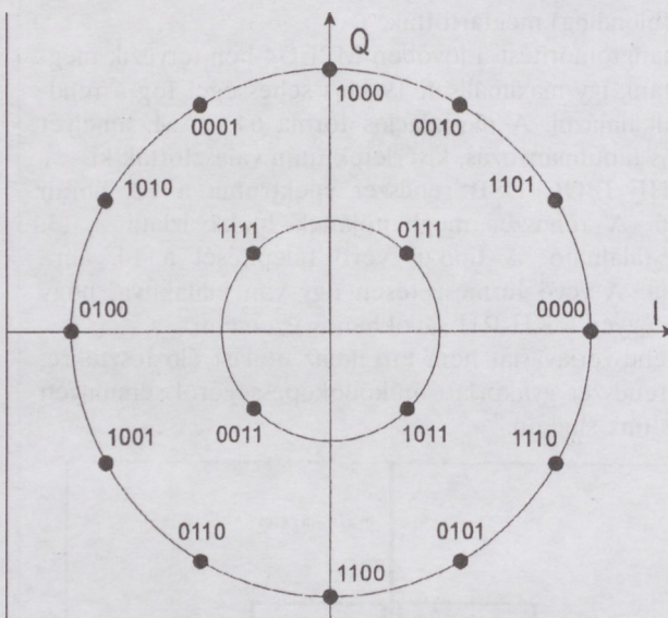
18. ábra. Az alkalmazott 16 APSK moduláció diagrammja
