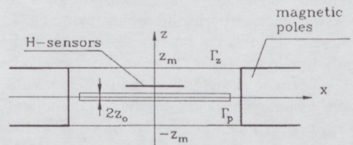
7. ábra. Hatszög alakú próbatest forgó mágneses térbeli viselkedésének elemzésére szolgáló térszámítási modell
