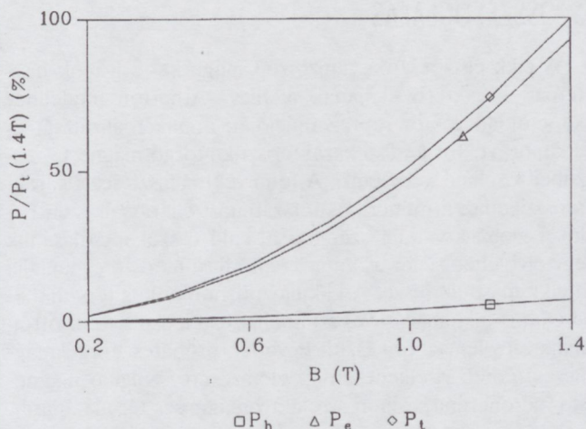
22. ábra. Hengerlés irányába mutató szinuszosan változó mágneses indukcióval való gerjesztés esetén a histerézis P_h , az örvényáram P_e és a teljes P_t veszteség alakulása különböző indukció értékek mellett
