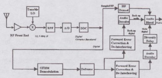
14. ábra. A tipikus vevő felépítése
