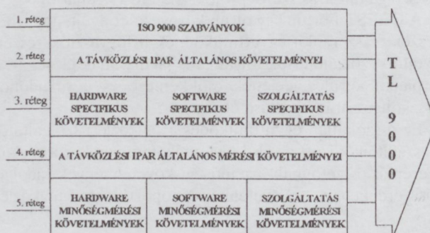
1. ábra. A QuEST által vizsgált terület
