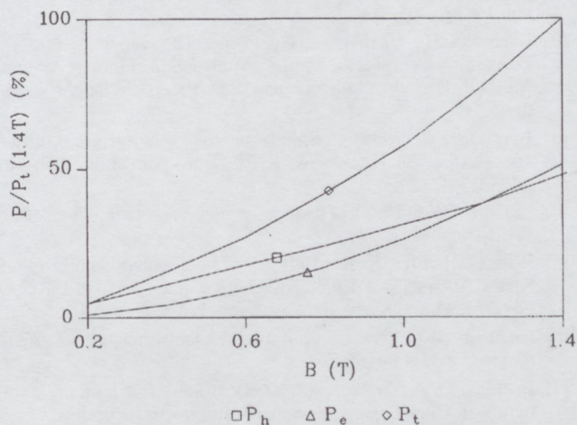
23. ábra. Hengerlés irányára merőleges irányba mutató szinuszosan változó mágneses indukcióval való gerjesztés esetén a histerézis P_h , az örvényáram P_e és a teljes P_t veszteség alakulása különböző indukció értékek mellett
