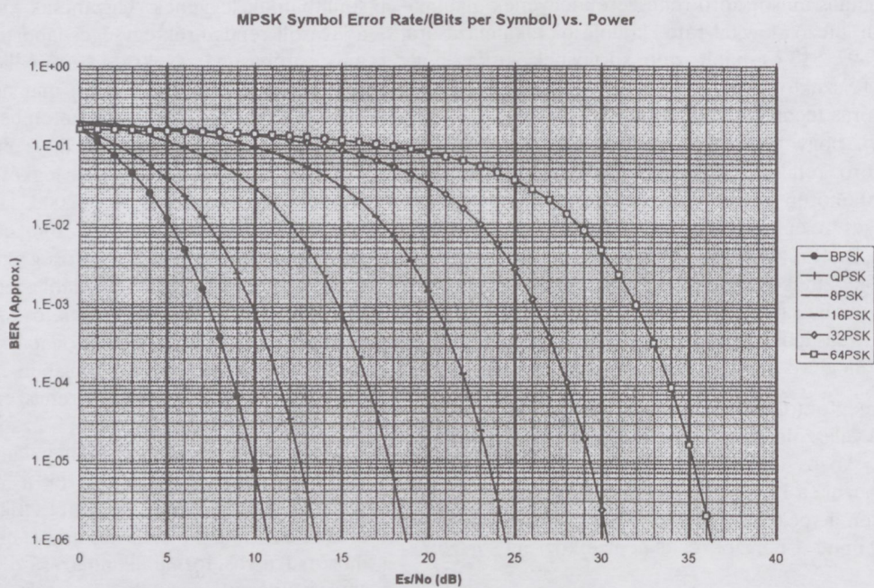
1. ábra. Hozzávetőleges bit-hibarány értékek különböző MPSK változatoknál
