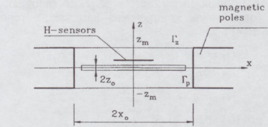
6. ábra. Négyyszög alakú próbatest forgó mágneses térbeli viselkedésének elemzésére szolgáló térszámítási modell
