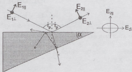
1. ábra. A Brewster-szögben beeső hullám visszaverődése
