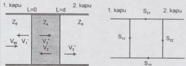
2. ábra. A vizsgált anyagminta mint kétkapu
