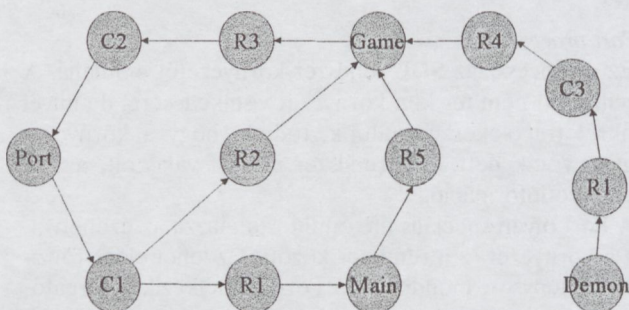
3. ábra. A Demon Game játék CG szerkezete
