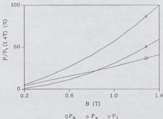
24. ábra. A mágneses indukció körkörösán polarizált átlagértéke mellett, forgó indukciójú mágneses gerjesztés esetén a histerézis P_h , az örvényáram P_e és a teljes P_t veszteség alakulása különböző indukció értékek mellett
