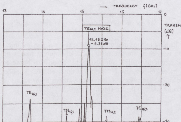
Fig. 13. Mode filtering using irices: 1.8^\circ - 1.8^\circ - 3.6^\circ
