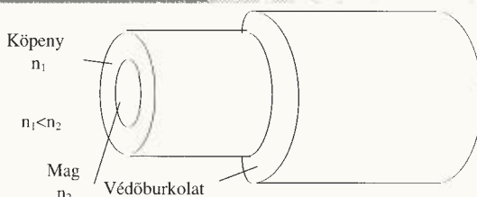
1. ábra . A szál szerkezete
