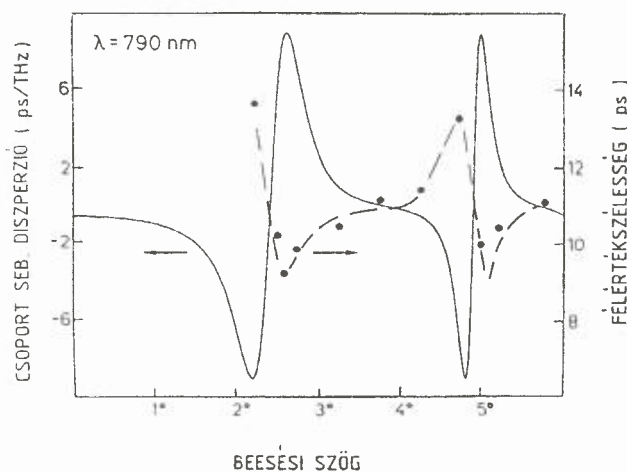
17. ábra. A Gires–Tournois interferométer által generált csoportsebesség diszperzió és az autokorrelációs függvény félértékszélessége (fekete pont) a beesési szög függvényében
