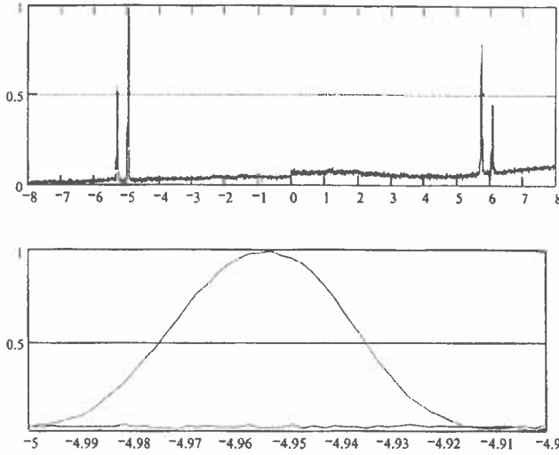
16. ábra. A detektált módus-spektrum, valamint egy rezonancia csúcs kinagyított képe (normalizált intenzitás a szöghelyzet függvényében [°])
