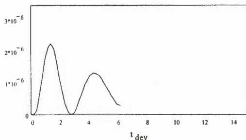
12. ábra. Holografikus rácselekhívási görbéje (a detektor fotoárama [A] a hívási idő [sec] függvényében)
