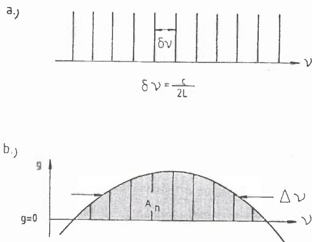
2. ábra. Fabry–Perot rezonátor longitudinális móduseloszlása (a) és a módusok erősítő közeg által meghatározott amplitúdóeloszlása; (b) az erősítés félértékessége
