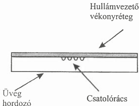
6. ábra. A rács-csatolóval ellátott optikai hullámvezető felépítése
