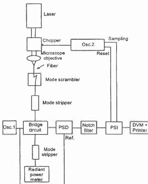
3. ábra. Kaloriméter mérőrendszer blokkvázlata
