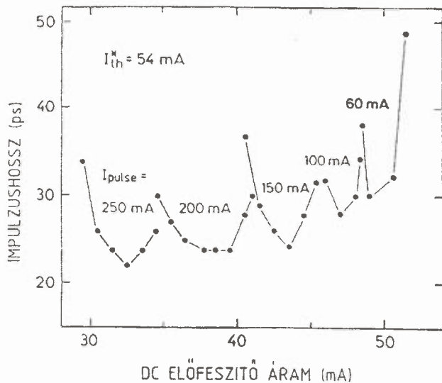
12. ábra. Az erősítés maximumánál ( \lambda = 824 \text{ nm} ) mért impulzushosszak az előfeszítő áram függvényében, különböző I_{\text{pulse}} amplitúdójú áramimpulzusokkal történő moduláció esetén. A lézerciódá külső rezonátorban mért küszöbárama I_{\text{th}}^* = 54 \text{ mA}
