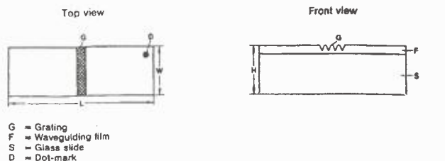
3. ábra Az ASI AG. által gyártott ASI 2400 típusú rács-csatolóval ellátott optikai hullámvezető szenzor (G: optikai rács-csatoló, F: hullámvezető réteg, S: üveg hordozó, D: front-felület jelölése)
