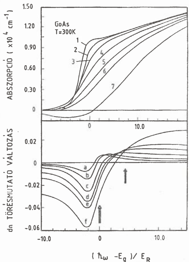
13. ábra. GaAs számított abszorpció spektruma különböző töltéshordozó koncentráció esetén [(1) 10^{15} , (2) 8 \times 10^{16} , (3) 2 \times 10^{17} , (4) 6 \times 10^{17} , (5) 10^{18} , (6) 15 \times 10^{18} , (7) 2 \times 10^{18} \text{ cm}^{-3} ], valamint a spektrum eltolódásából Kramers – Kronig transzformációval meghatározott törésmutató változás [24] alapján. Az a jelű görbe \alpha(1) - \alpha(2) , a b jelű \alpha(1) - \alpha(3) , ... stb. abszorpció változáshoz tartozik. A vízszintes tengelyen E_g = 1,42 \text{ eV} és E_R = 4,2 \text{ meV}
