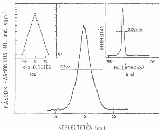
16. ábra. Móduszszinkronizált impulzus spektruma és a nemlineáris kristályban keltett második harmonikus fény intenzitásával mért autokorrelációs függvénye
