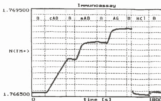
5. ábra Az IOS-1 készülékkel detektált szenzogram. (az effektív törésmutató időbeli változásának görbéje)
