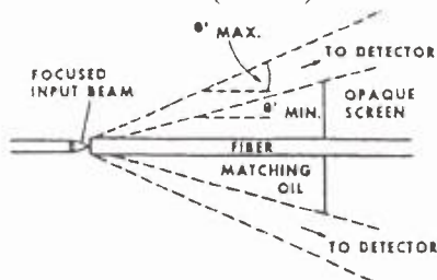
7. ábra. Refraktált közeltéri mérési módszer elvi vázlata
