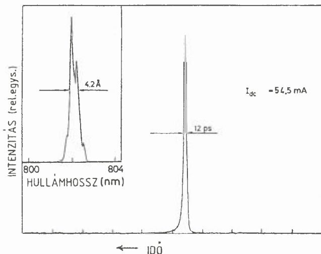
10. ábra. Streak kamera felvétel és az emisszió spektruma 802 nm-en
