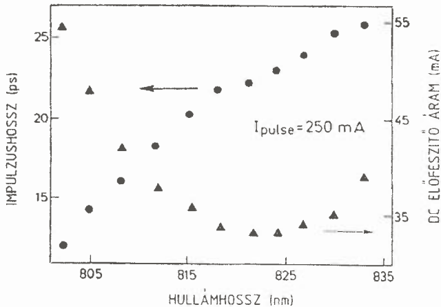
8. ábra. Az impulzusidőtartam mért értékei (fekete pontok) és a hozzátartozó optimális egyenáramértékek (háromszögek) a hullámhossz függvényében. Az eredeti lézeremisszió hullámhossza 824 \text{ nm} .
