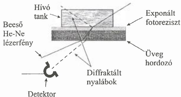
11. ábra. A reziszt réteg monitorozott hívására alkalmas összeállítás
