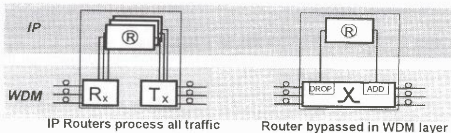
3. ábra. Az a) eset olyan pont–pont WDM rendszert mutat, ahol minden csomag áthalad az R routeren. A b) eset olyan csomópontot ábrázol, ahol a WDM réteg lehetőséget nyújt az R router kikerülésére.
