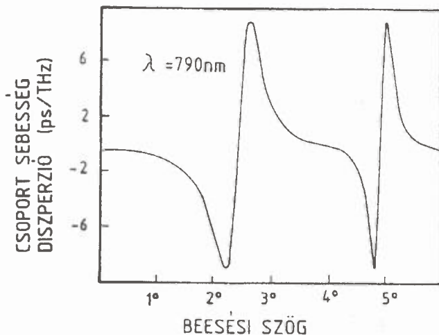
14. ábra. A Gires–Tournois interferométer csoportsebesség diszperziójának számolt értékei különböző beesési szögek esetén
