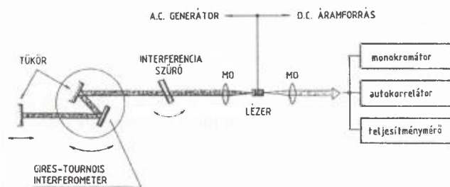
15. ábra. A Gires–Tournois interferométerrel kiegészített külső rezonátoros mérés sematikus rajza (MO: mikroszkópobjektív)
