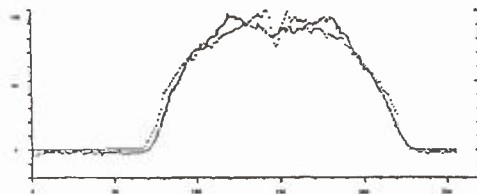
8. ábra. Szál törésmutató eloszlások összehasonlítása
