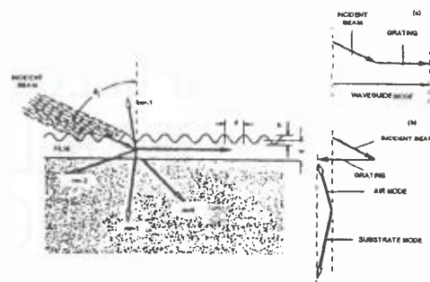
11. ábra. Rács-csatolású szenzor
