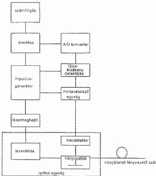
2. ábra. OTDR blokkvázlata
