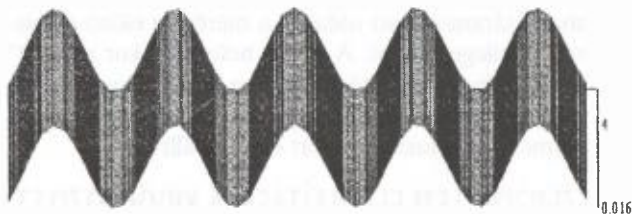
7. ábra. He–Cd lézer 441,6\ \text{nm} nyalábjainak 70^\circ -os szög alatti interferenciájakor kialakuló mező intenzitás-eloszlása (az intenzitás-eloszlás helyfüggése)
