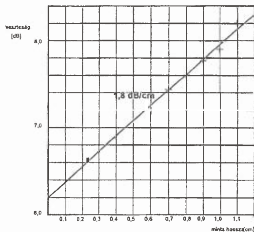
9. ábra. Integrált optikai elem csillapítása
