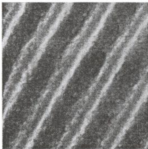
14. ábra. elektronmikroszkópos felvétel egy előhívott, arannyal bevont fotoreziszt rácstről
