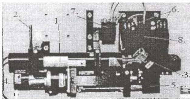
2. ábra. IOS-1 típusú készülék optomechanikai egysége. (A számokkal jelölt alkatrészek a következők: 1.: He–Ne lézer, 2.: polarizáció-állító, 3.: terelő tükör, 4.: léptető motor 5.: szöghelyzet pozícionáló asztal, 6.: detektorok 7.: mérendő folyadék-, ill. gázkezelő, 8.: rács-csatolóval ellátott optikai hullámvezető szenzor (küvettként kialakított tartó belsejében)
