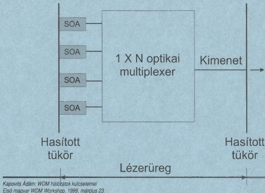
33. A sokfrekvenciás lézer (MFL) sematikus felépítése
