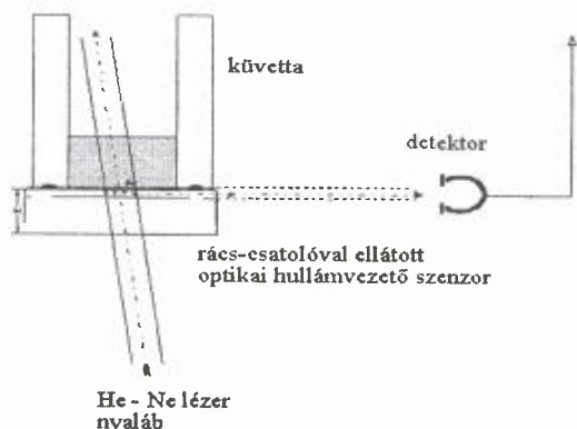
4. ábra. A He-Ne lézernyaláb sugármenete az érzékelő térfogatban
