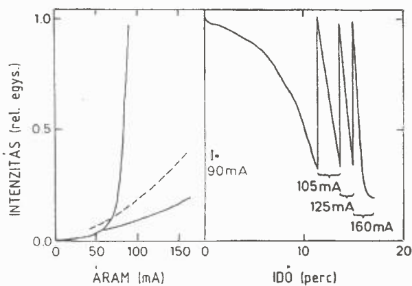
6. ábra. Lézerdióda fénytéljesítmény-áram karakterisztikája a porlasztási folyamat előtt és után, valamint az in-situ mért intenzitás a porlasztás idejének függvényében
