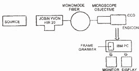
5. ábra. Közeltéri eloszlásmérő
