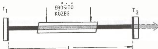
1. ábra. L hosszúságú Fabry—Perot lézer sematikus felépítése ( T_1 , T_2 : tükrök)
