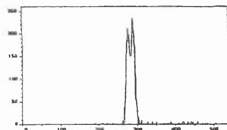
6. ábra. Egymódusú szálak közeltéri eloszlása
