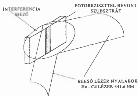
8. ábra. A holografikus exponálás felvételi elrendezésének vázlata
