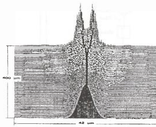
10. ábra. Y tag optikai téreloszlása
