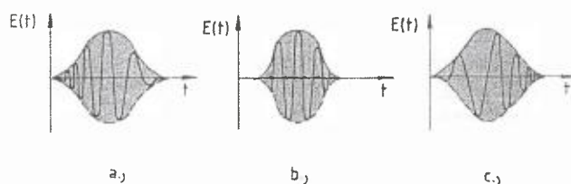
4. ábra. Impulzus elektromos terének amplitúdóváltozása (a) „down-chirp”, (c) „up-chirp” (b) „chirpmentes” esetben
