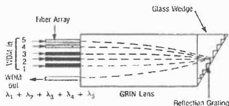
15. ábra. Hagományos optikai elemekből kialakított WDM nyaláboló
