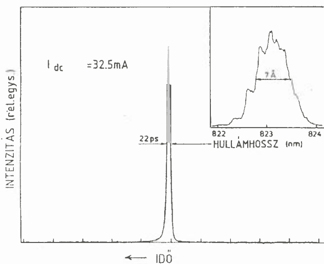
9. ábra. Streak kamera felvétel és az emisszió spektruma 824 nm-en
