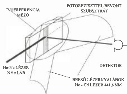
9. ábra. A holografikus exponálás felvétel közben történő monitorozásának vázlata
