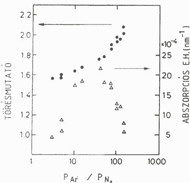
5. ábra. Porlasztott szilíciumnitrid réteg törésmutatójának (fekete pontok) és abszorpciós együtthatójának (háromszögek) változása a nitrogén parciális nyomásának függvényében
