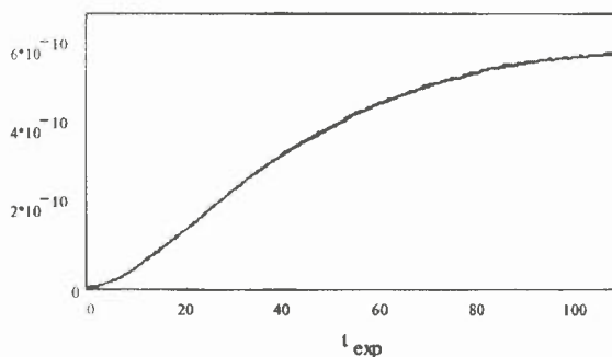
10. ábra. Egy holografikus rács exponálódási görbéje (a detektor fotoárama [A] az exponálási idő [sec] függvényében)
