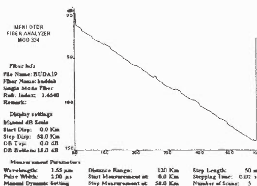
1. ábra. OTDR mérési görbe
