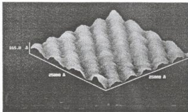
13. ábra. STM felvétel egy előhívott, arannyal bevont fotoreziszt rácstről
