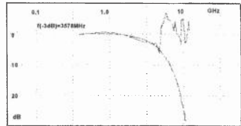
4. ábra. Az időtartományú diszperziós mérésekből számolt átviteli függvény
