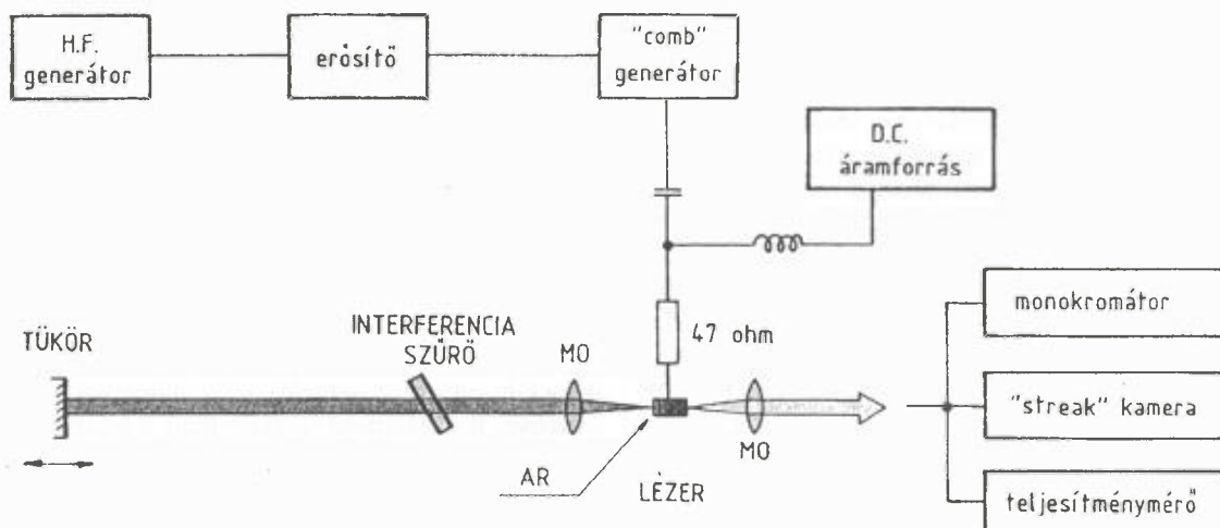
7. ábra. A külső rezonátor felépítése, a lézervediódára szolgáló elektronika kapcsolási vázlata és a fényimpulzusok mérésére szolgáló összeállítás (MO: mikroszkópobjektív, AR: antireflexiós réteg)
