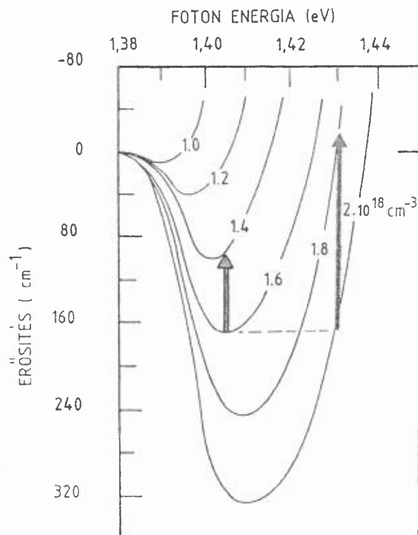
11. ábra. GaAs alapú lézerdíóda erősítése a kibocsátott foton energiájának függvényében, különböző töltéshordozó koncentráció esetén [7]
