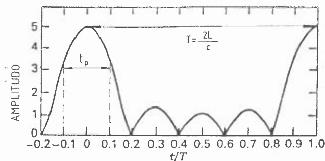
3. ábra. A sugárzási tér amplitúdójának időbeli változása módusszinkronizáció esetén (1.1 függvény, N = 5 , \alpha = 0 )
