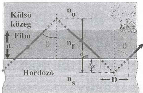
1. ábra. Sugármenet egy vékonyréteg hullámvezetőben
