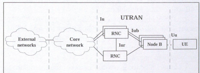
1. ábra UMTS hálózati architektúra
