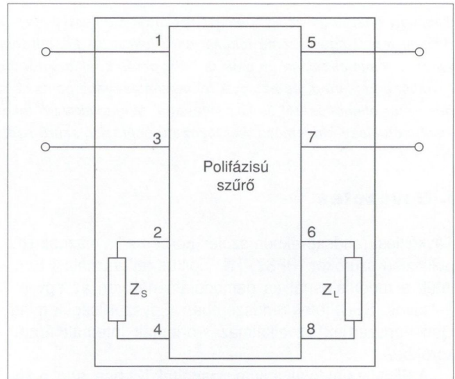
3. ábra A kétkapu, melynek zajtényezőjét meghatározzuk. Z_S és Z_L a külső lezárásokkal egyezik meg.
