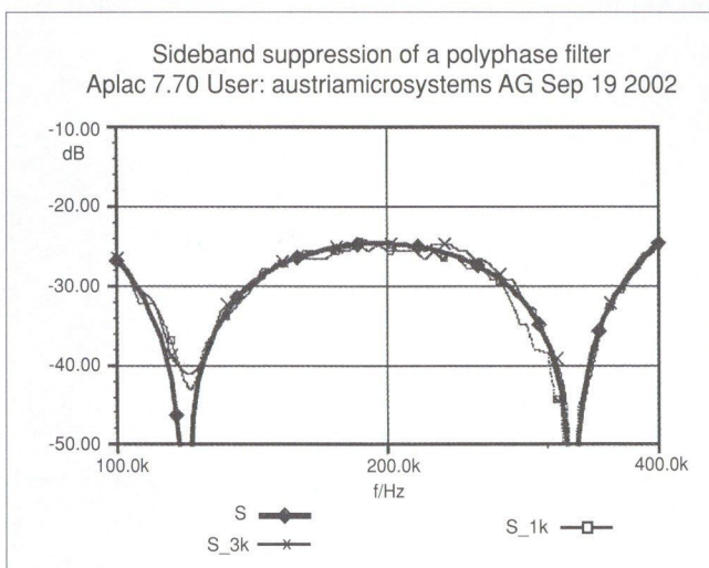
10. ábra Két fokozatú PFSZ elméleti (S) és mért (S_1k, S_3k) oldalsáv-elynomása
