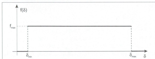
3. ábra A legjobbnak bizonyult (egyenletes eloszlású) sűrűségfüggvény
