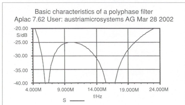
7. ábra A zajillesztett szűrő oldalsáv-elnyomása
