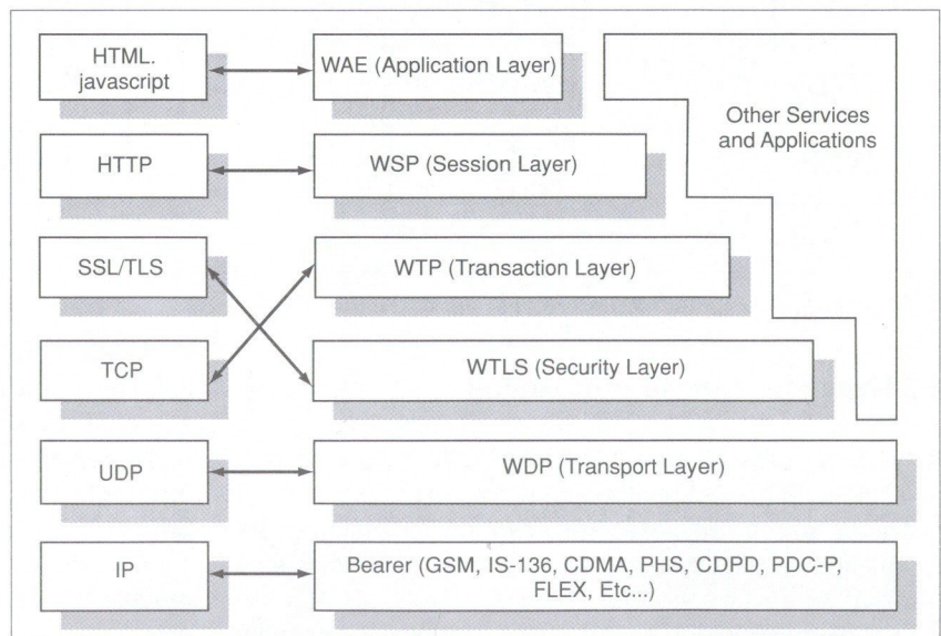
1. ábra TCP/IP protokollok és WAP megfelelőik
