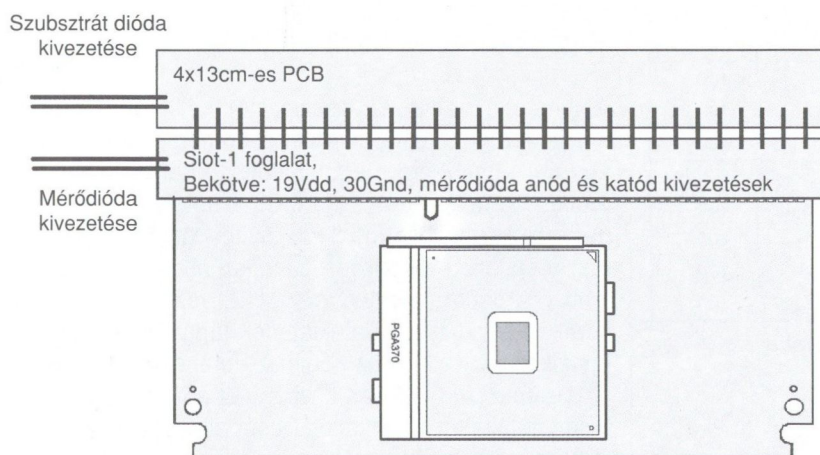
2/b A processzor és a PCB elrendezése
