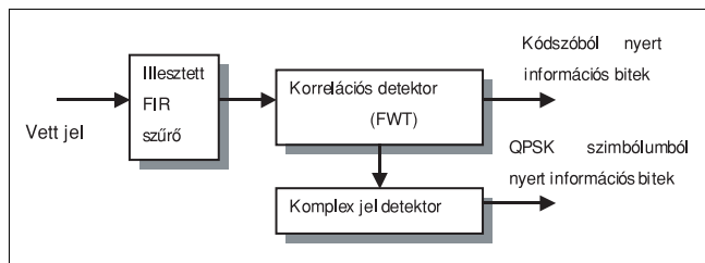
CCK moduláció, vevő áramkör elvi felépítése
