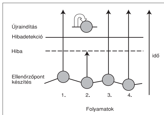
2. ábra Nem koordinált ellenőrzőpont-állomány készítés
