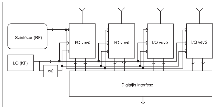
10. ábra: A hardver felépítése
