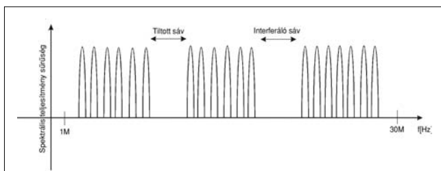
2. ábra OFDM moduláció spektruma
