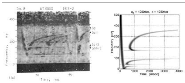
3. ábra Mért (ISIS-2 műhold fedélzetén) és számított elektron- és ionwhistler dinamikus spektruma
