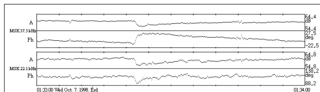
2. ábra Izlandi (37.5 kHz) és skóciai (22.1 kHz) VLF jeladók jelén megjelenő amplitúdó és fázis trimp effektus keskenysávú felvétel egy részletén (Érd)
