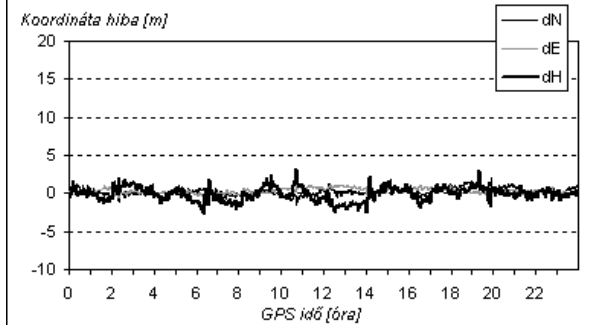
6. ábra Az abszolút helymeghatározás hibája a BME permanens állomáson (mérés: 2002. jún. 16., berni lokális ionoszféra-modell, IGS precíz pályák és órákorrekciók)
