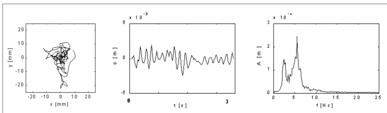
4. ábra A stabilogram (balra) és a gyorsulásmérővel regisztrált esszenciális tremor (középen), melyből kétszeres integrálással és a Fourier spektrum meghatározásával (jobbra) diagnosztizálható a tremor.
