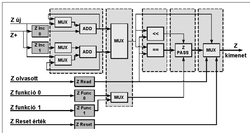
7. ábra Z egység
