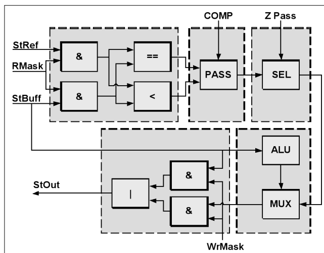
8. ábra Stencil Egység
