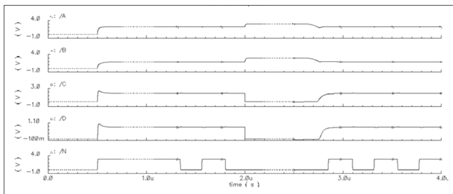
5. ábra Az áramreferencia szimulációja
