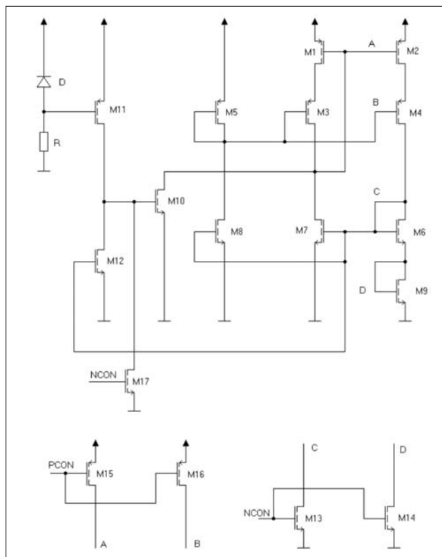
4. ábra A javított áramreferencia
