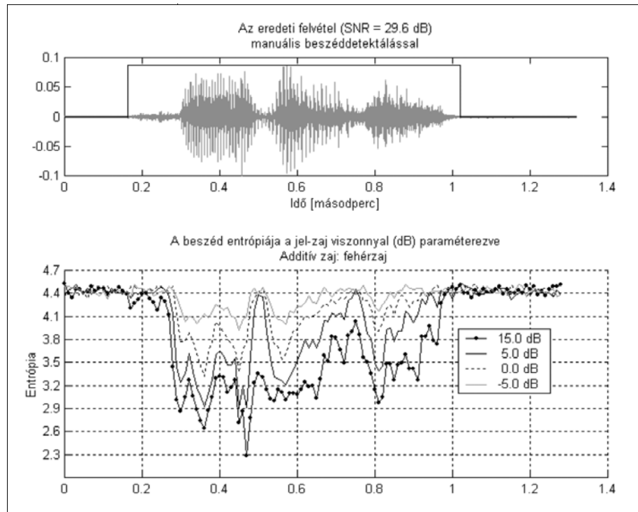
2. ábra Beszédjel entrópiájának alakulása fehérzajban
