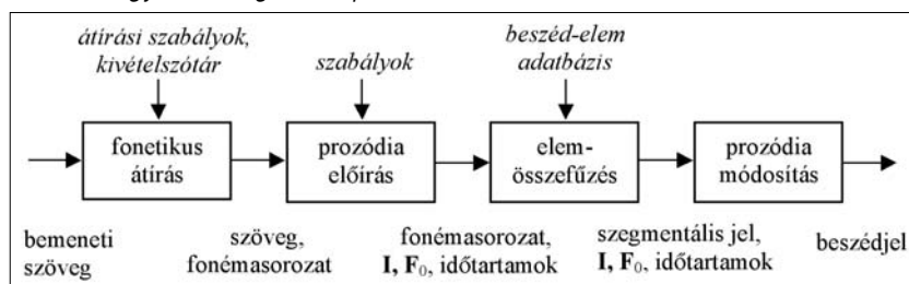
2. ábra Elemösszefűzésen alapuló beszédsszintetizátor egy lehetséges felépítése
