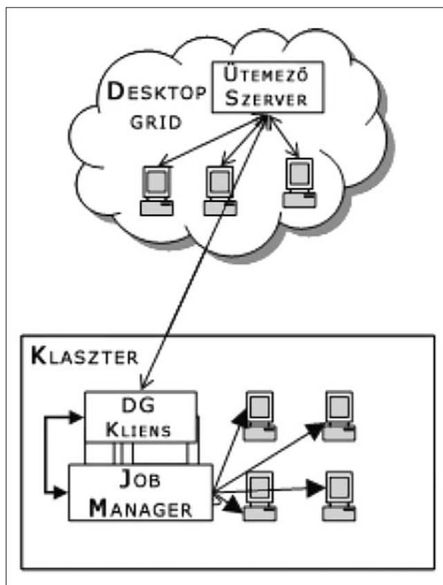
5. ábra Desktopgridhez csatlakozó klaszter
