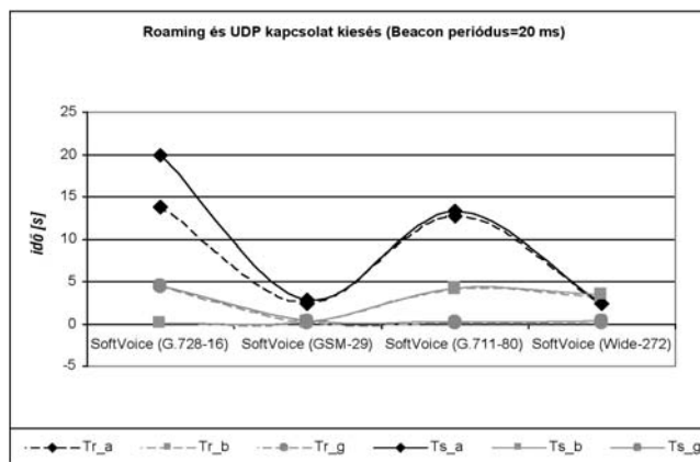
10. ábra Az IP telefon viselkedése ( T_b=20 msec)
