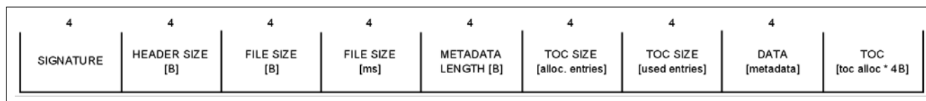
4. ábra Az NSV PDU fejlécének formátuma
