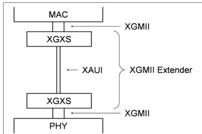
2. ábra XGMII Extender
