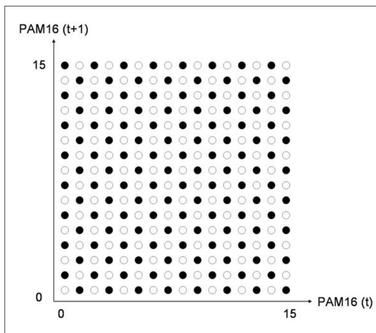
4. ábra DSQ128 konstelláció
