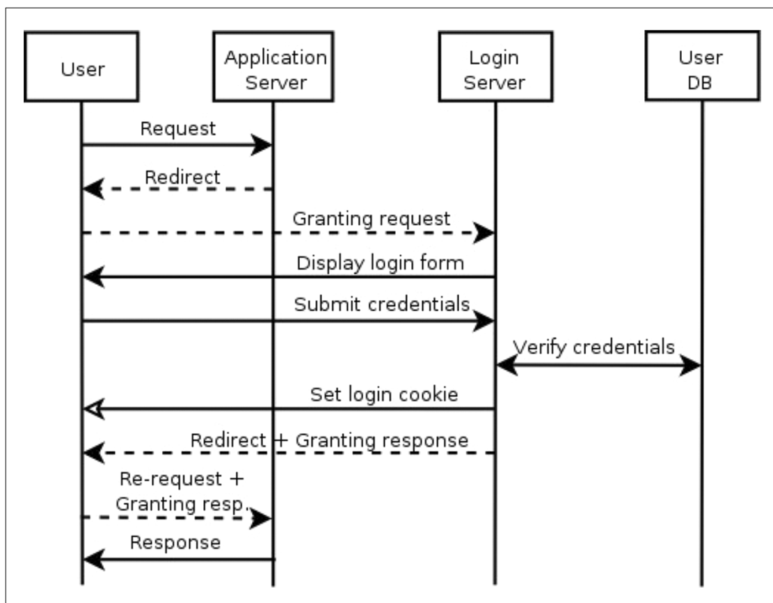
1. ábra Webes SSO alkalmazás (PubCookie) működésének folyamata [2]
