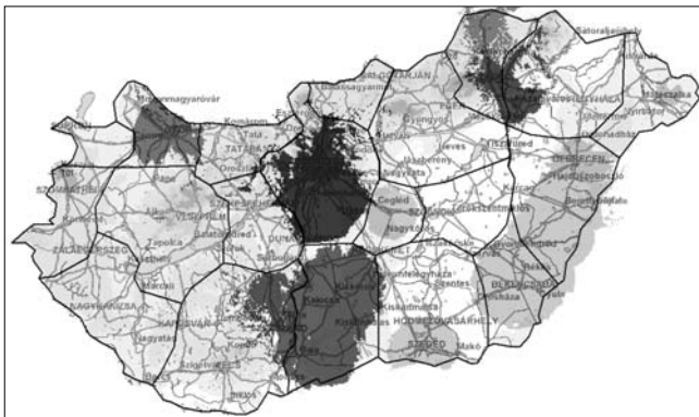
5. ábra Hordozható kültéri vétel L=70% (megfelelő vétel), Emed=79.3 dBμV/m
