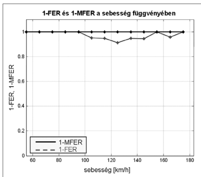
16. ábra Mobil Doppler mérés: 2k, 64-QAM, CR=2/3, MPE-FEC=3/4
