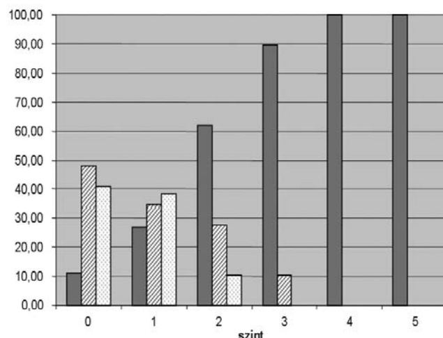
21. ábra 2k, QPSK, CR=1/2, MPE-FEC=3/4
