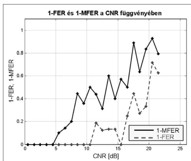
10. ábra Mérés eredmények: külváros, 2k, 64-QAM, CR=2/3, MPE-FEC=3/4
