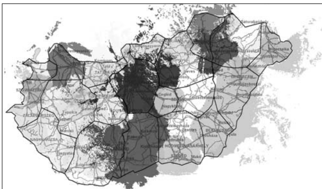
7. ábra Mobil vétel, külső antennához csatlakoztatva L=90% (megfelelő vétel), Emed=62.5 dBμV/m
