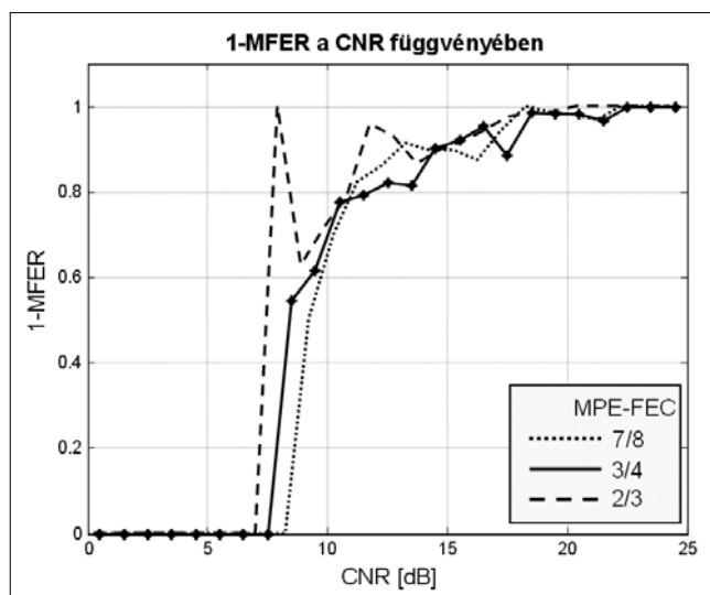
8. ábra Az MPE-FEC hatásának szemléltetése 8k, 16-QAM, CR=2/3 esetén
