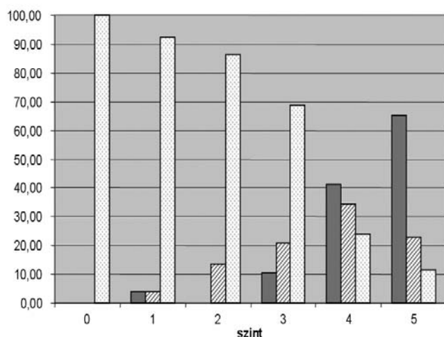
20. ábra 8k, 64-QAM, CR=2/3, MPE-FEC=3/4
