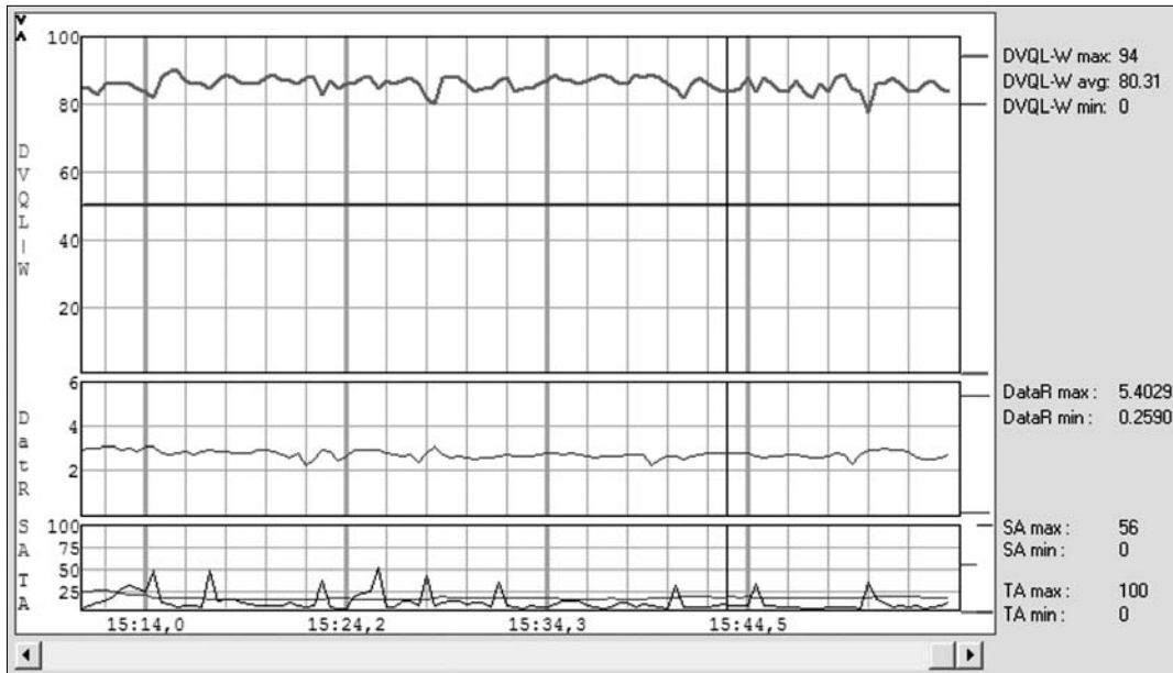
17. ábra A Rohde&Schwarz DVQ műszere által rögzített objektív képmínőség- vizsgálat adatai
