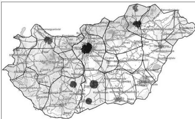
6. ábra Hordozható beltéri vétel L=70% (megfelelő vétel), Emed=91.7 dBμV/m
